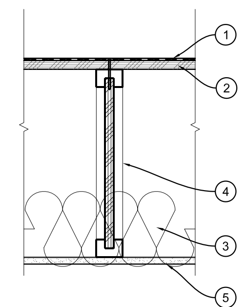
D2 ROOF DECK
