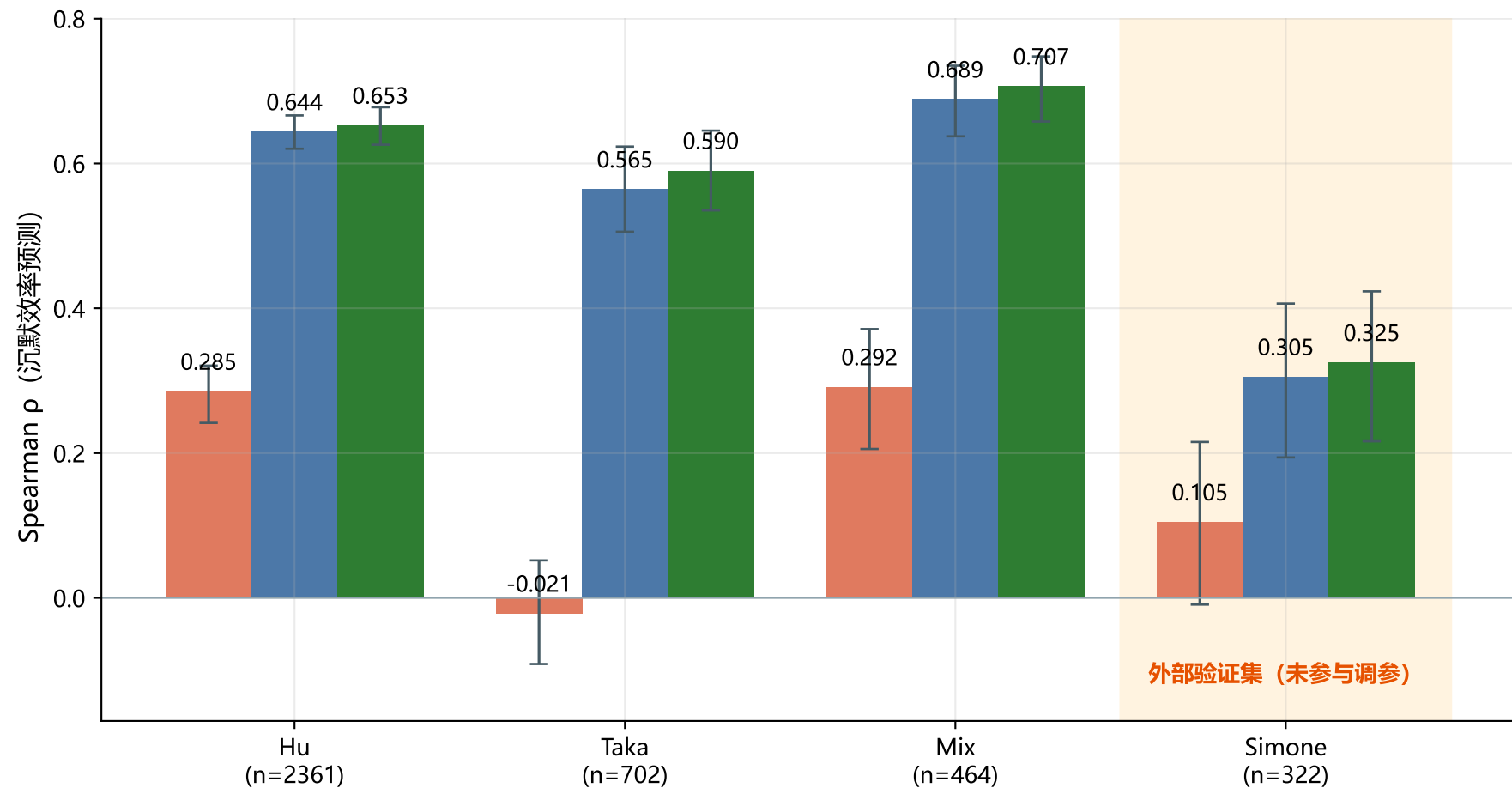
四套公开数据集：组合分均高于单用热力学或单用深度学习 (含 95% CI) 组合分 \alpha 0.4/\beta 0.6
