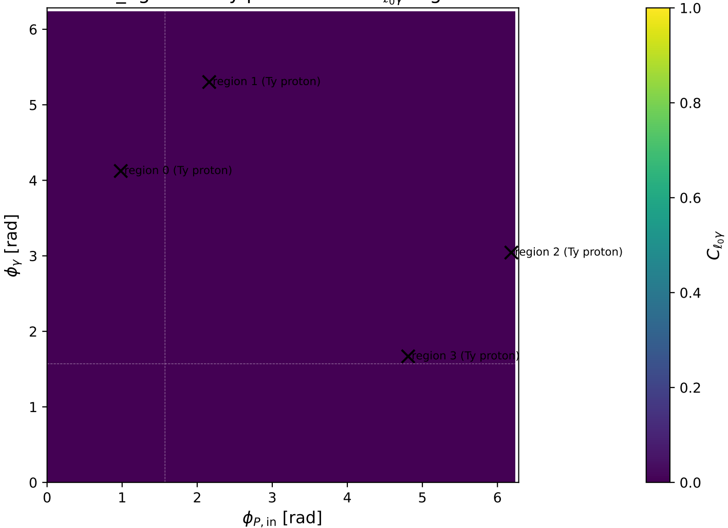
low_Egamma Ty proton: max C_{\ell_0\gamma} regions
