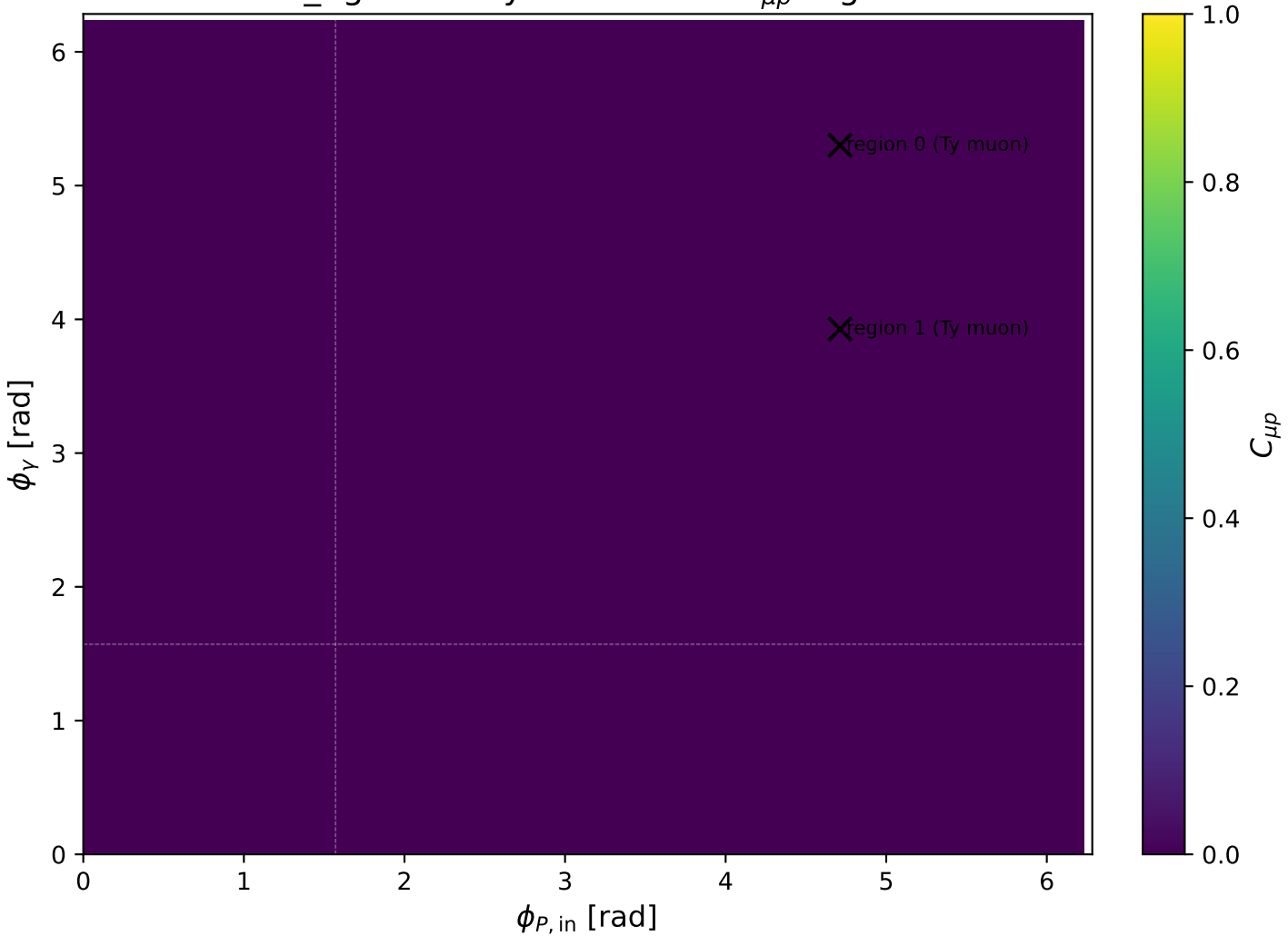
low_Egamma Ty muon: max C_{\mu p} regions
