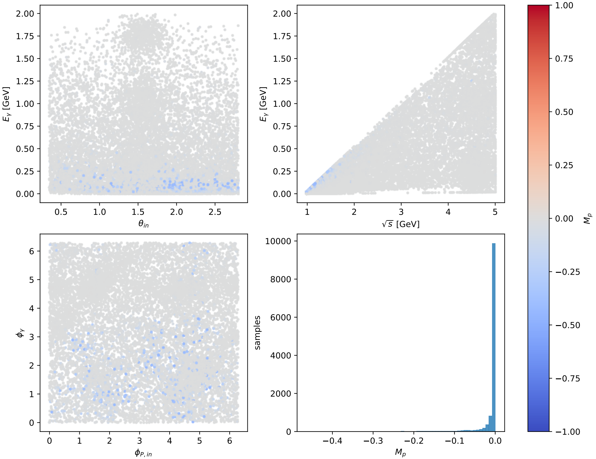
Phase-space scan: L proton [L_proton], max M_p=1.1813\text{e-13}
