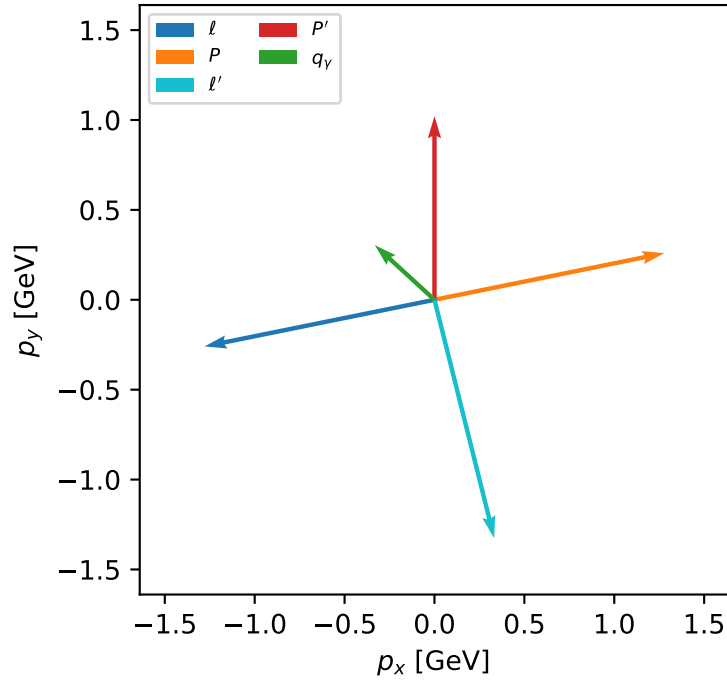
Transverse momenta
