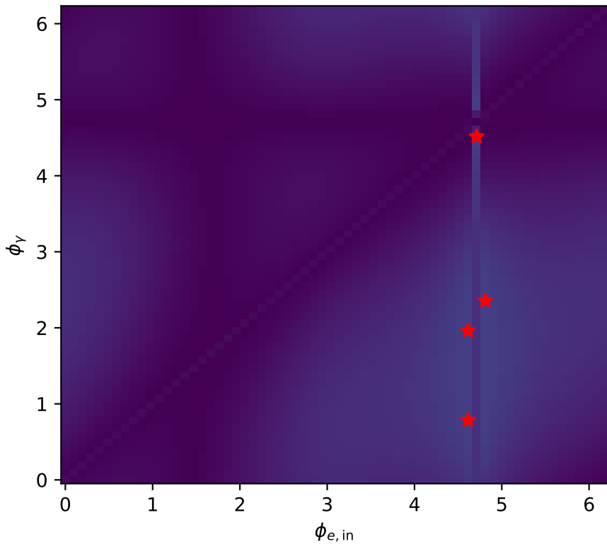
low_Egamma
