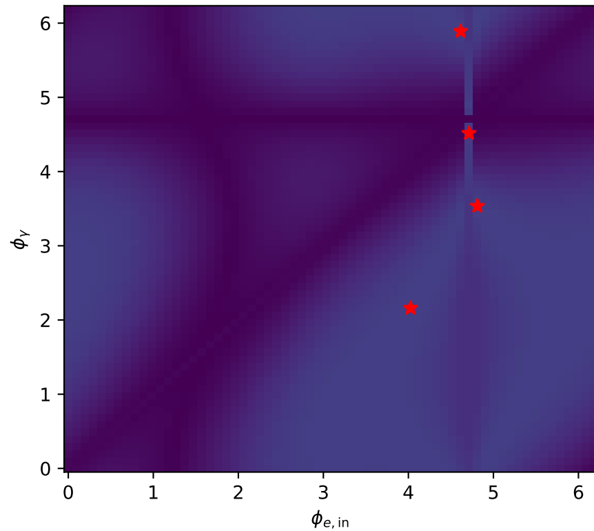
mid_Egamma
