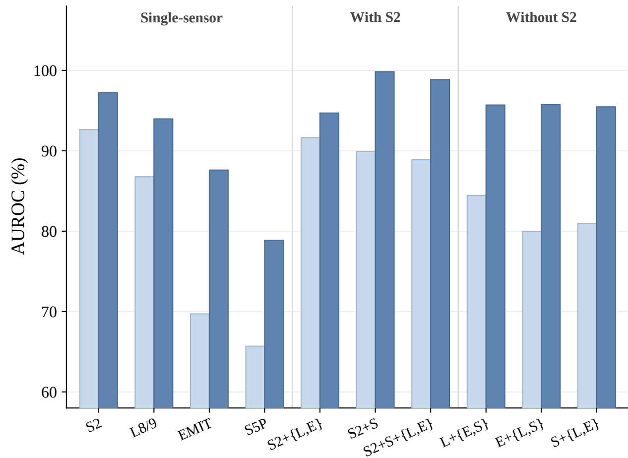
AUROC
