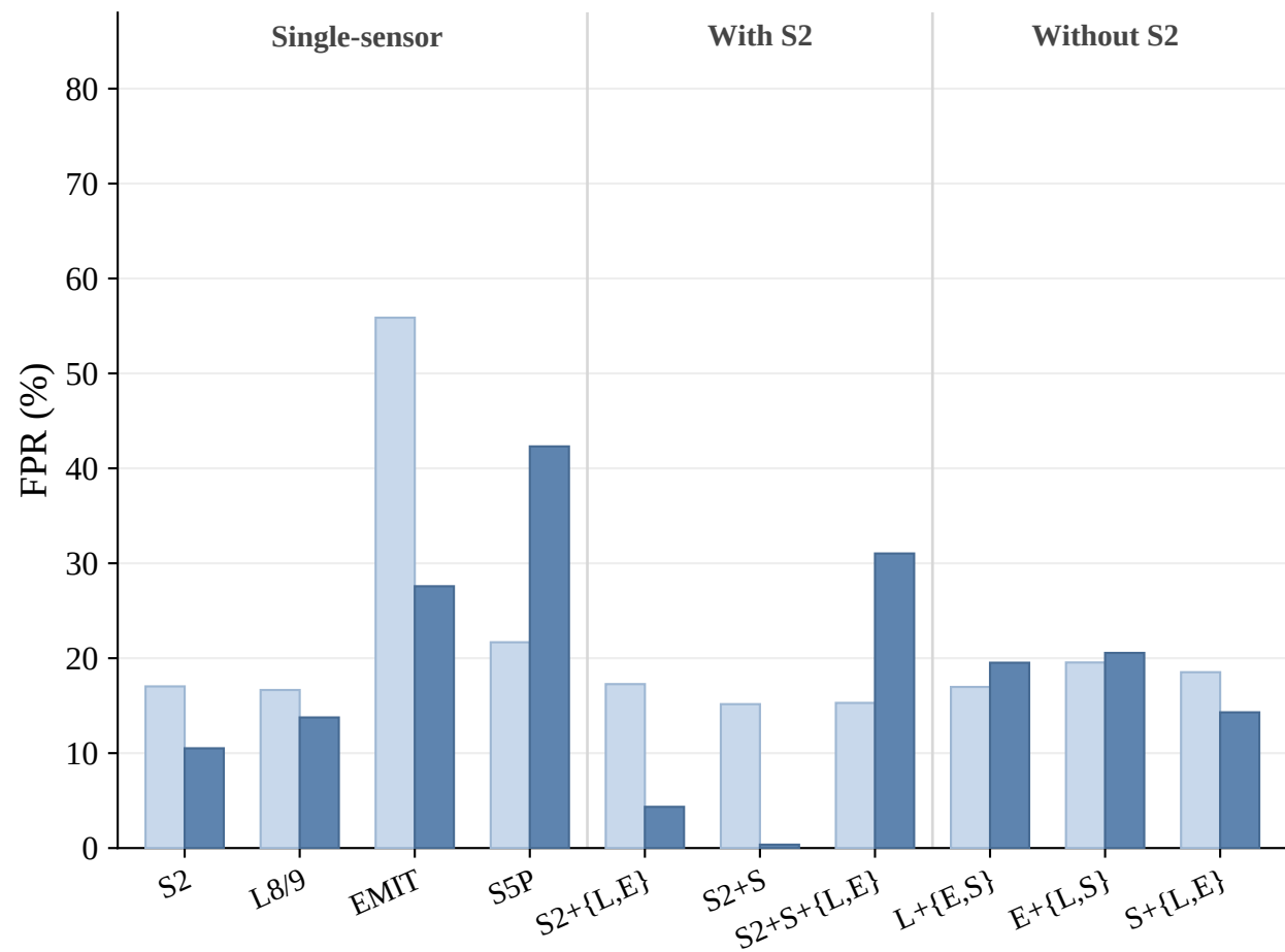
FPR
