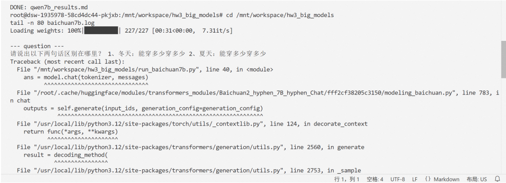
图 6 Baichuan2-7B 兼容性错误日志截图
