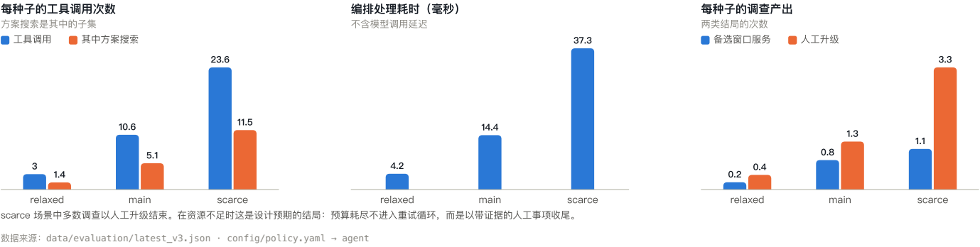
图 24-3 Agent 调查的成本与产出随资源稀缺度的变化。
