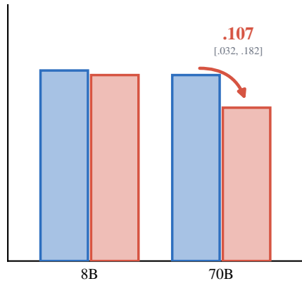
Llama (R1-distill)
