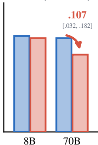
Llama (R1-distill)
