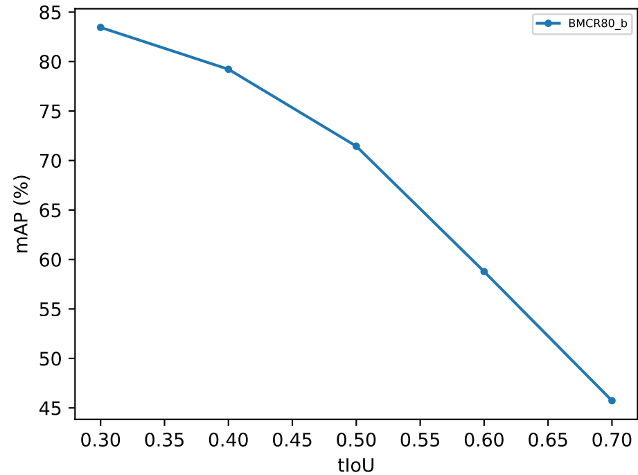
VideoMAE-B
