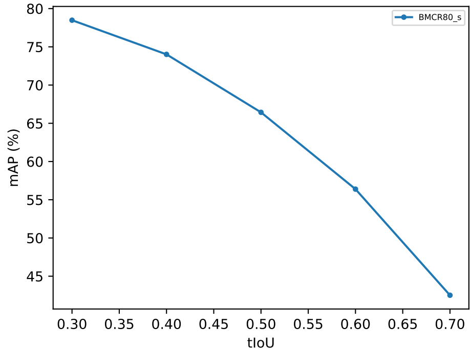
VideoMAE-S
