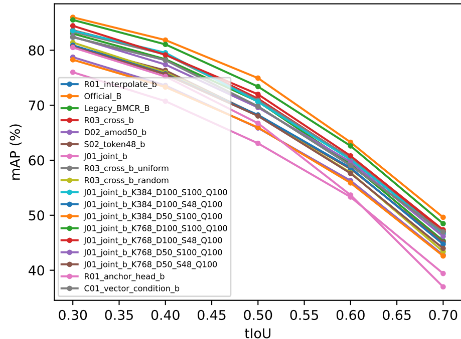
VideoMAE-B
