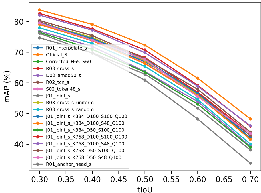
VideoMAE-S
