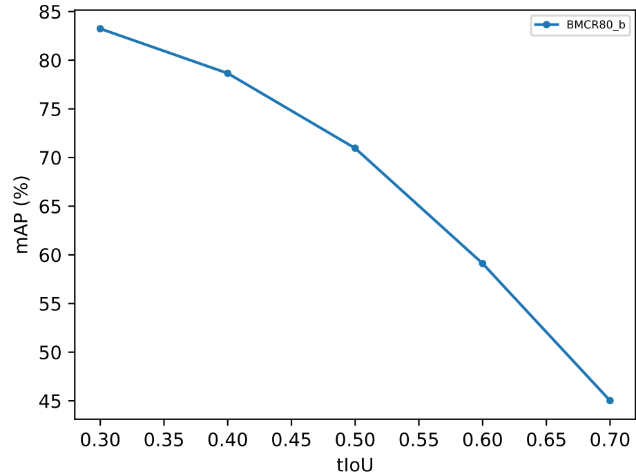
VideoMAE-B
