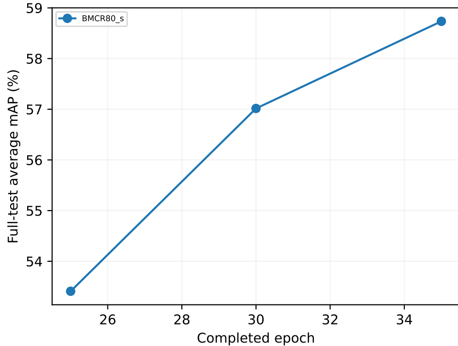
VideoMAE-S
