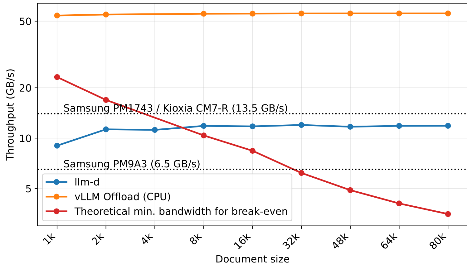
KV Cache Break-Even Bandwidth (Llama 3.2 3B)
