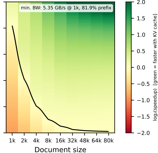
vLLM Offload (CPU)
