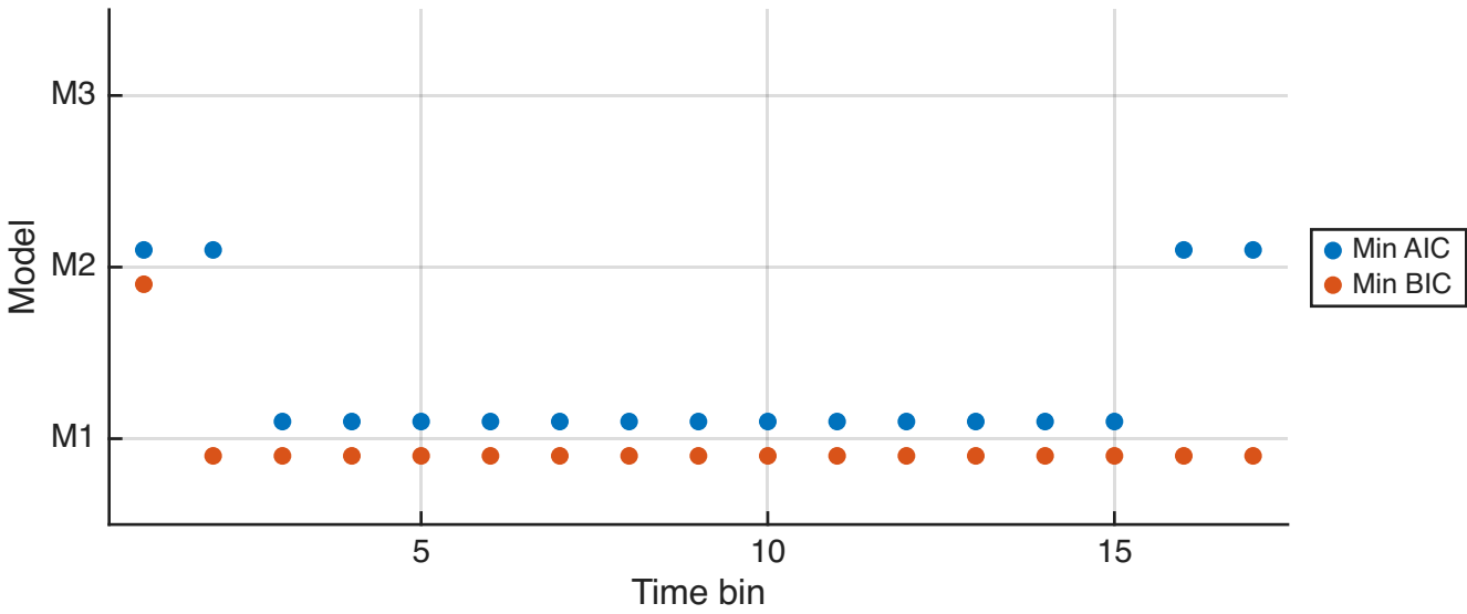
vol3abs - incorr - all n = 404
