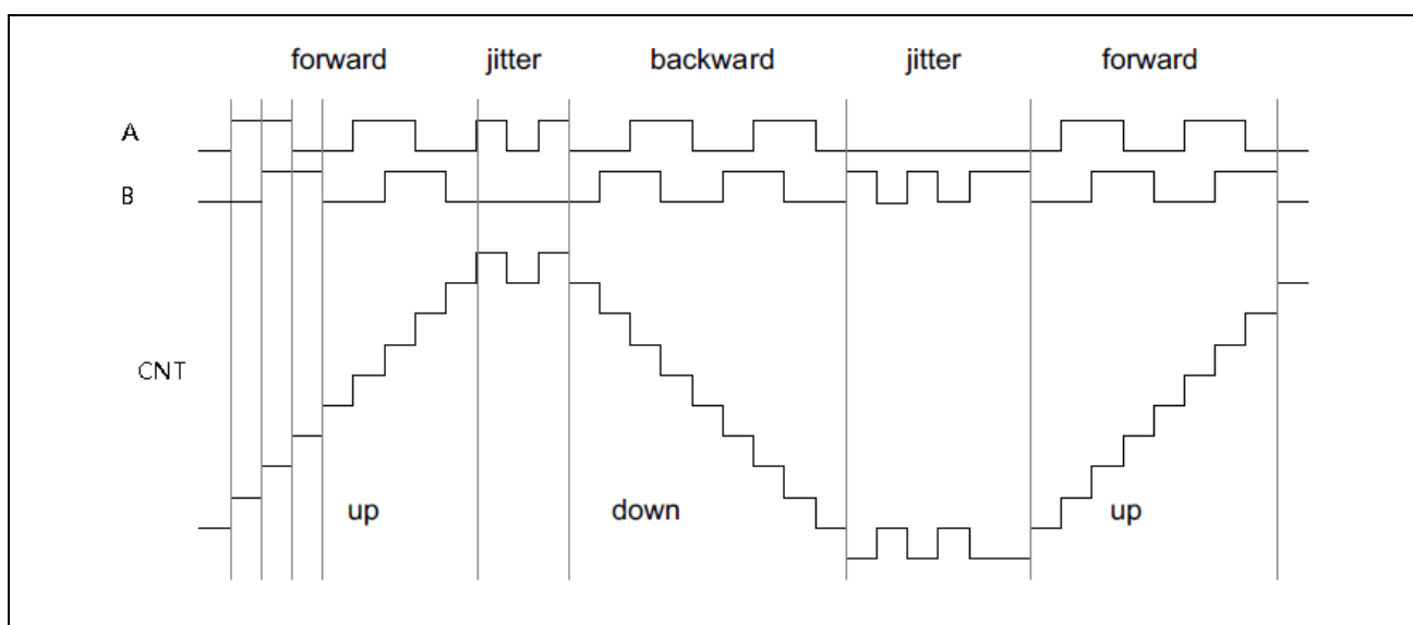
图 14-54 编码计数
