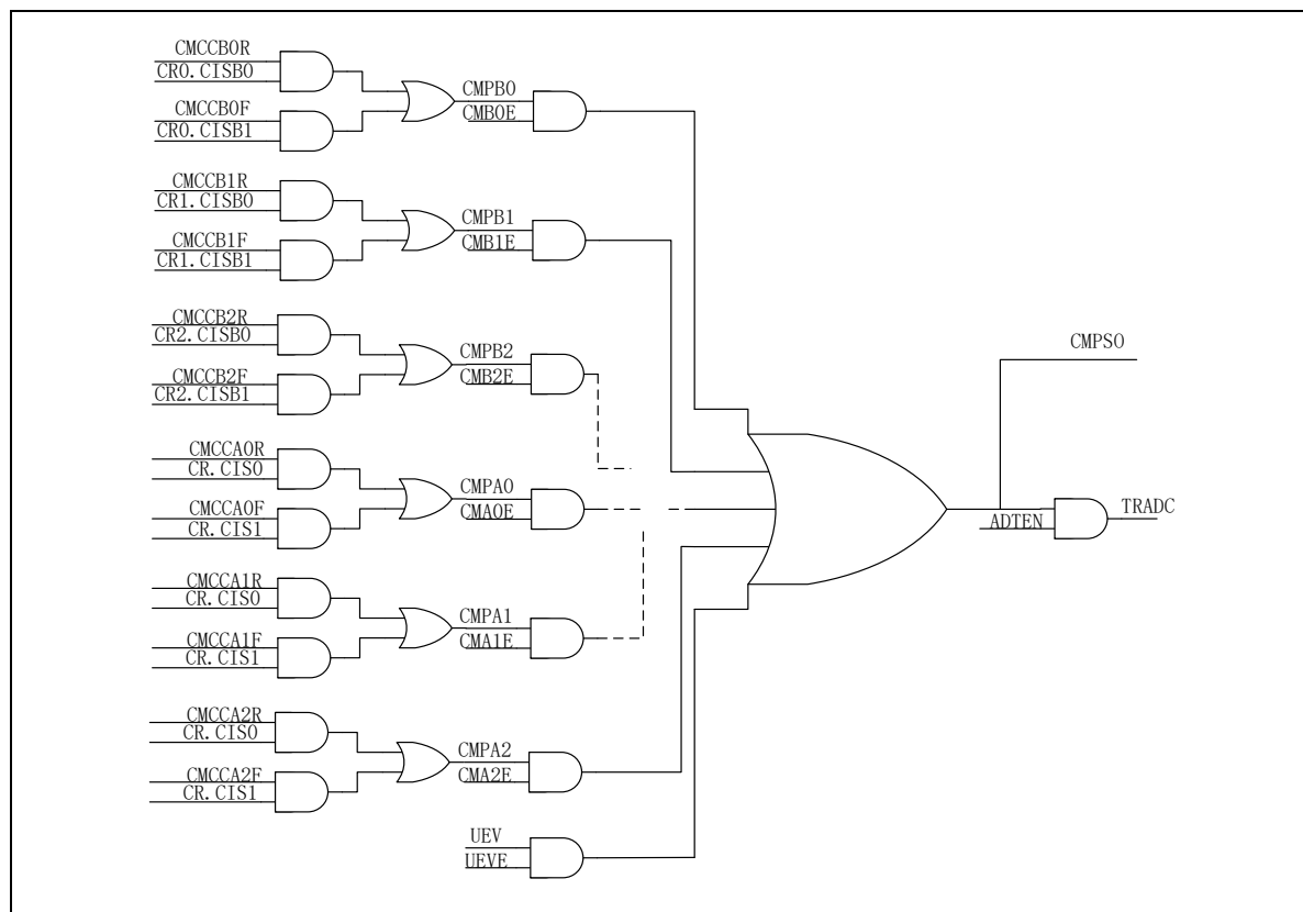
图 14-55 ADC 触发
