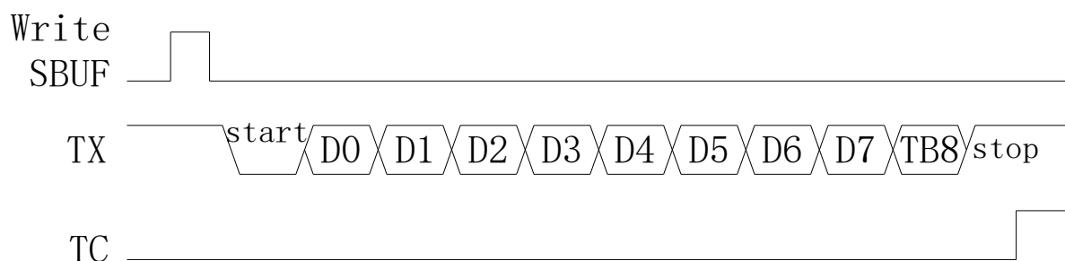
图 18-8 Mode3 发送数据
