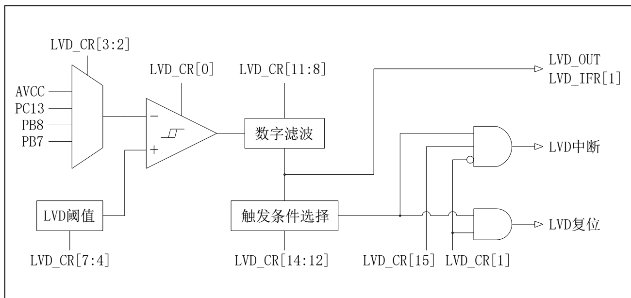
图 24-1 LVD 框图
