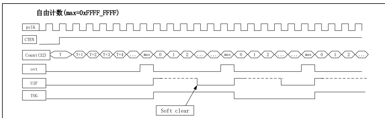
图 14-7 自由计数时序图
