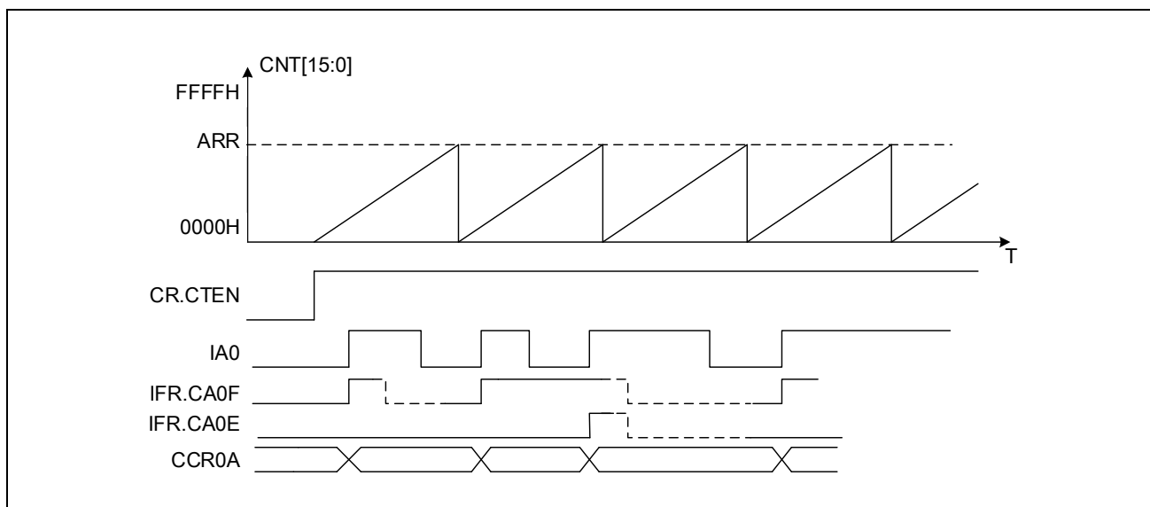
图 14-48 捕获时序图
