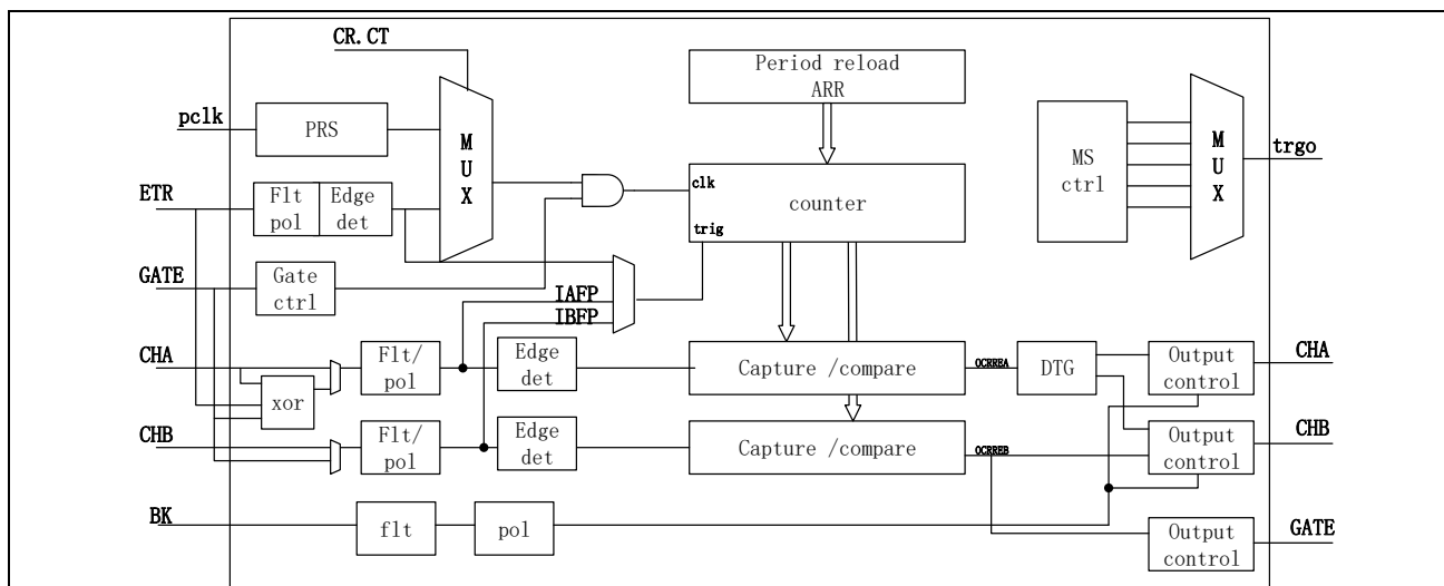
图 14-1 TIM0/1/2 框图
