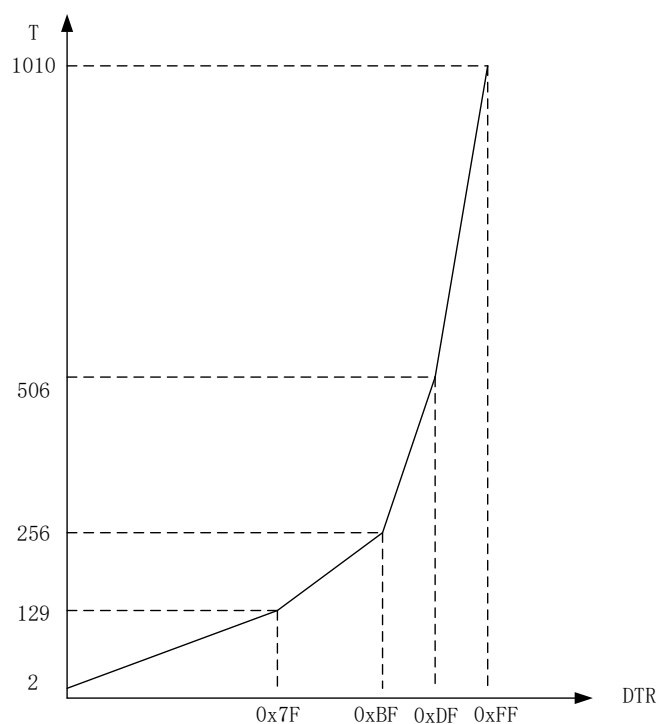
图 14-42 死区时间
