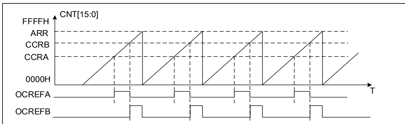
图 14-34 锯齿波计数双点比较 OCREF 输出 (OCMx=111)
