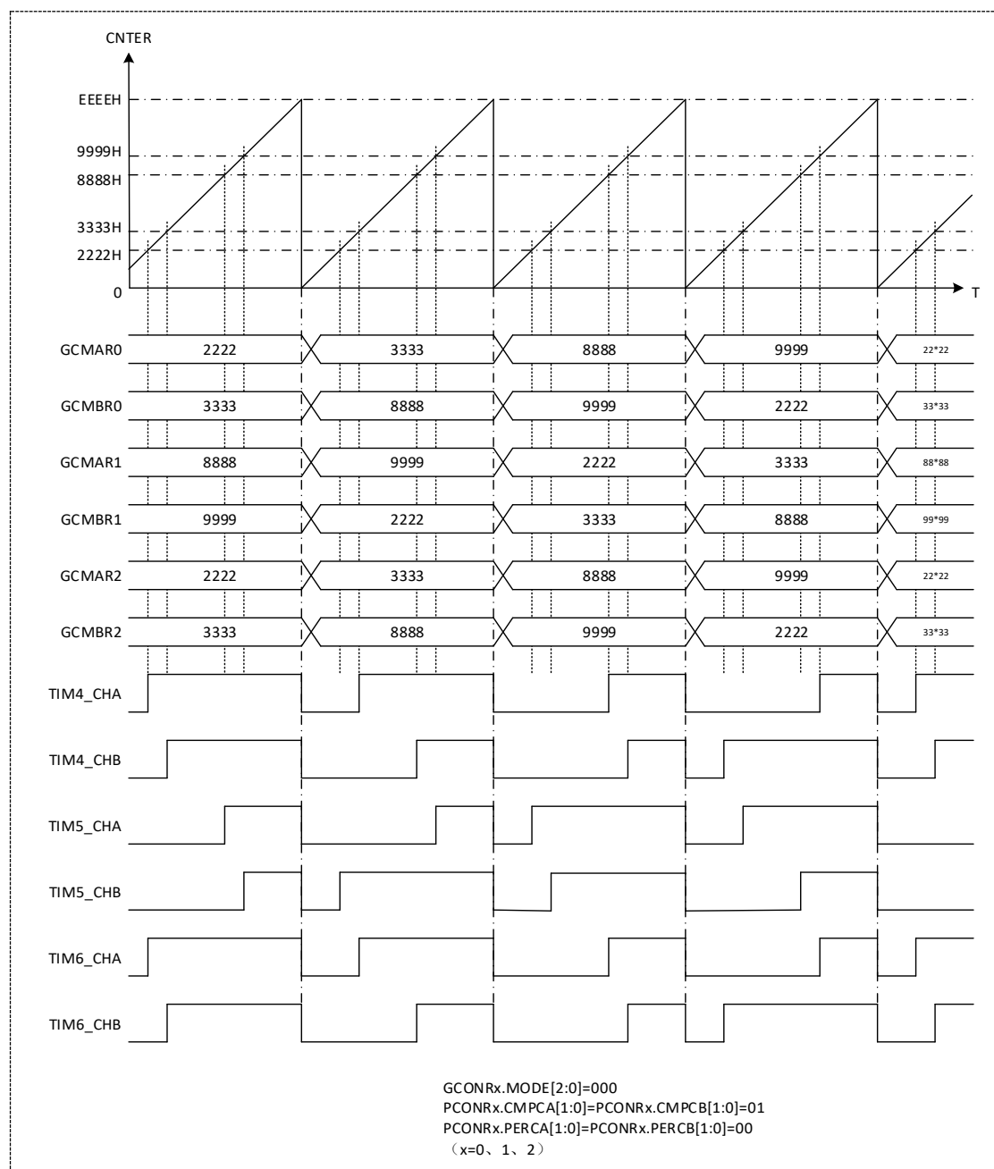
图 16-14 6 相 PWM 波
