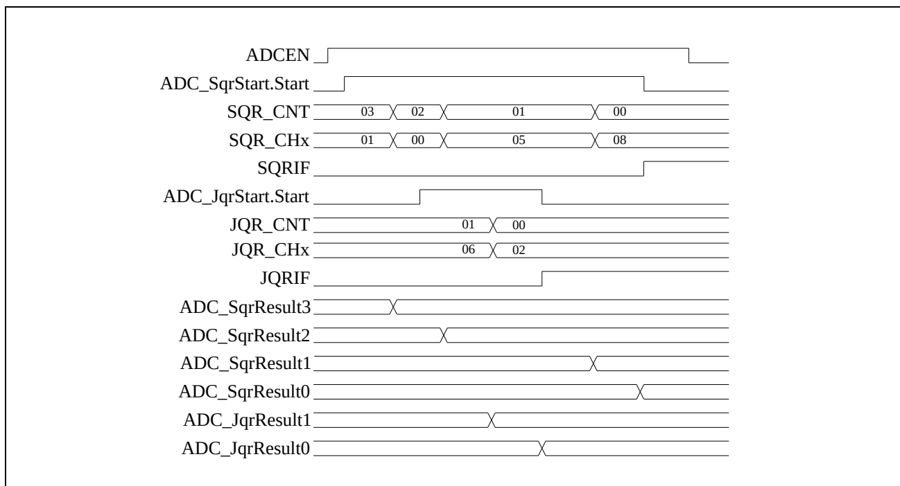
图 22-5 ADC 顺序扫描过程中进行插队扫描示例
