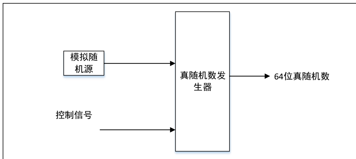
图 20-1 TRNG 数据流
