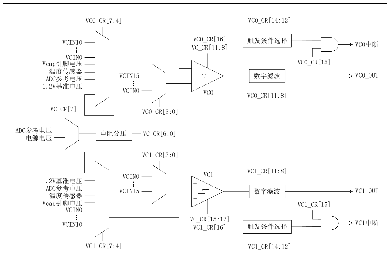
图 23-1 VC 框架图
