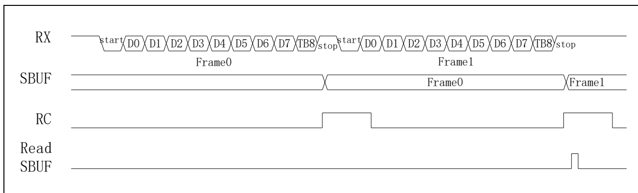
图 18-13 接收缓存
