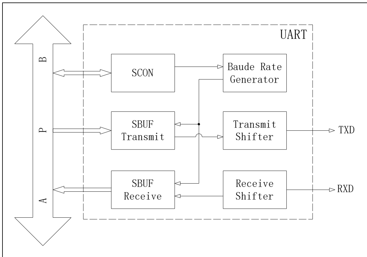
图 18-1 结构框图
