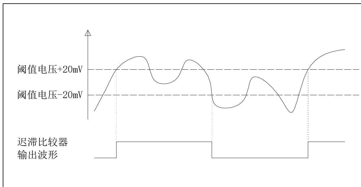
图 24-3 LVD 迟滞响应
