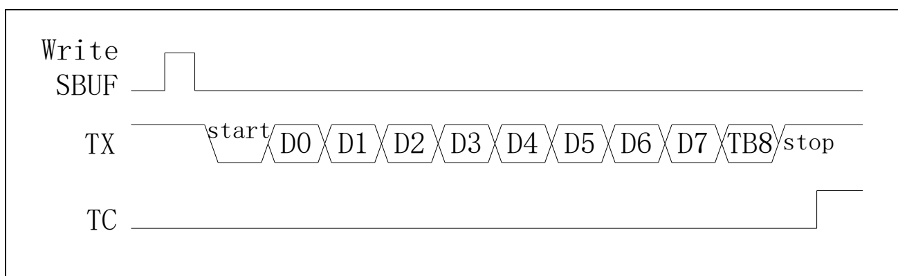
图 18-6 Mode2 发送数据
