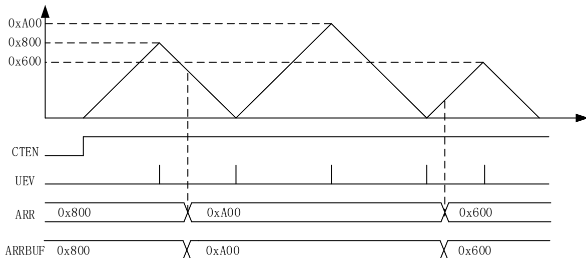
图 14-25 角波模式下缓存无效
