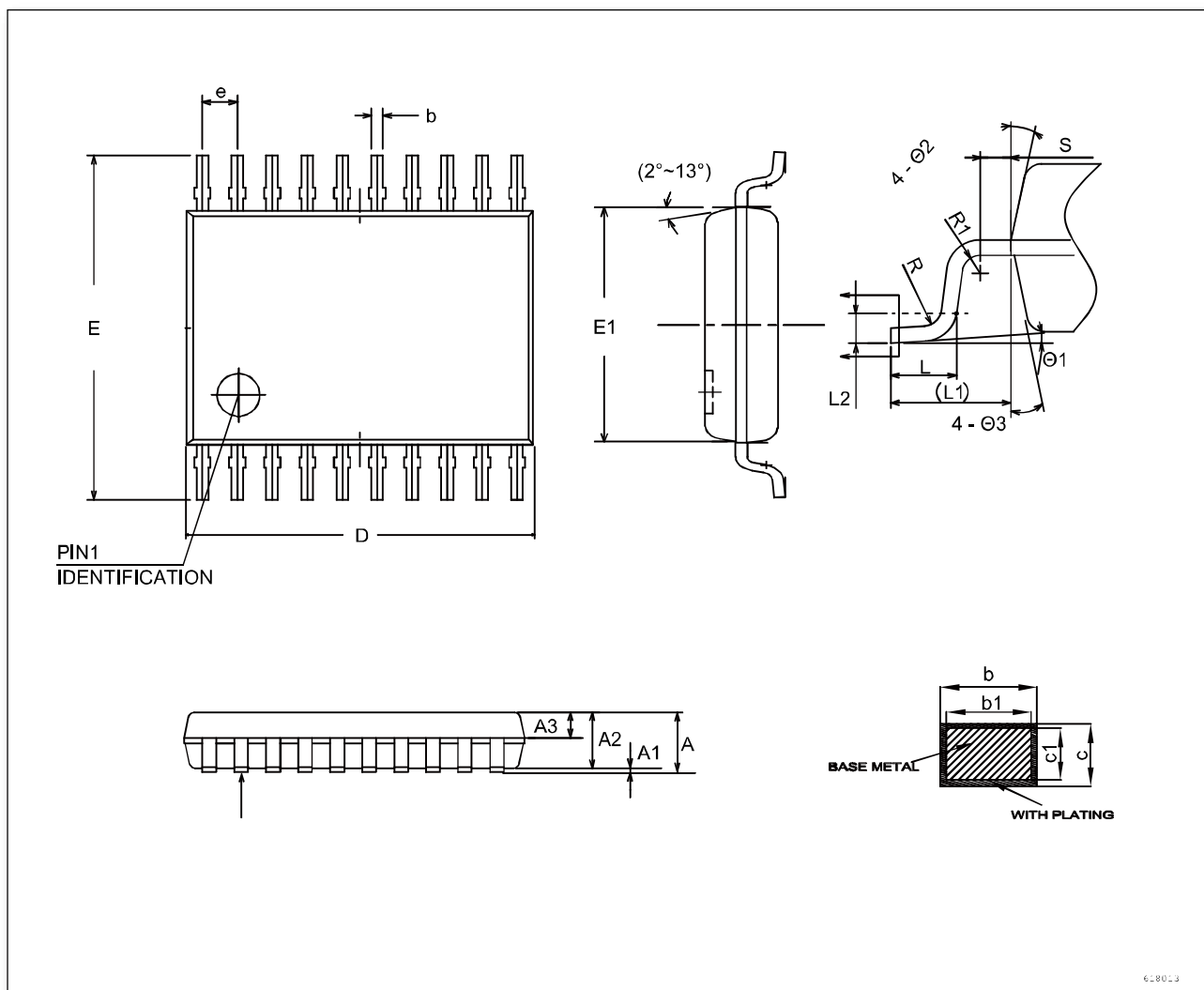
图 6-2 TSSOP20 封装尺寸
