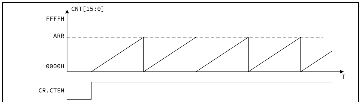
图 13-21 边沿对齐计时器波形 ( DIR =0)
