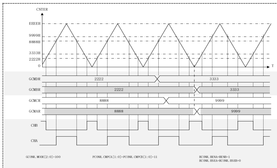
图 15-12 三角波 A 模式时软件设定 GCMBR 互补 PWM 波输出
