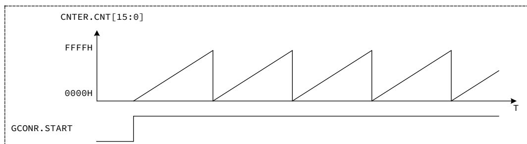
图 15-2 锯齿波波形（递加计数）
