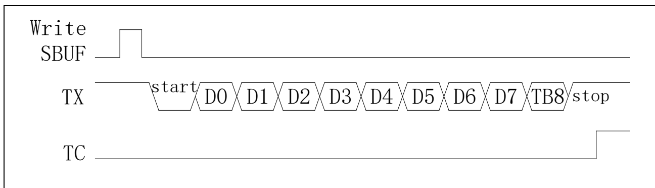
图 17-6 Mode2 发送数据
