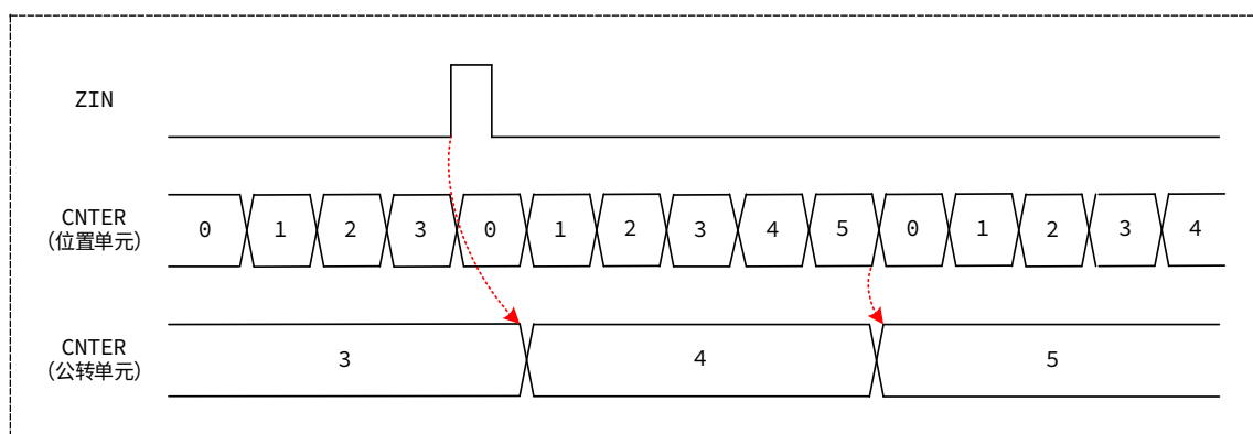
图 15-23 公转模式时 Z 相计数和位置计数器输出混合计数动作
