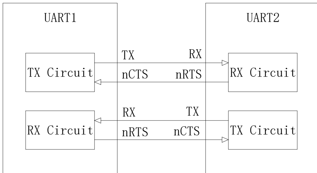
图 17-10 UART 硬件流控
