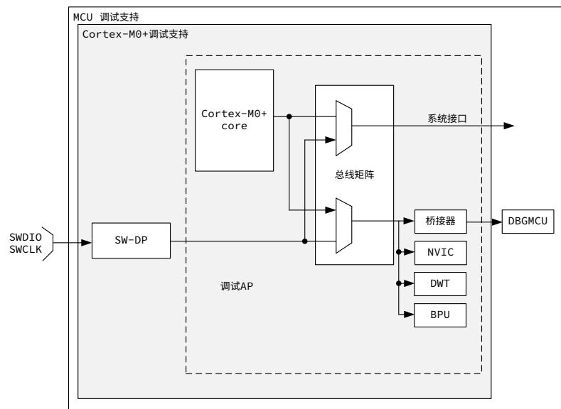
图 28-1 调试支持框图
