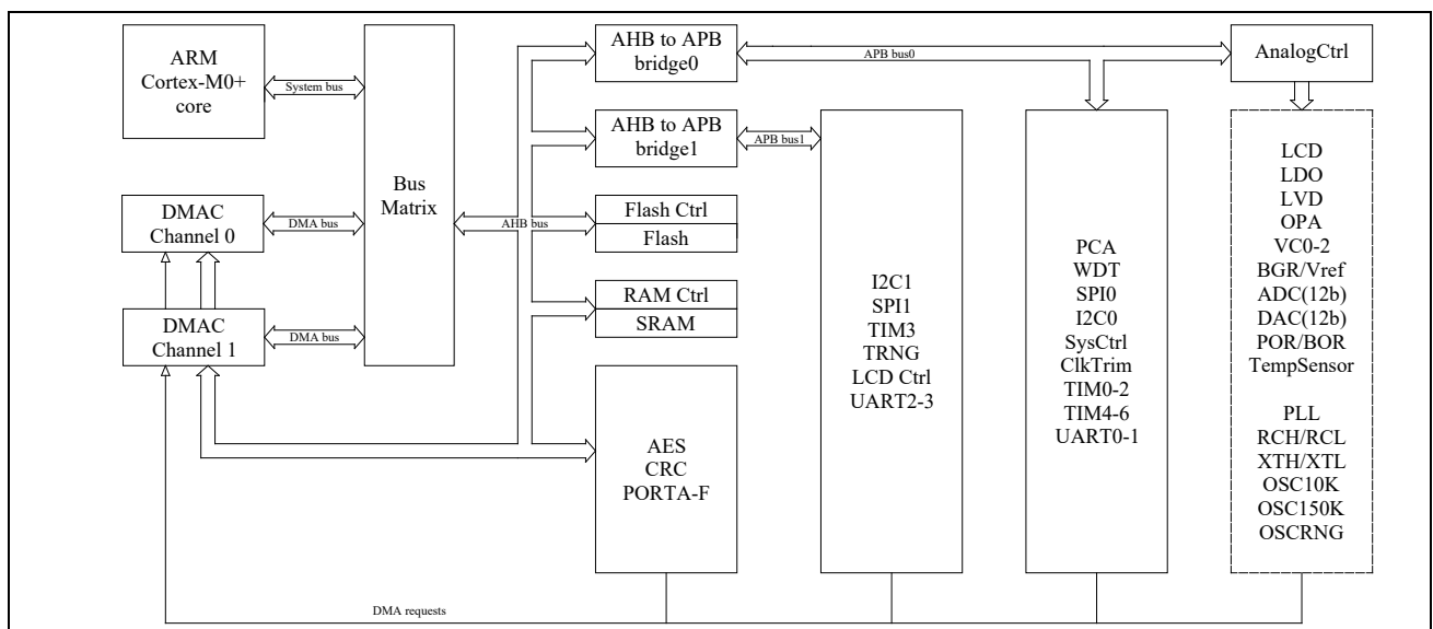
图 1-1 系统架构示意图
