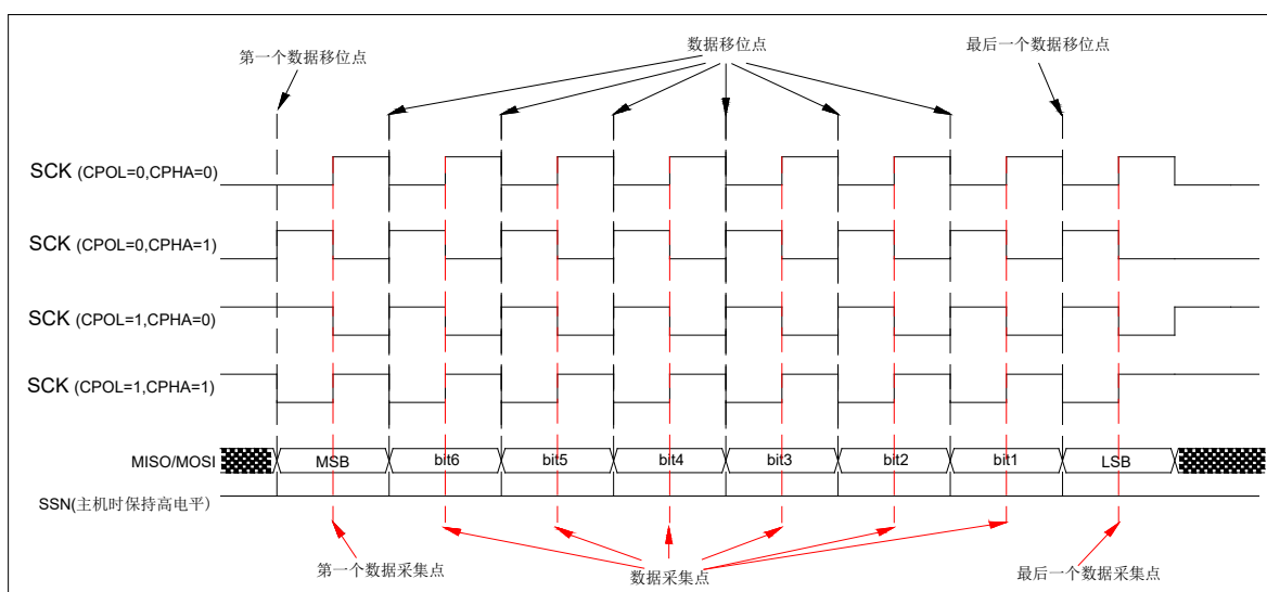
图 8-3 主机模式帧格式
