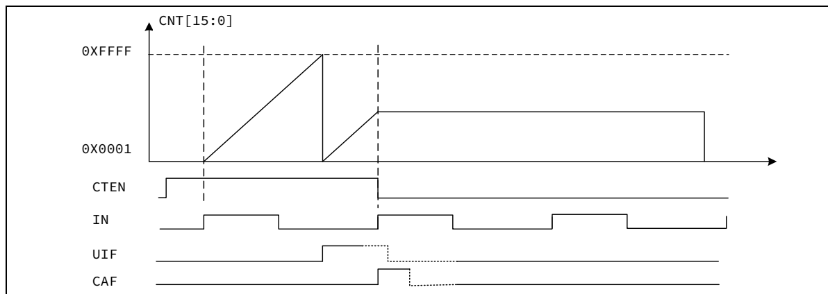
图 13-13 上升沿到上升沿周期测量单次模式
