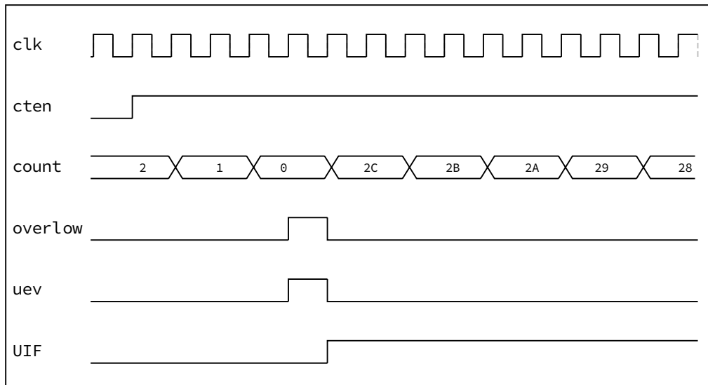
图 13-18 带预分频的下计数
