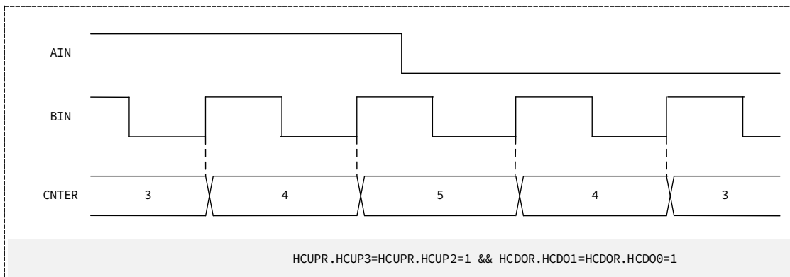
图 15-20 位置模式时方向计数动作
