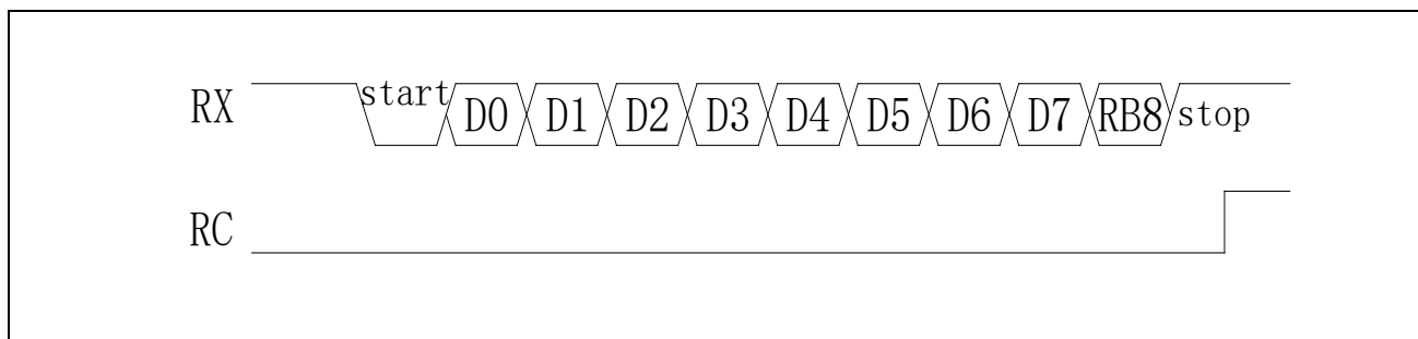
图 17-9 Mode3 接收数据
