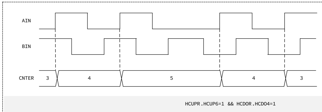
图 15-17 位置模式时相位差计数动作设定 (1 倍)
