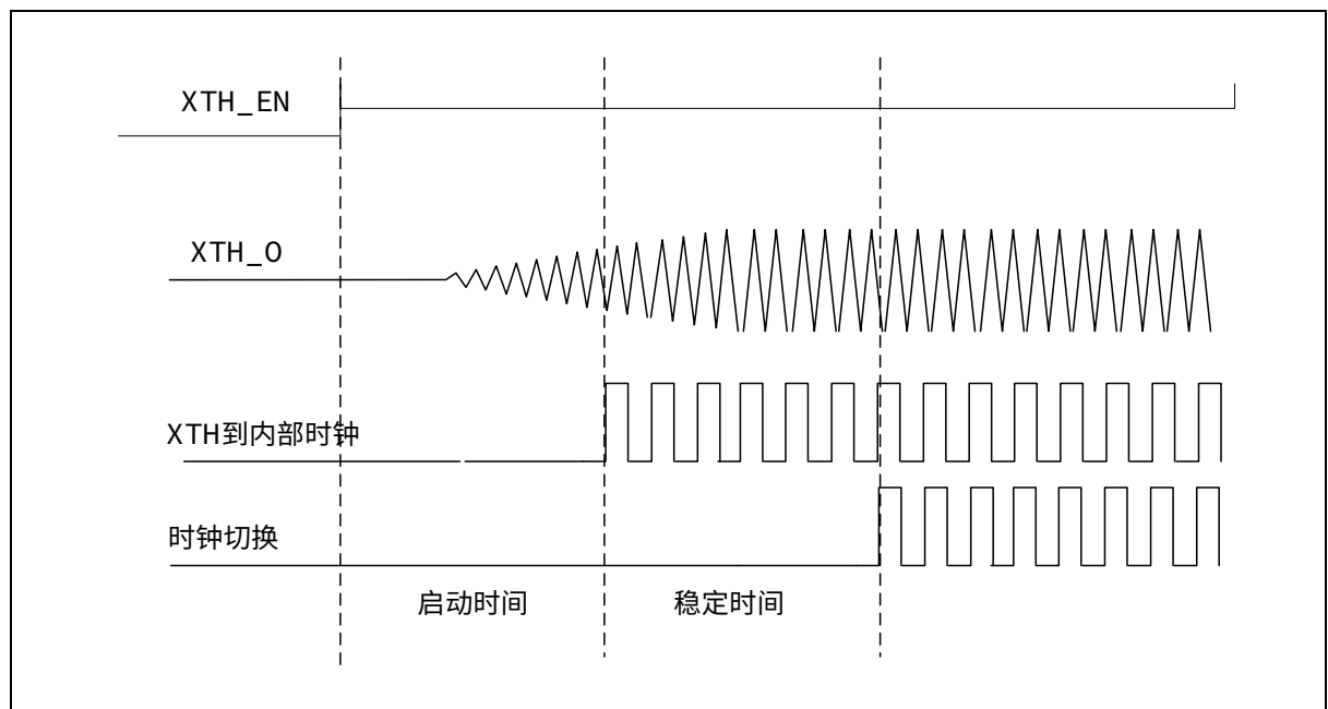
图 3-2 晶振时钟启动示意图
