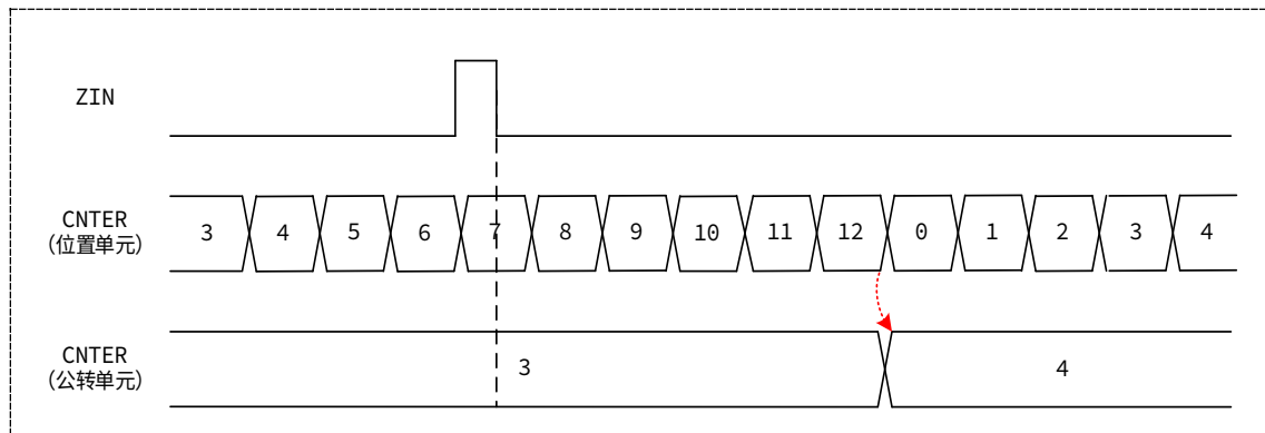
图 15-22 公转模式时位置计数器输出计数动作
