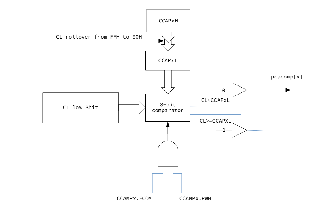
图 14-7 PCA PWM 功能框图
