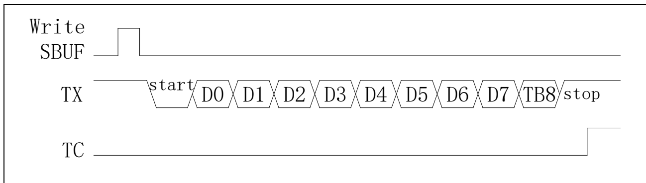
图 17-8 Mode3 发送数据
