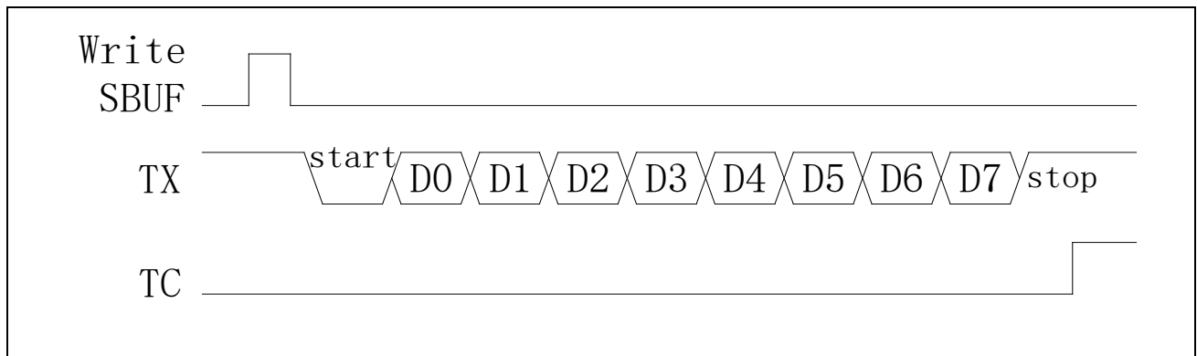
图 17-4 Mode1 发送数据
