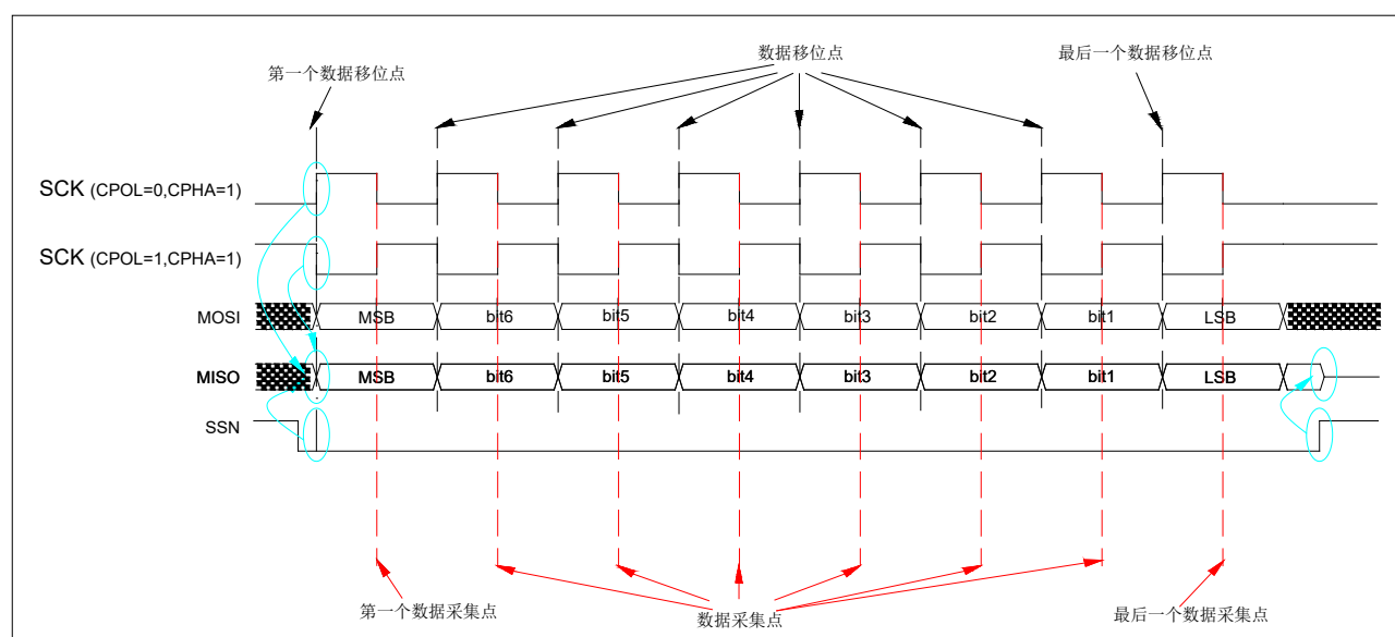
图 8-5 从机 CPHA 为 1 时数据帧格式
