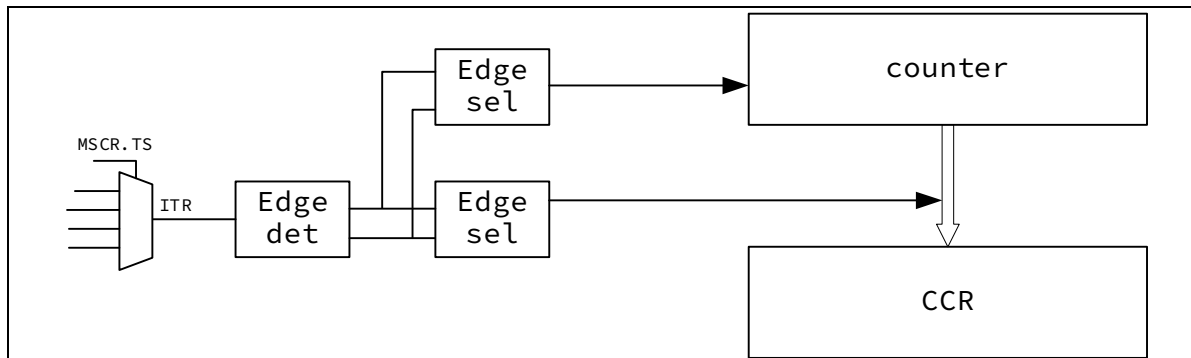
图 13-9 PWC 测量框图
