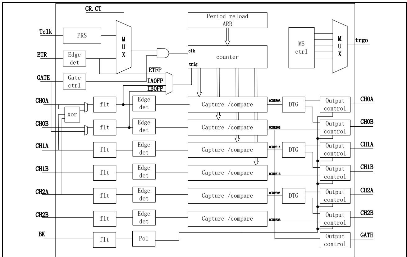
图 13-2 TIM3 框图
