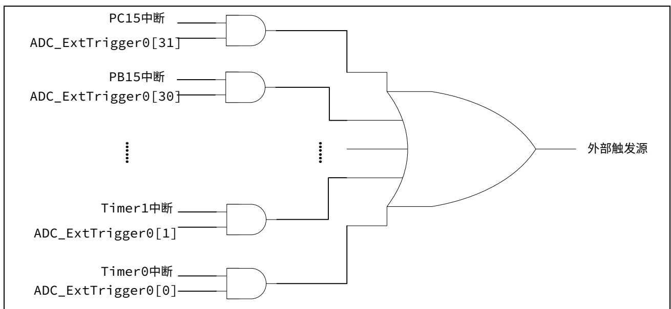
图 22-7 ADC 单次转换或顺序扫描转换外部触发源示意图
