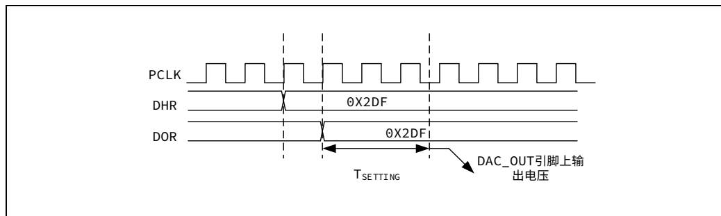
图 23-1 触发不使能时 DAC 转换时序图
