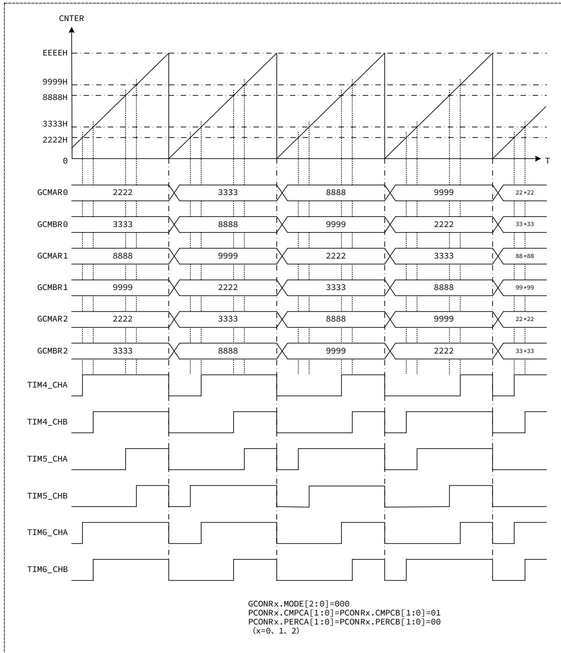
图 15-14 6 相 PWM 波
