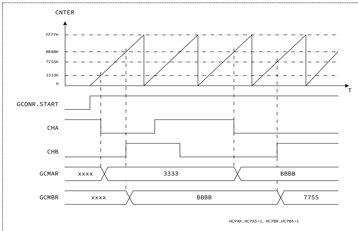
图 15-5 捕获输入动作
