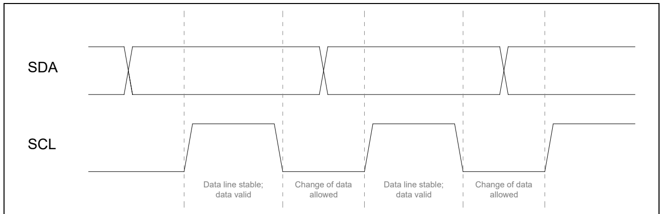
图 7-3 I2C 总线上位传输
