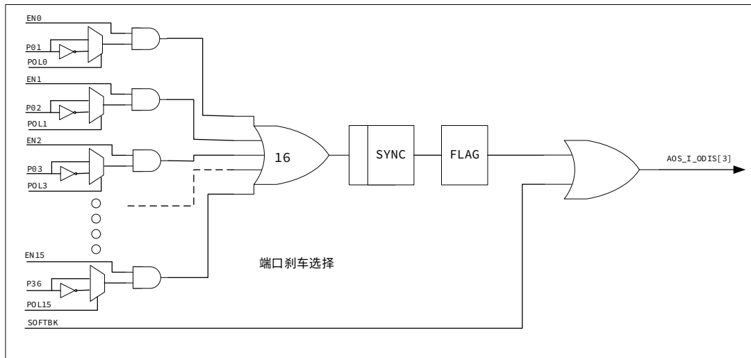
图 15-27 端口刹车与软件刹车示意图
