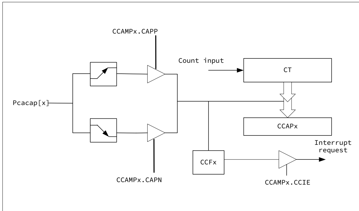
图 14-3 PCA 捕获功能框图
