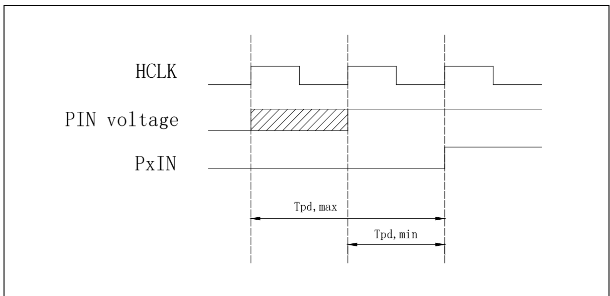
图 6-3 读取端口引脚数据同步图
