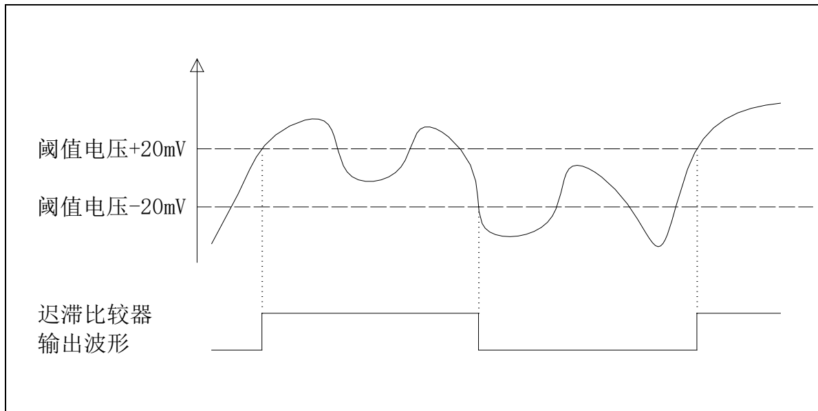
图 25-2 LVD 迟滞响应
