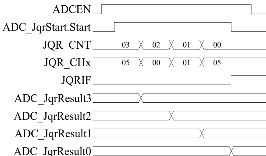
图 22-4 ADC 插队扫描转换过程示例
