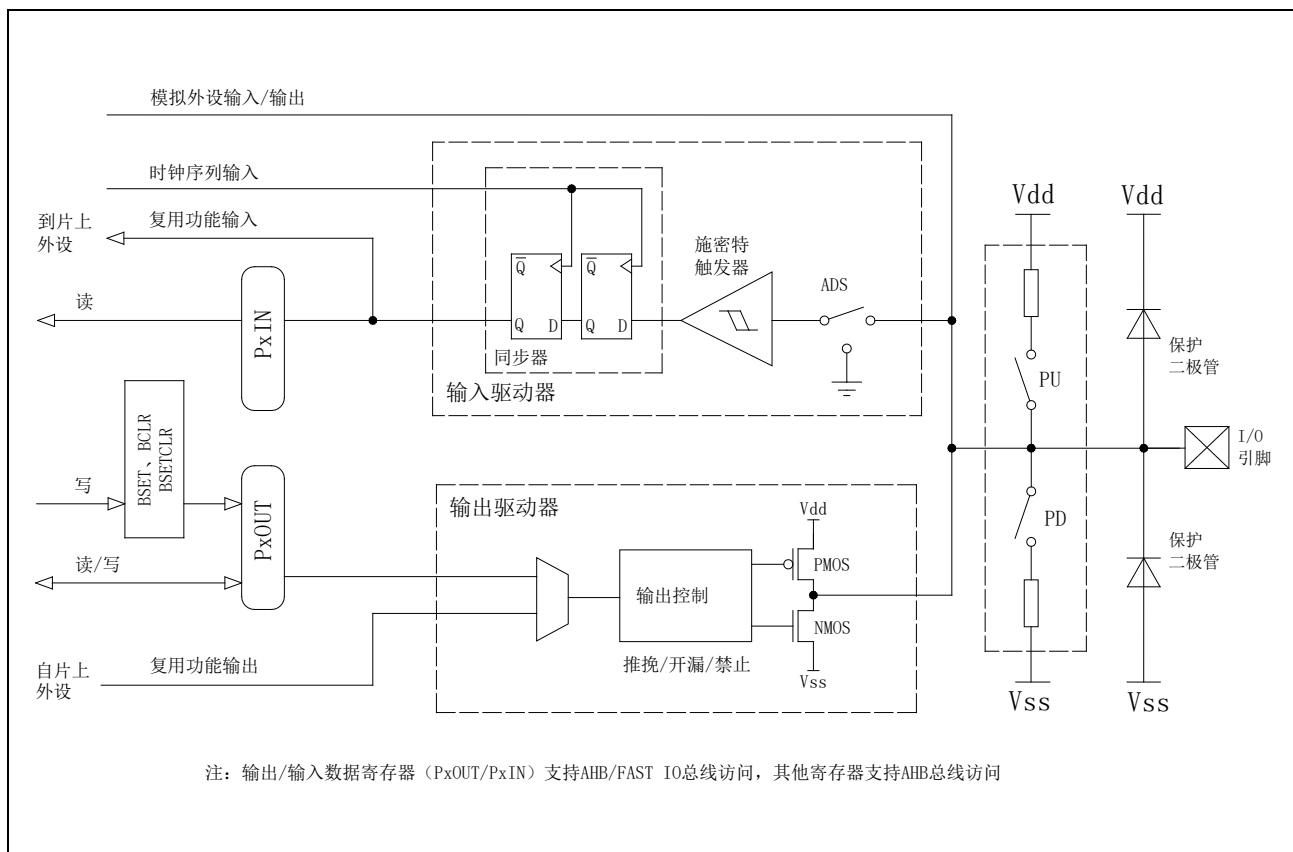
图 6-1 端口电路图
