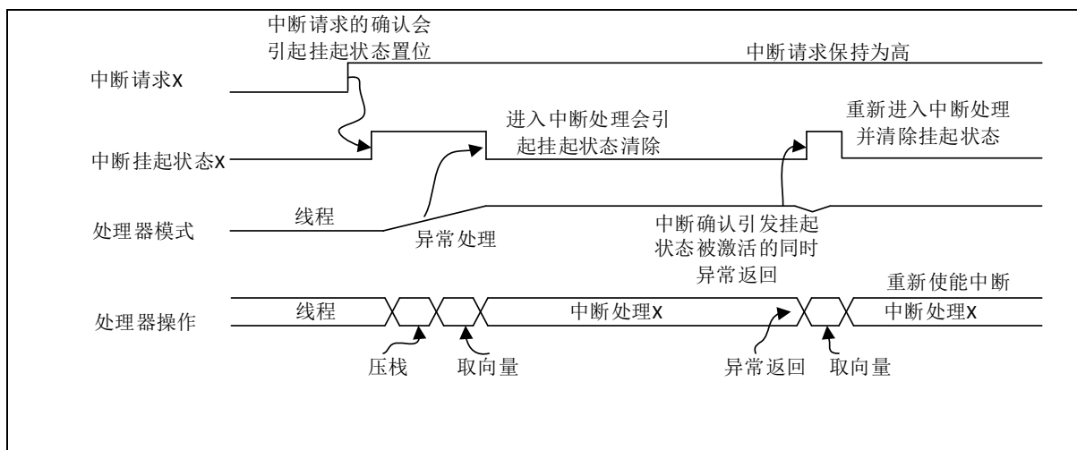
图 5-5 中断退出时若中断请求保持高电平就会引起中断处理的再次执行
