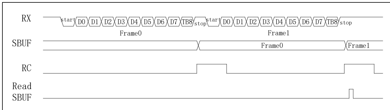
图 17-13 接收缓存
