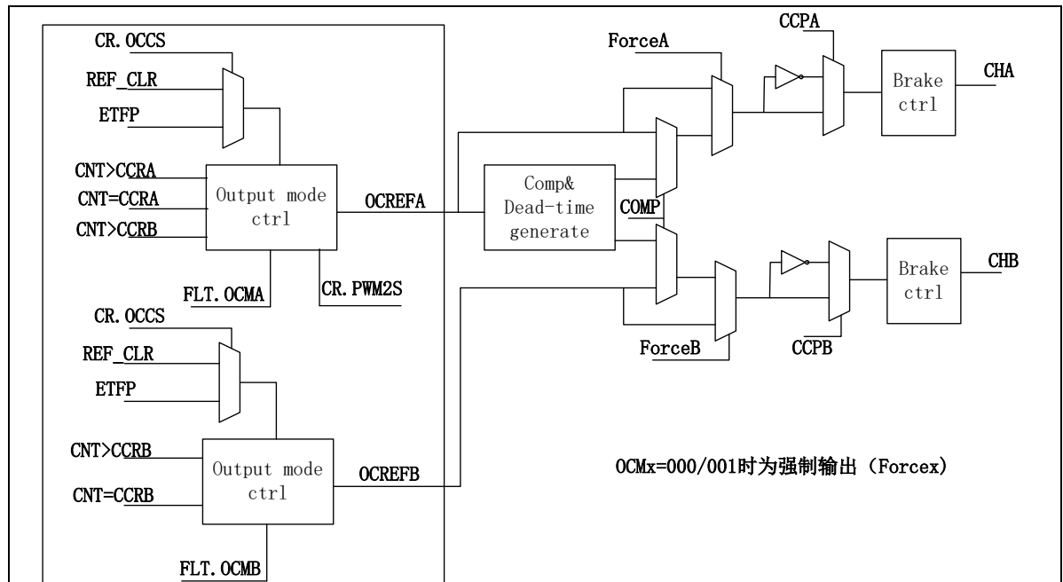
图 13-31 OCREF 输出框图
