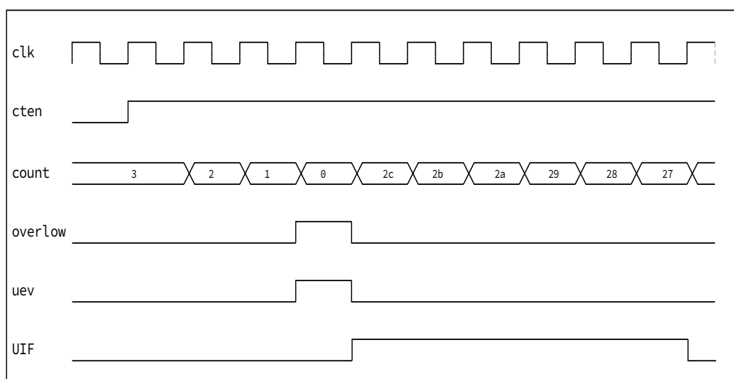
图 13-17 不带预分频的下计数
