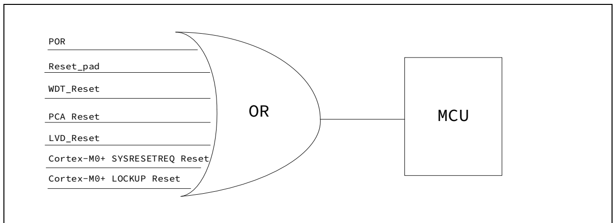
图 4-1 复位来源示意图
