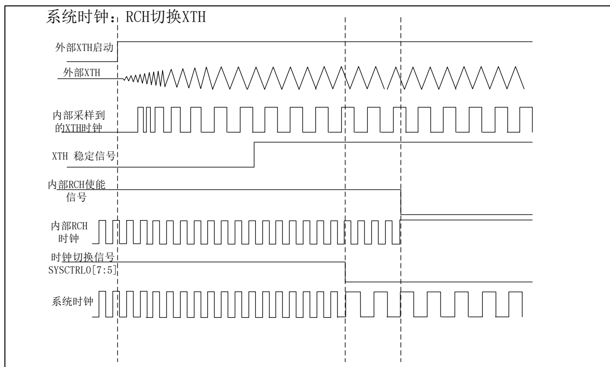
图 3-3 时钟切换示意图
