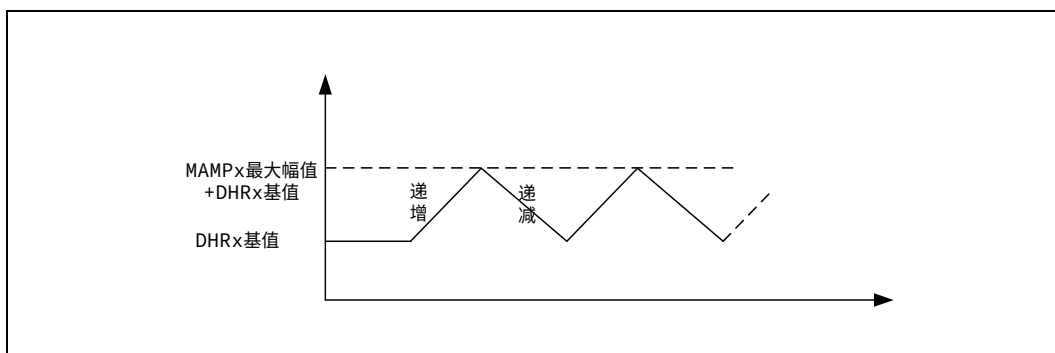
图 23-3 生成 DAC 三角波
