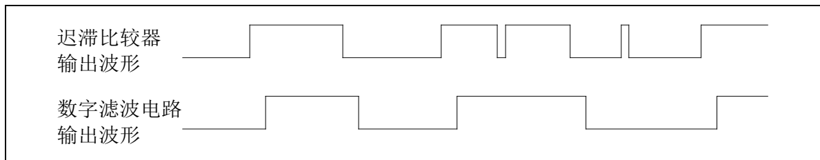
图 25-3 LVD 滤波输出
