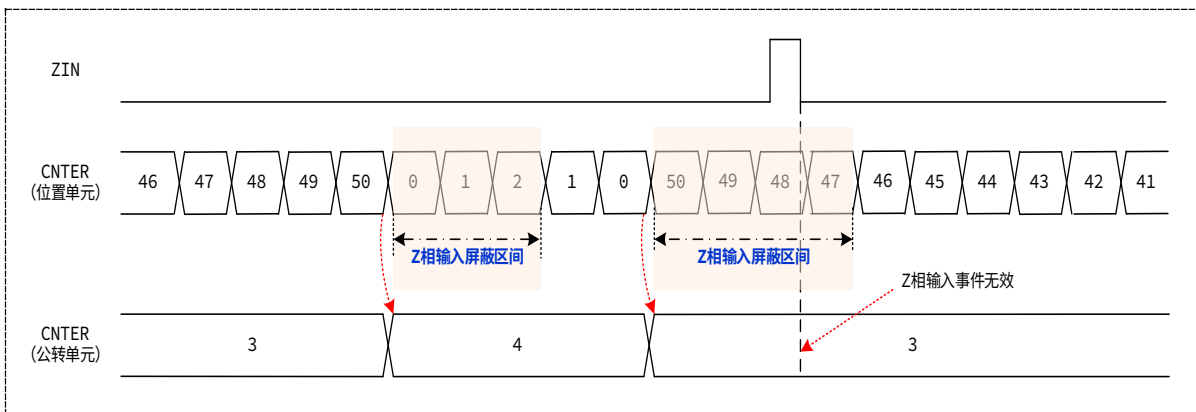
图 15-25 公转计数模式-混合计数 Z 相屏蔽动作例 2
