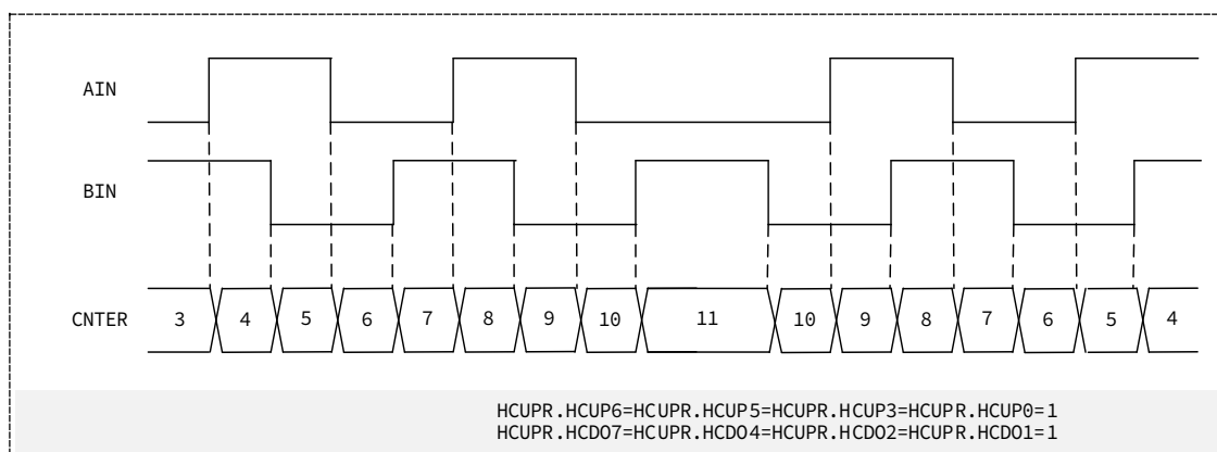
图 15-19 位置模式时相位差计数动作设定 (4 倍)
