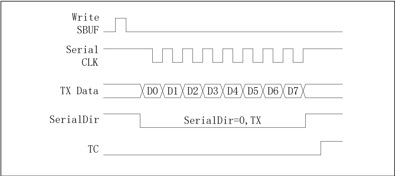
图 17-2 Mode0 发送数据
