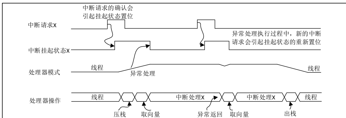
图 5-6 中断处理中产生的中断挂起也可以被确认
