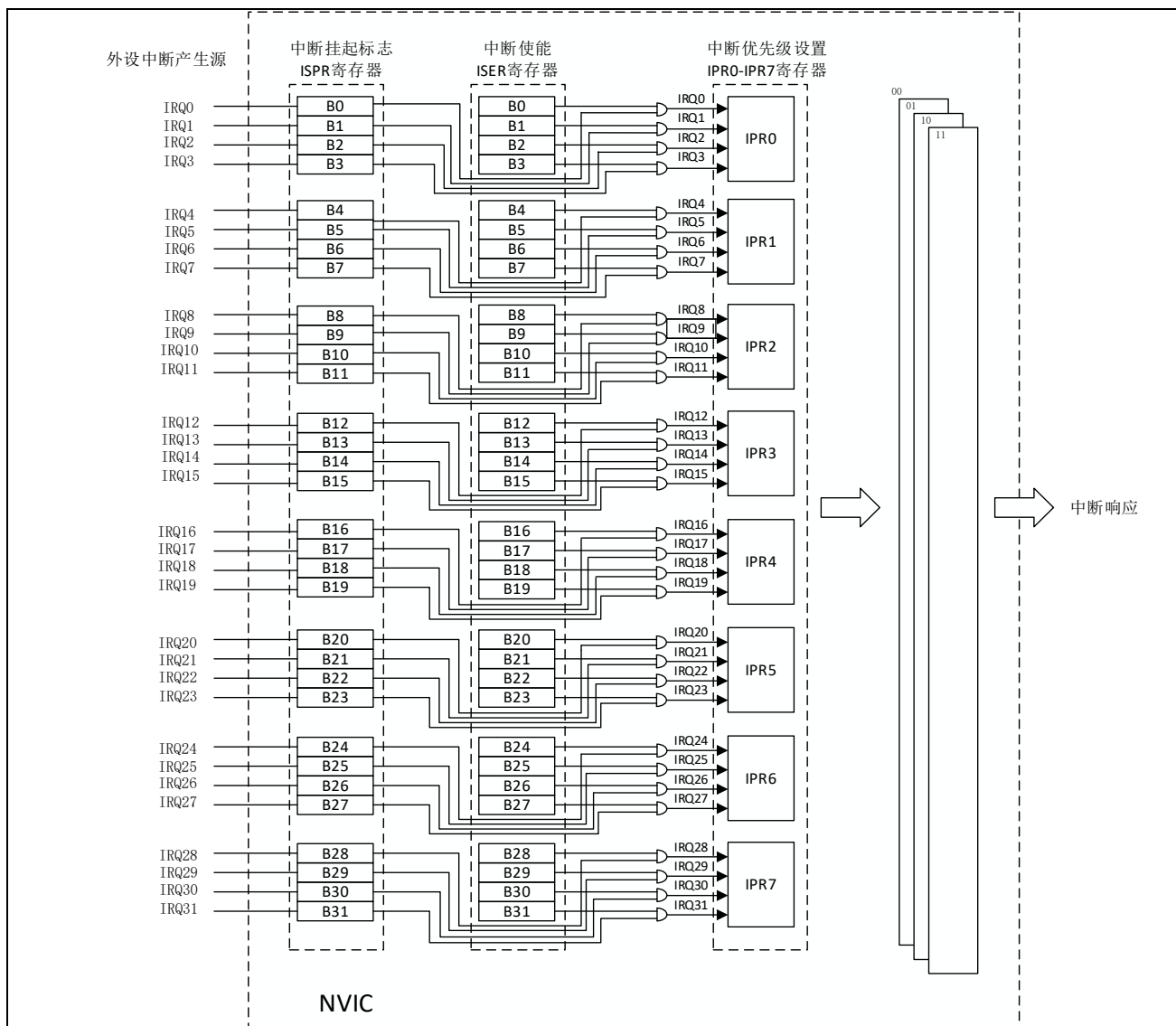
图 5-7 中断结构图
