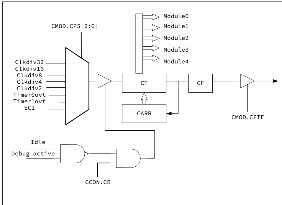
图 14-2 PCA 计数器框图
