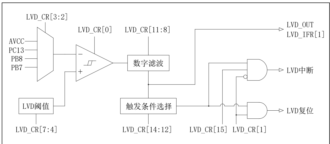
图 25-1 LVD 框图
