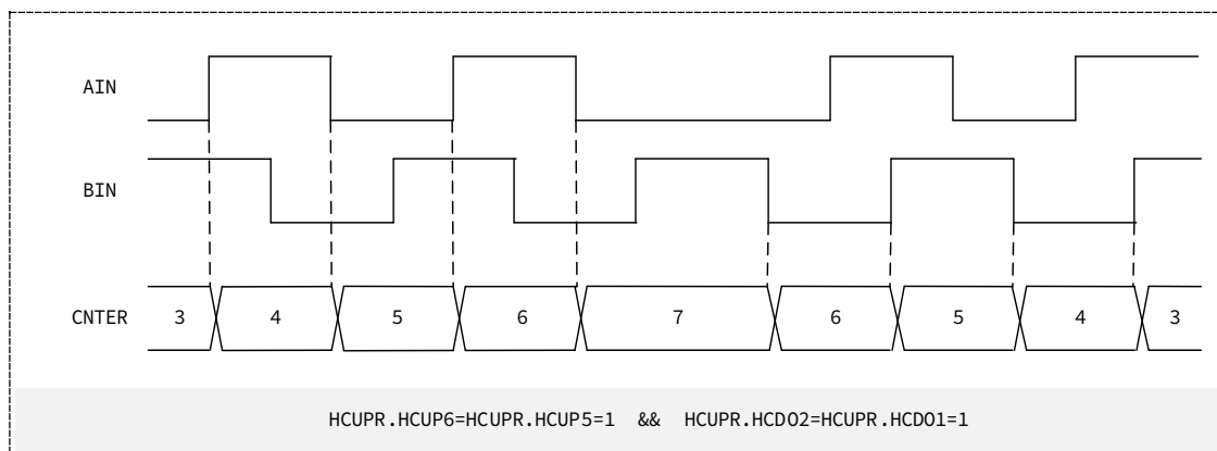
图 15-18 位置模式时相位差计数动作设定 (2 倍)
