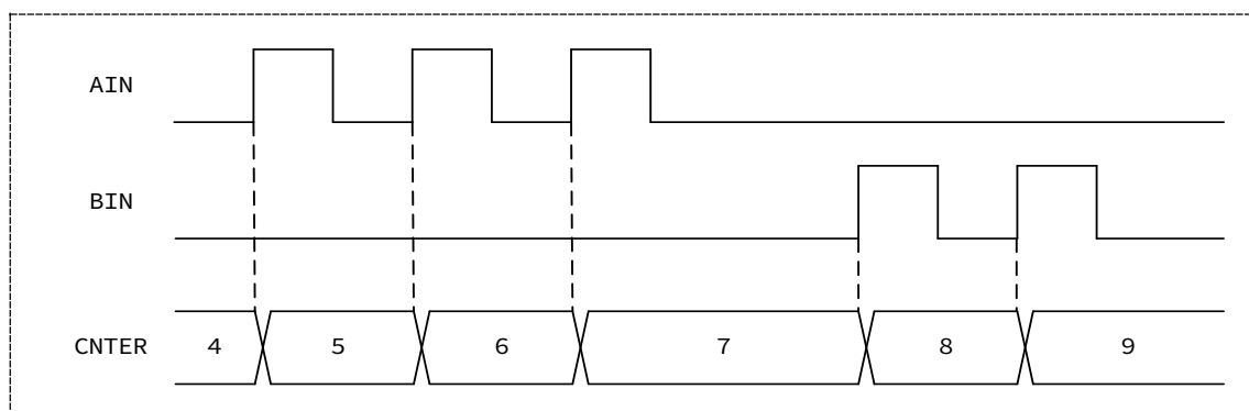
图 15-16 位置模式时基本计数动作
