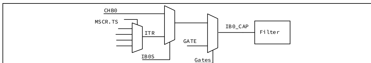
图 13-50 CHB 端口选择
