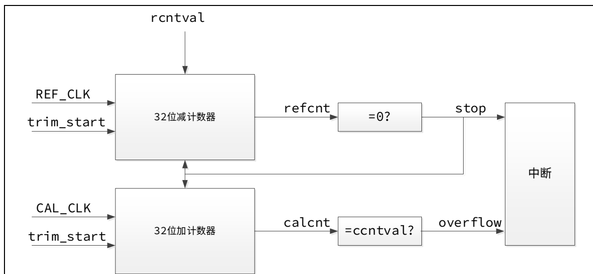
图 9-2 时钟校准模块硬件示意图
