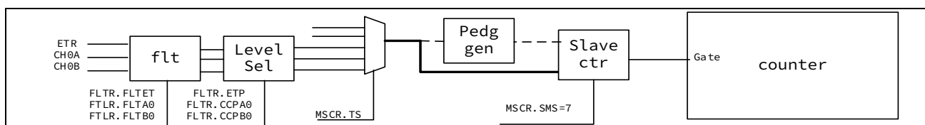
图 13-52 门控功能
