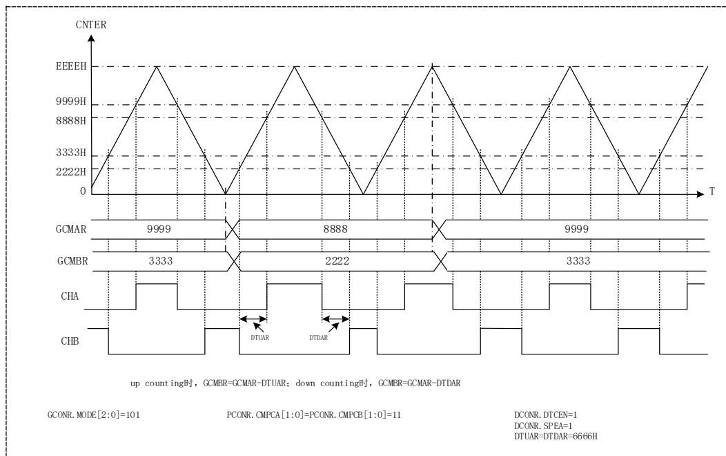
图 15-13 三角波 B 模式时硬件设定 GCMBR 互补 PWM 波输出（对称死区）
