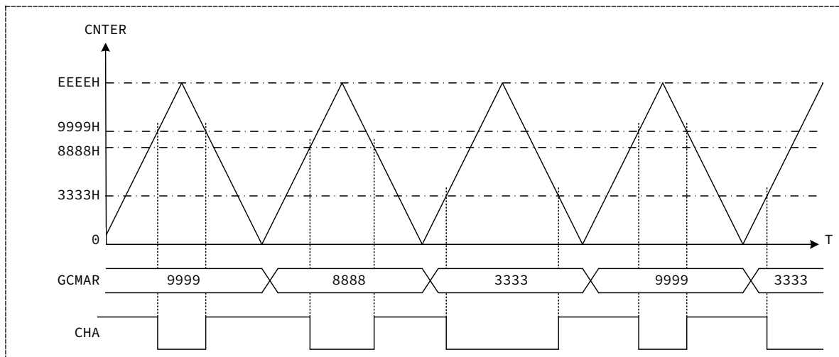
图 15-11 CHA 输出 PWM 波
