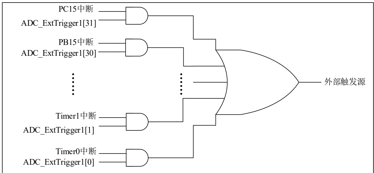
图 22-8 ADC 插队扫描转换外部触发源示意图
