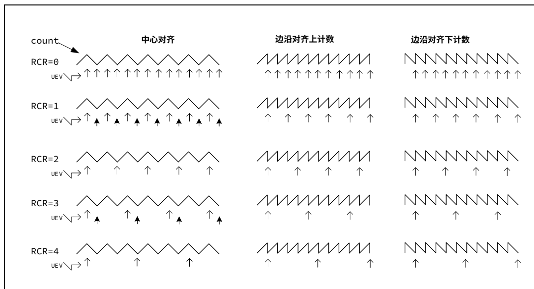
图 13-23 重复计数器产生更新时序
