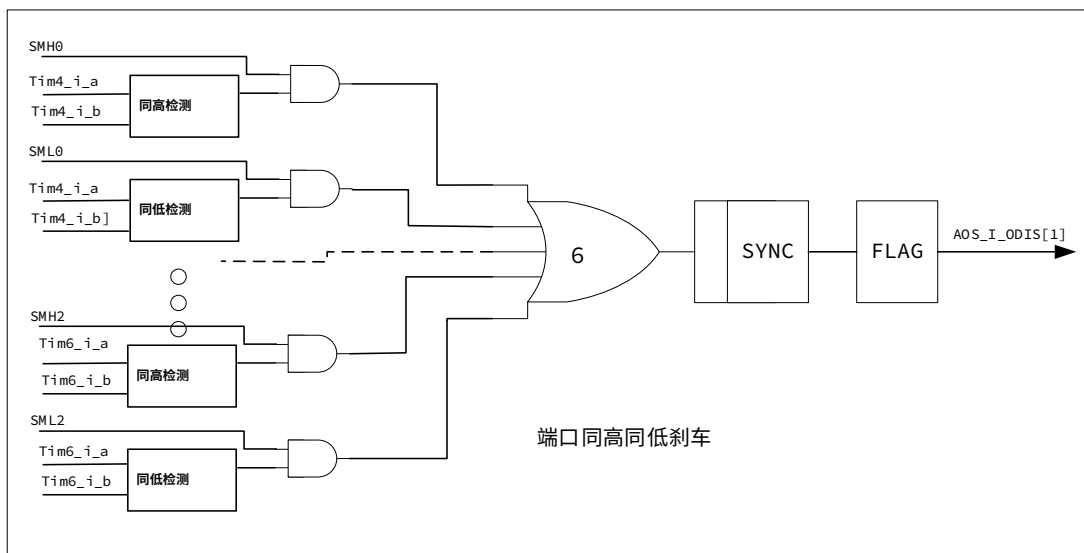
图 15-28 输出同高同低刹车示意图
