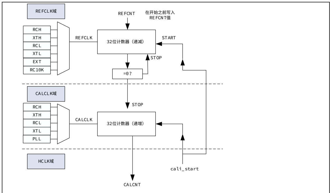
图 3-4 时钟校准原理图
