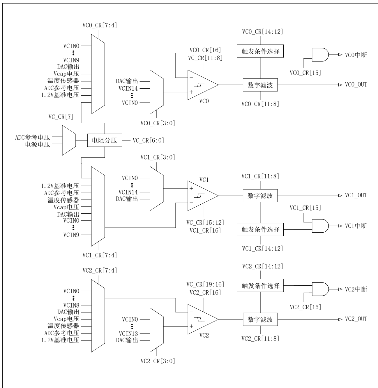
图 24-1 VC 框架图
