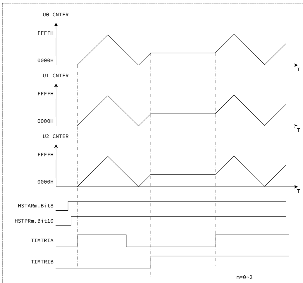
图 15-8 硬件同步动作
