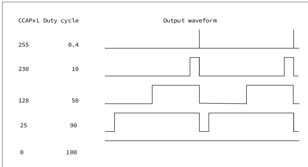
图 14-8 PCA PWM 输出波形
