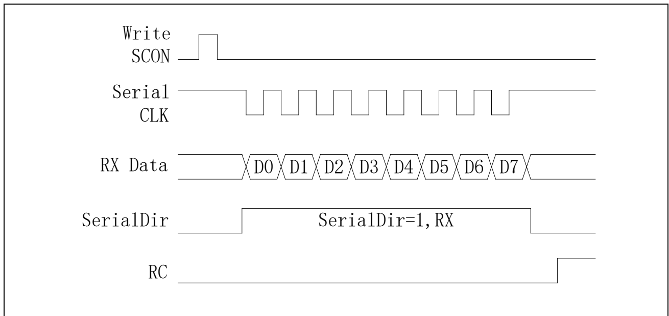
图 17-3 Mode0 接收数据
