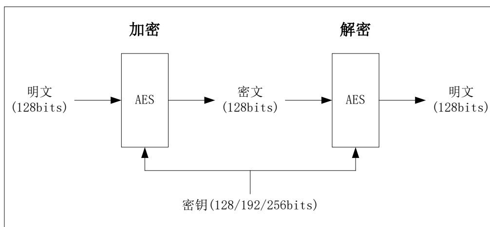
图 20-1 AES 的加解密示意图
