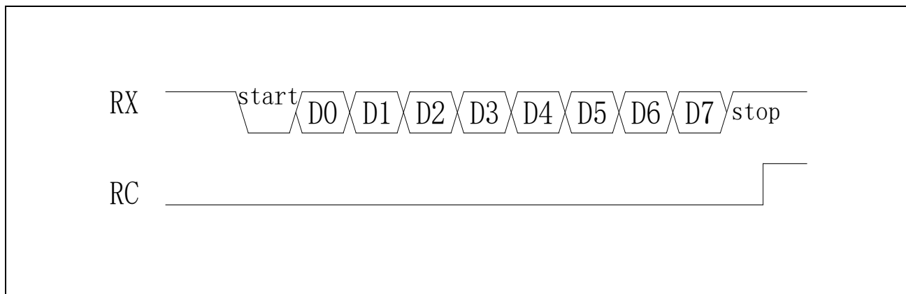
图 17-5 Mode1 接收数据
