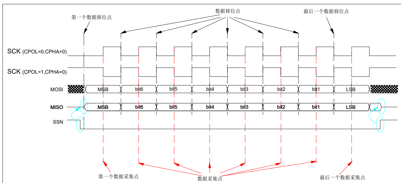
图 8-4 从机 CPHA 为 0 时数据帧格式
