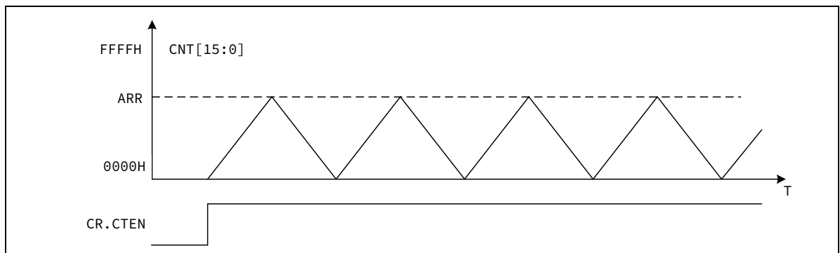
图 13-22 中心对齐计数器波形
