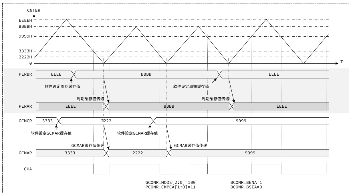
图 15-9 单缓存方式比较输出时序
