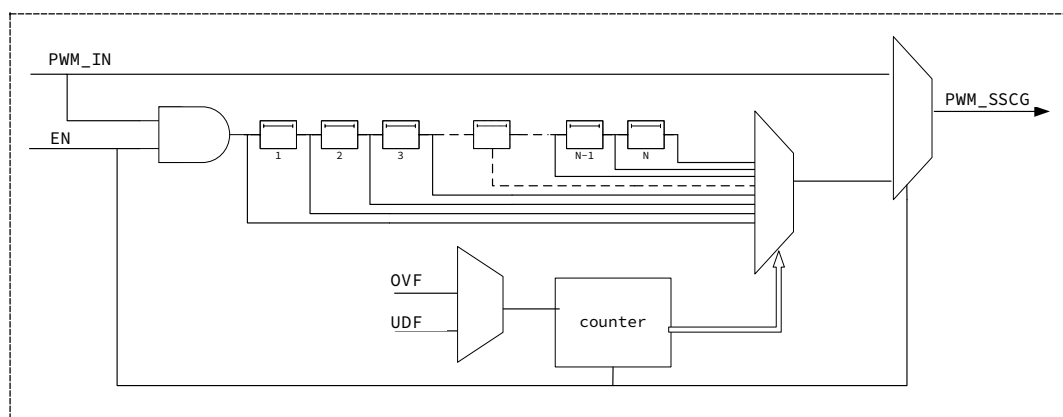
图 15-10 PWM 展频输出示意图
