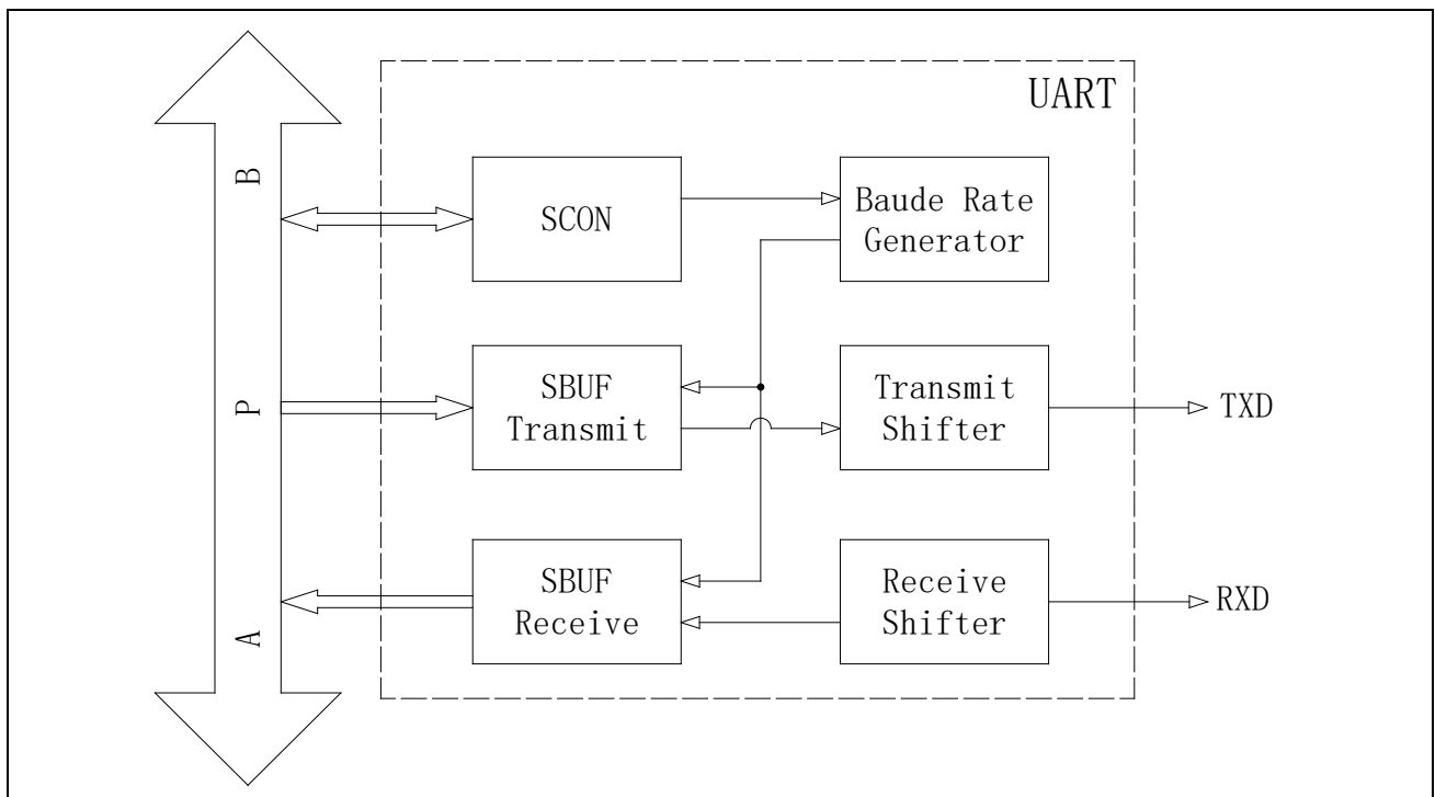
图 17-1 结构框图
