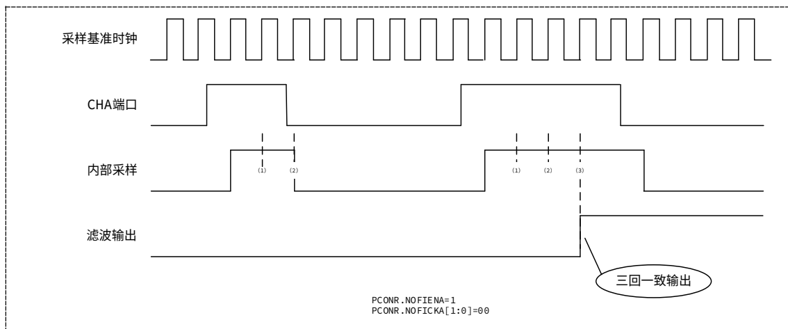
图 15-6 捕获输入端口的滤波功能
