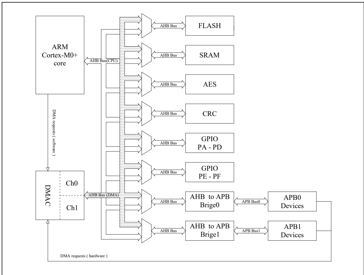
图 12-1 功能框图
