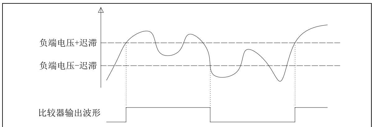
图 24-3 VC 迟滞功能
