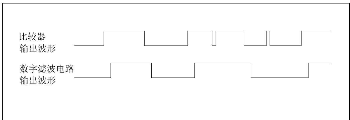
图 24-2 VC 滤波响应时间
