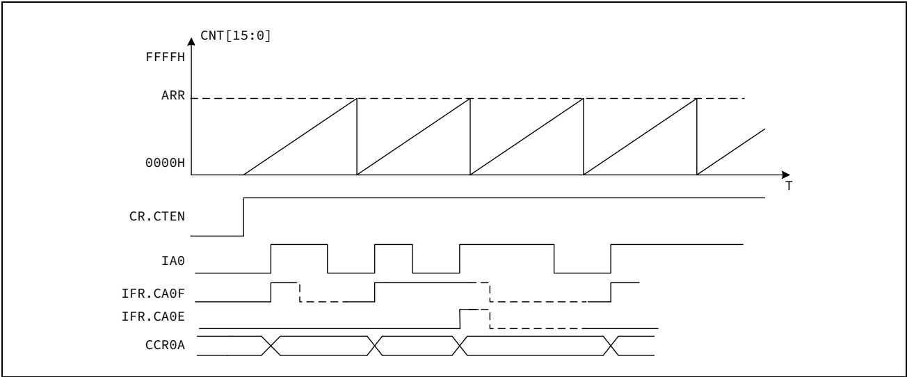
图 13-48 捕获时序图
