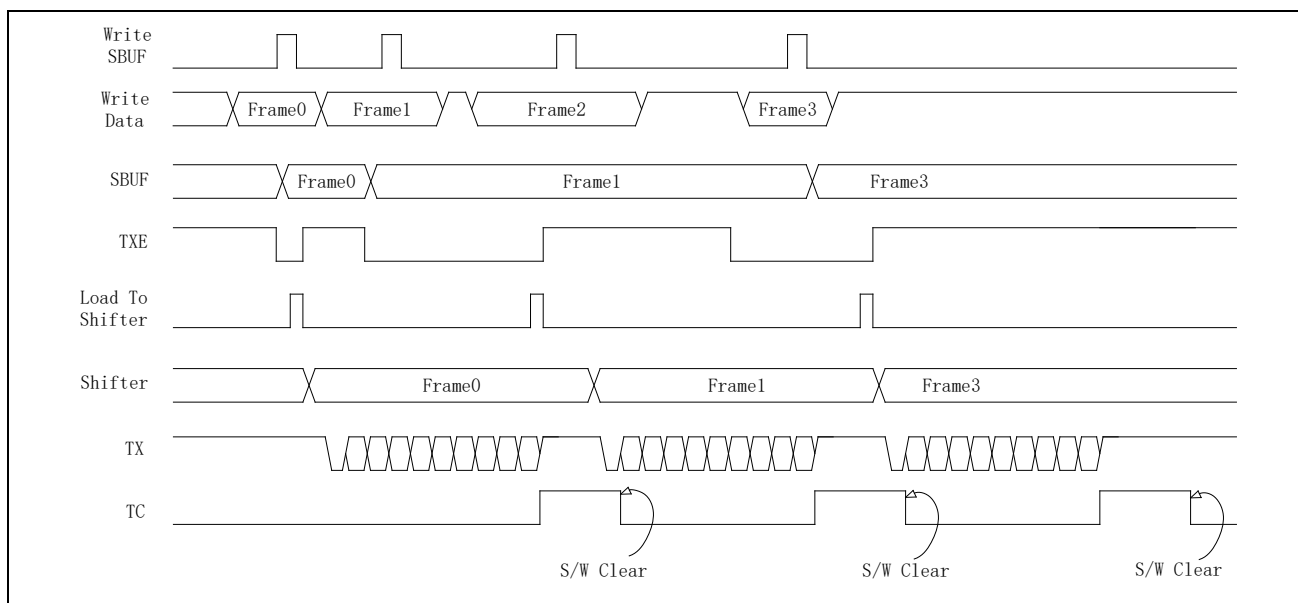
图 17-14 发送缓存
