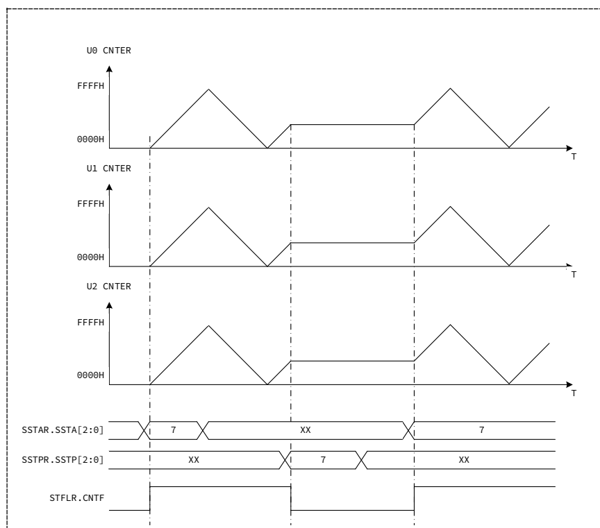
图 15-7 软件同步动作
