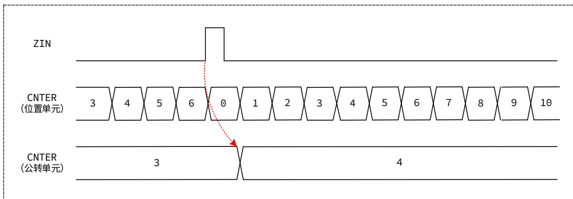
图 15-21 公转模式时 Z 相计数动作
