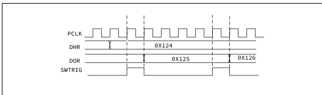
图 23-4 生成三角波波形的 DAC 转换（使能软件触发）
