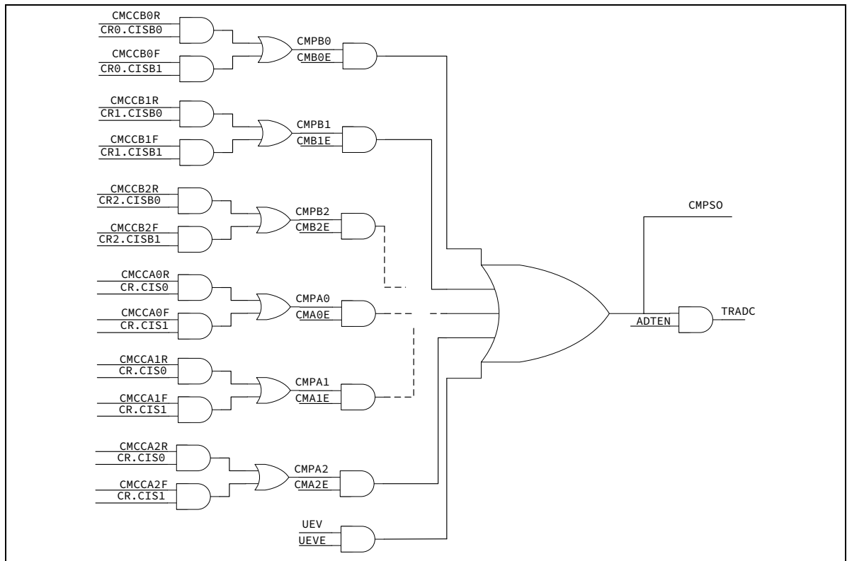
图 13-55 ADC 触发
