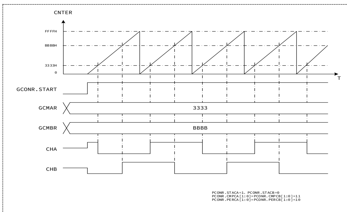
图 15-4 比较输出动作
