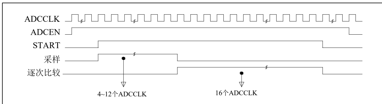
图 22-2 ADC 转换时序图
