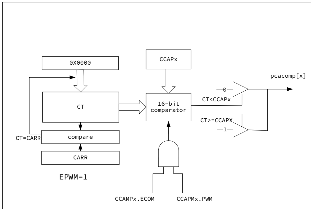
图 14-5 PCA 16 位 PWM 功能框图
