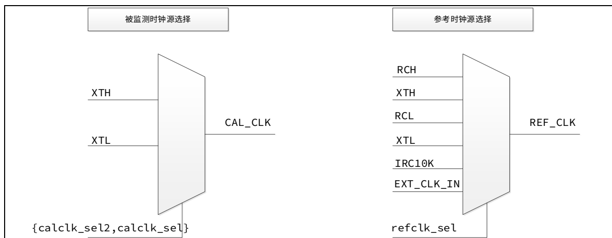
图 9-4 CLKTRIM 时钟选择
