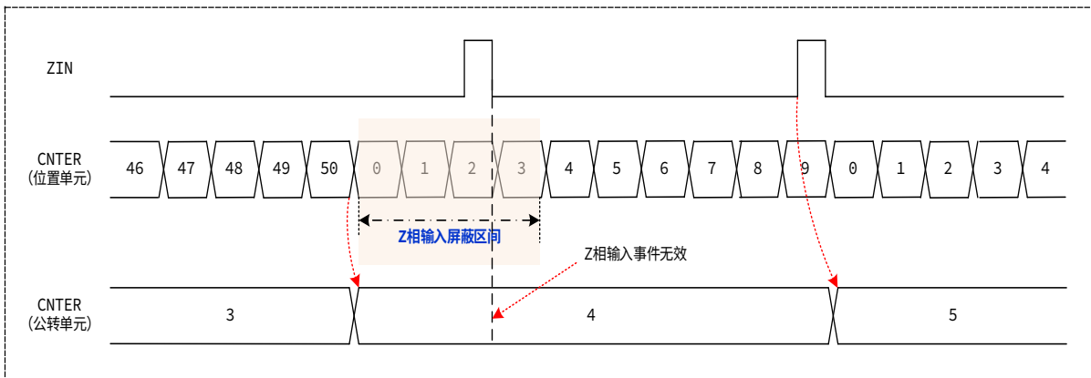
图 15-24 公转计数模式-混合计数 Z 相屏蔽动作例 1
