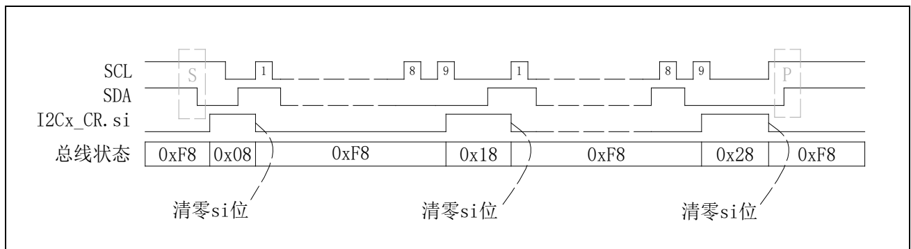
图 7-7 主发送模式数据同步图
