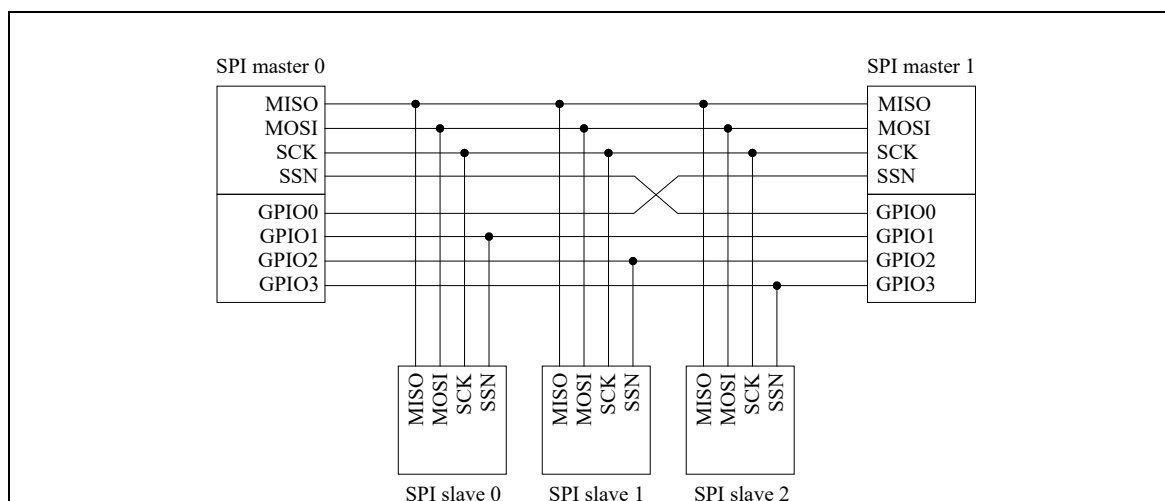
图 8-6 SPI 多主机/多从机系统的示意图
