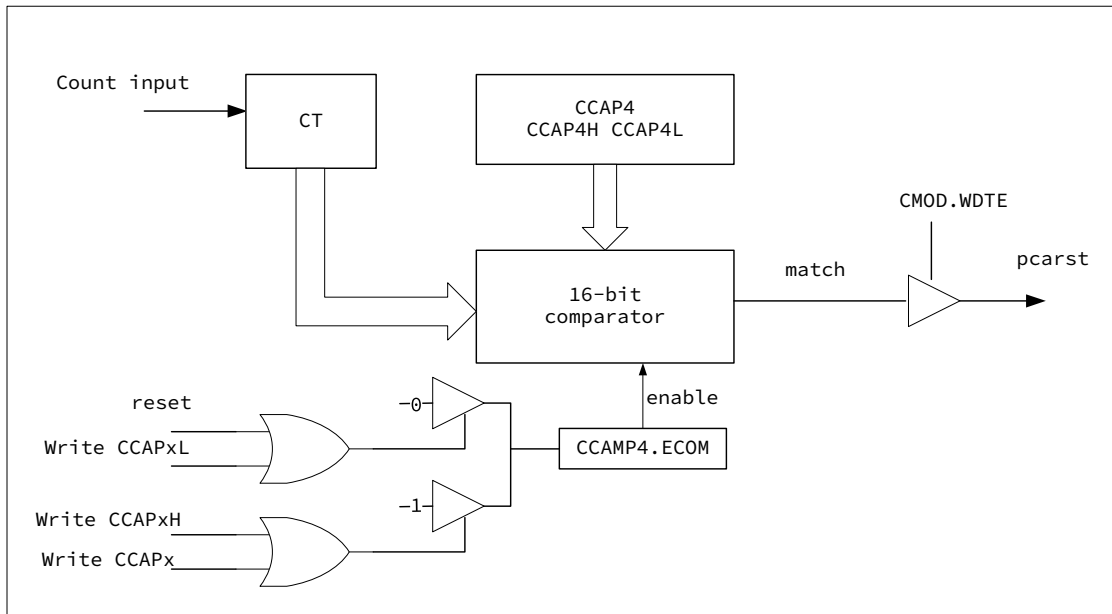
图 14-6 PCA WDT 功能框图
