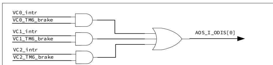
图 15-29 VC 刹车控制示意图
