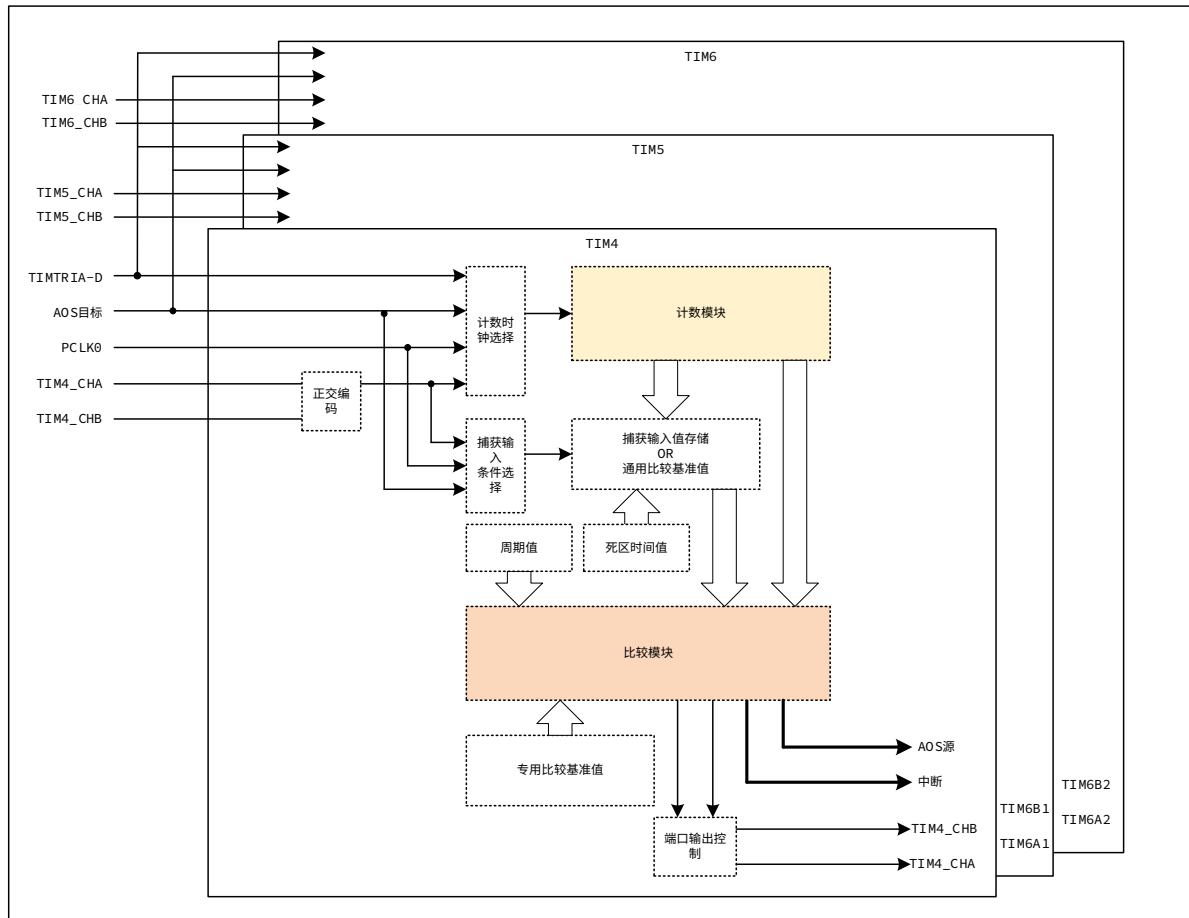
图 15-1 Advanced Timer 框图
