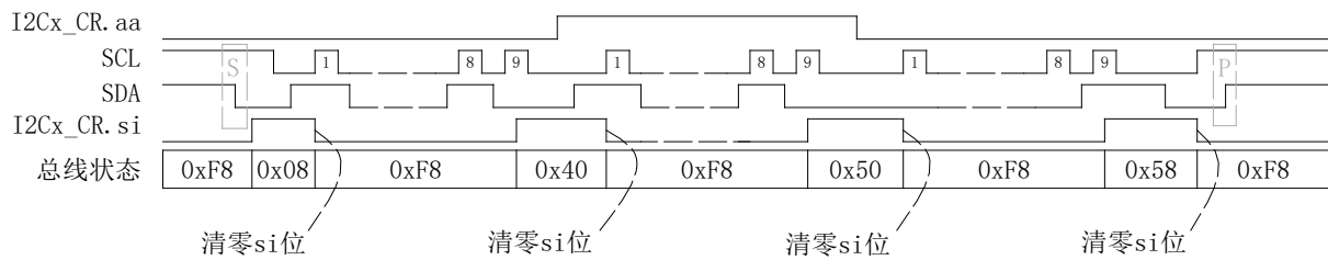
图 7-9 主接收模式数据同步图
