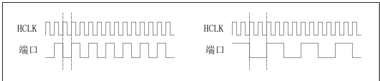
图 6-2 AHB/FAST I/O 总线端口随系统时钟的变化
