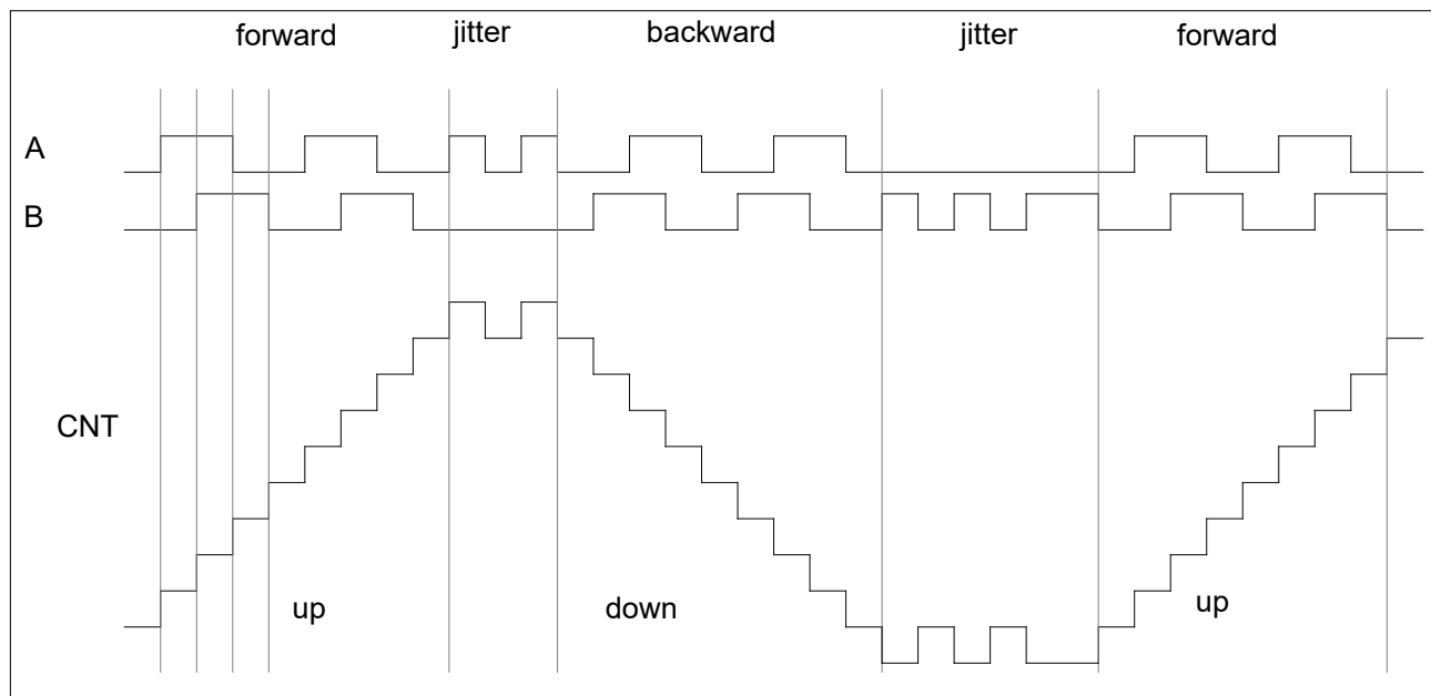
图 13-54 编码计数
