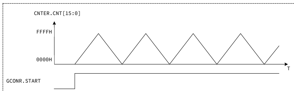
图 15-3 三角波波形
