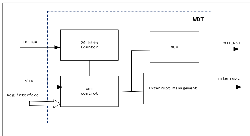
图 16-1 WDT 整体框图
