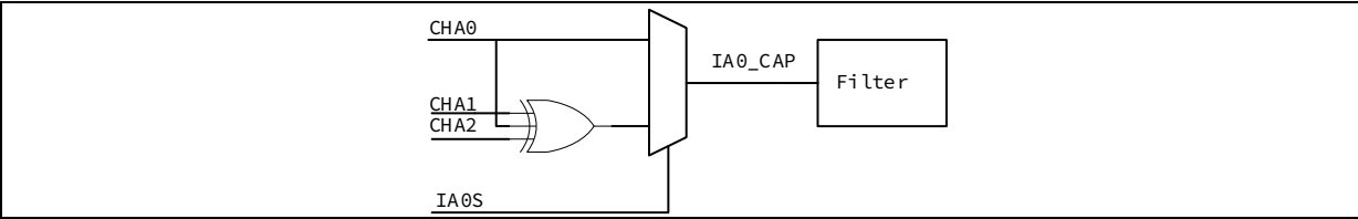
图 13-49 CHA 端口选择
