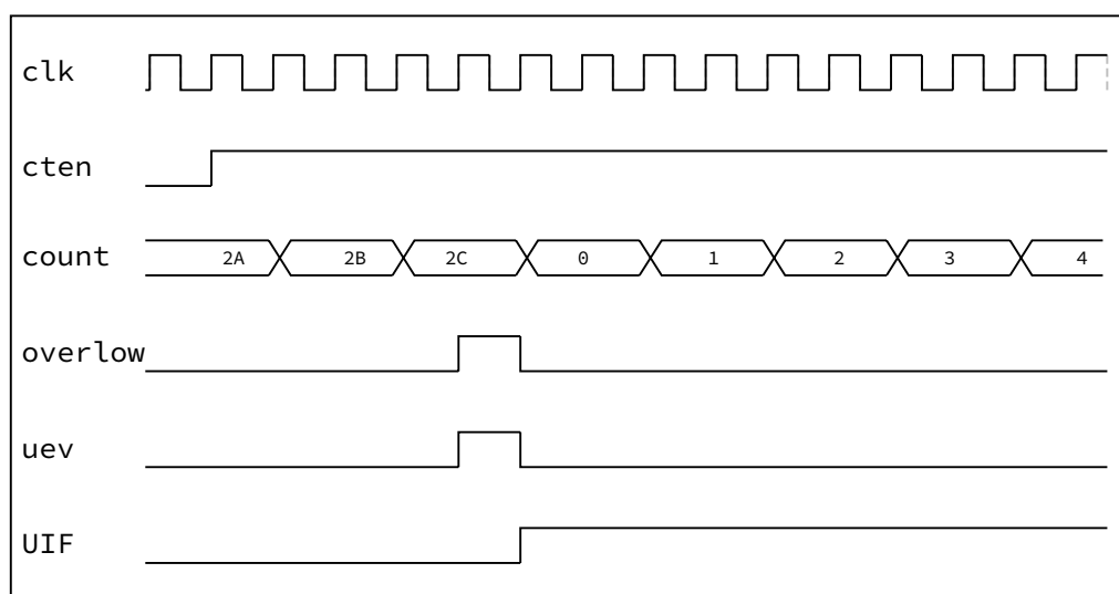
图 13-16 带预分频的上计数
