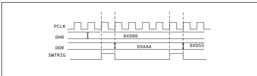
图 23-2 LFSR 产生波形的 DAC 转换（使用软件触发）
