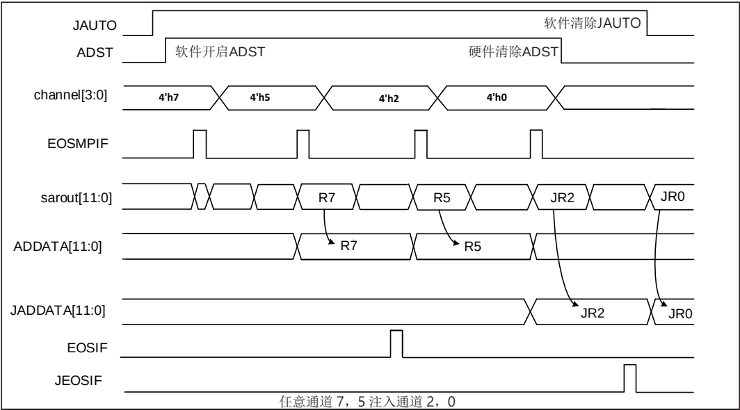
图 18-12 自动注入通道转换单周期扫描通道转换时序图
