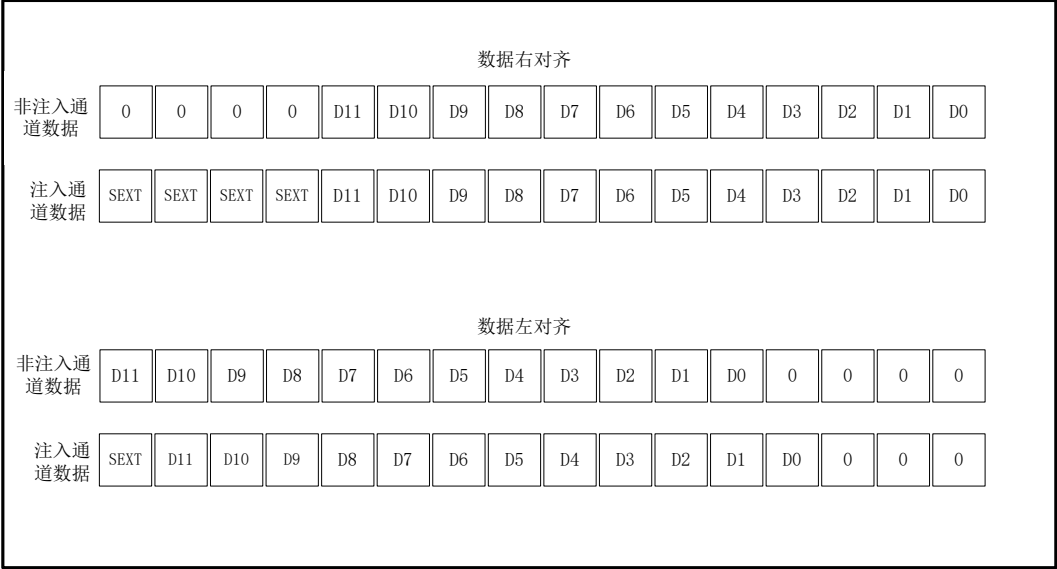
图 18-2 数据对齐方式
