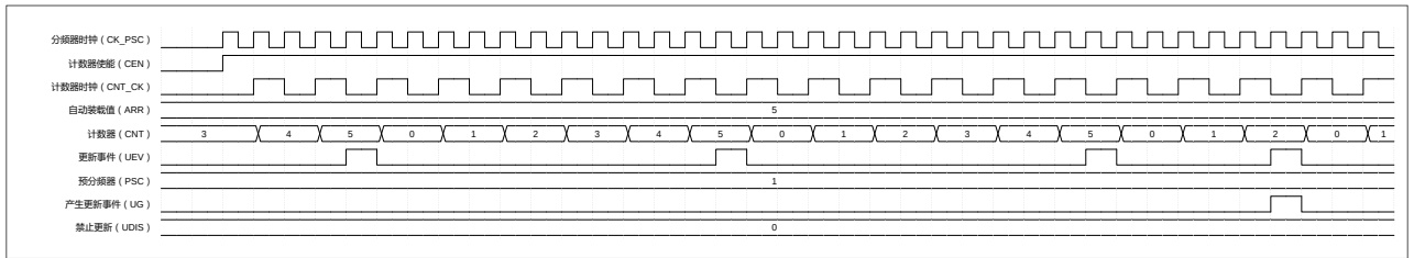
图 9-6 递增计数模式（UDIS=0）
