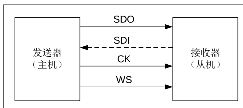
图 14-9 I2S 主模式（SD 配置成 SDO 为发送器，配置成 SDI 为接收器）
