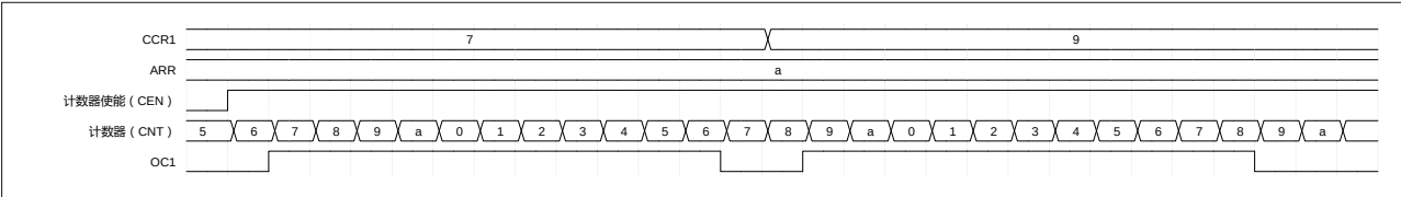
图 9-15 比较输出模式，OC1 信号在匹配时翻转
