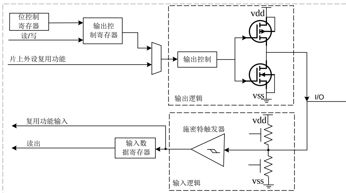
图 8-4 复用功能配置
