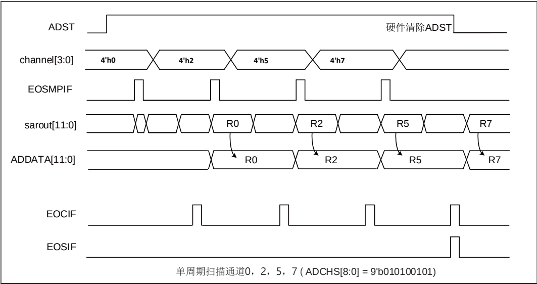
图 18-5 单周期扫描下使能通道转换时序图（通道方向从低到高）
