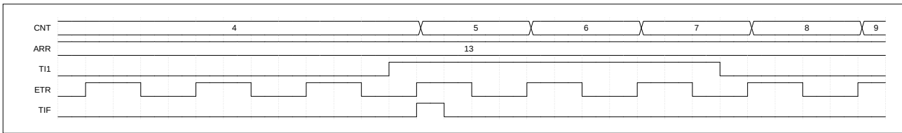
图 9-26 外部时钟模式 2+从模式（触发模式）控制时序图
