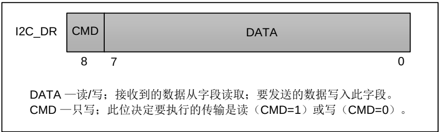
图 17-9 I2C_DR 寄存器
