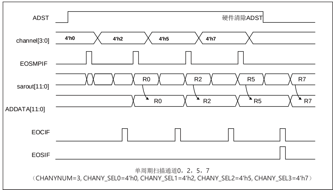
图 18-9 单周期扫描下通道转换时序图
