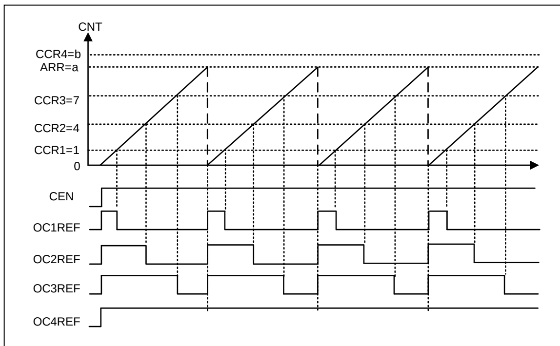
图 9-16 边沿对齐递增计数时 PWM 模式 1 的波形
