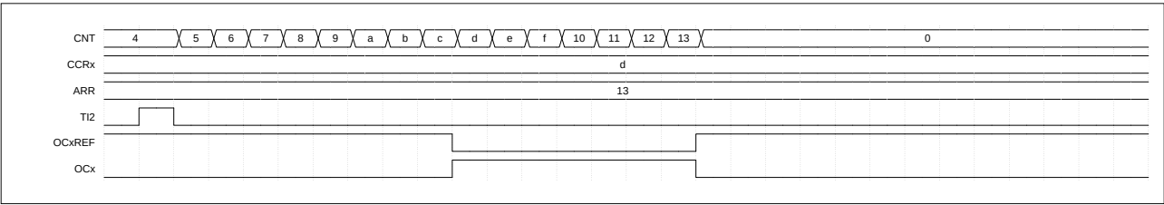
图 9-20 单脉冲模式
