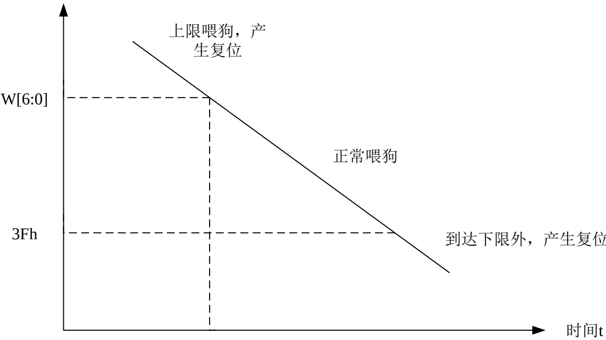
图 13-2 WWDG 超时时间坐标图
