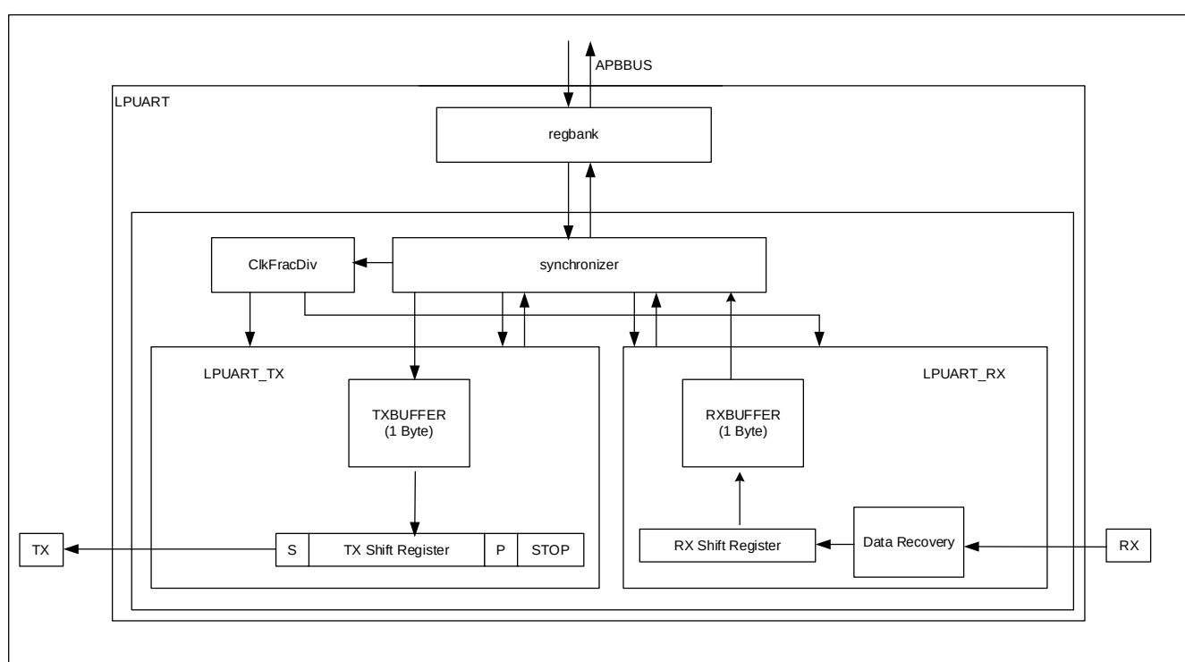
图 16-1 LPUART 功能框图
