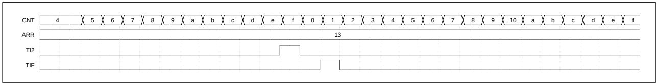
图 9-23 复位模式的控制时序图
