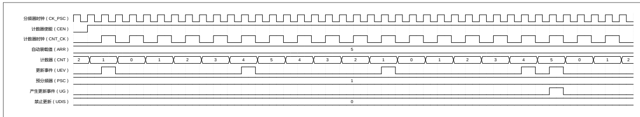
图 9-10 中央计数模式（UDIS=0）
