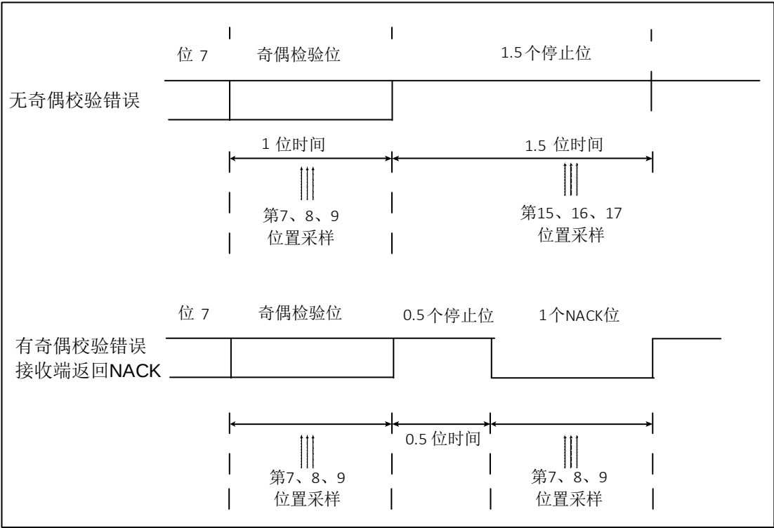
图 15-6 UART 采样 NACK 信号方框图
