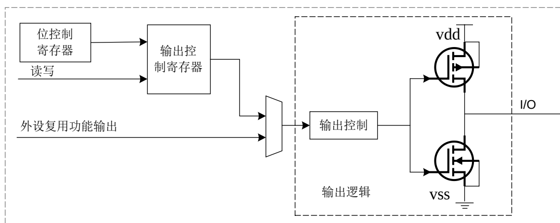
图 8-3 输出配置
