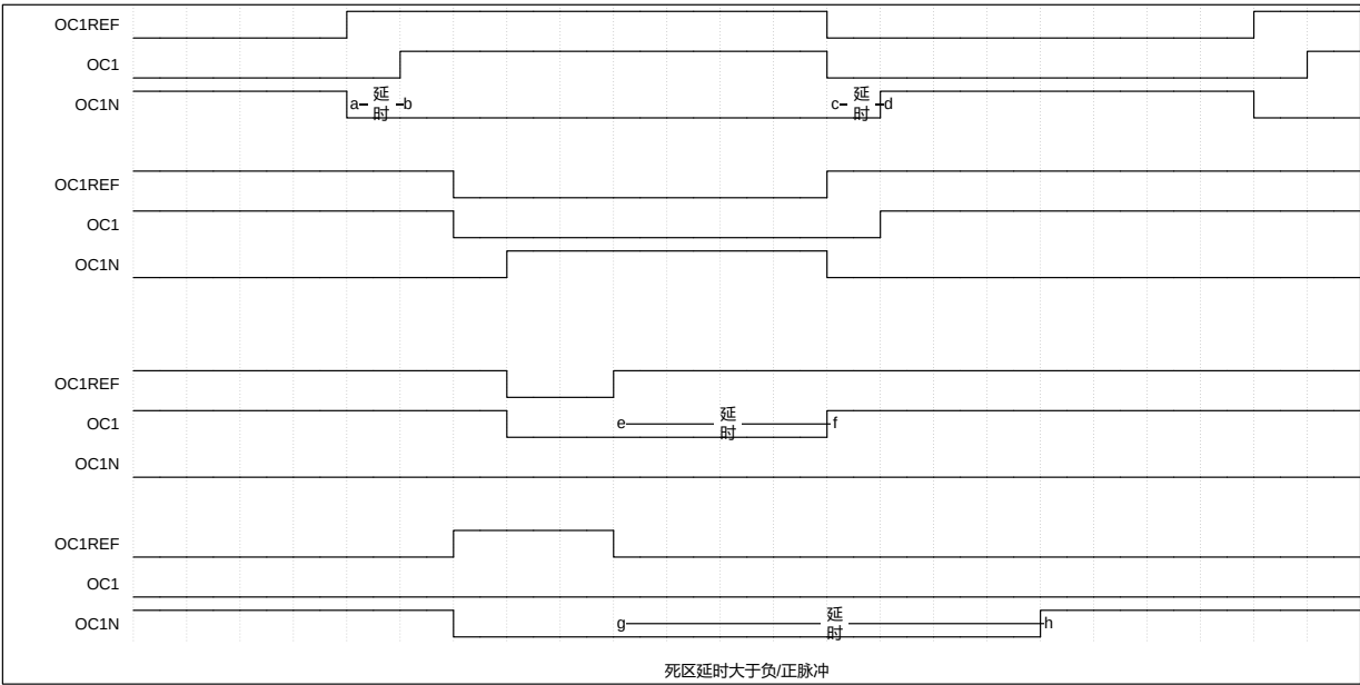
图 10-9 死区插入
