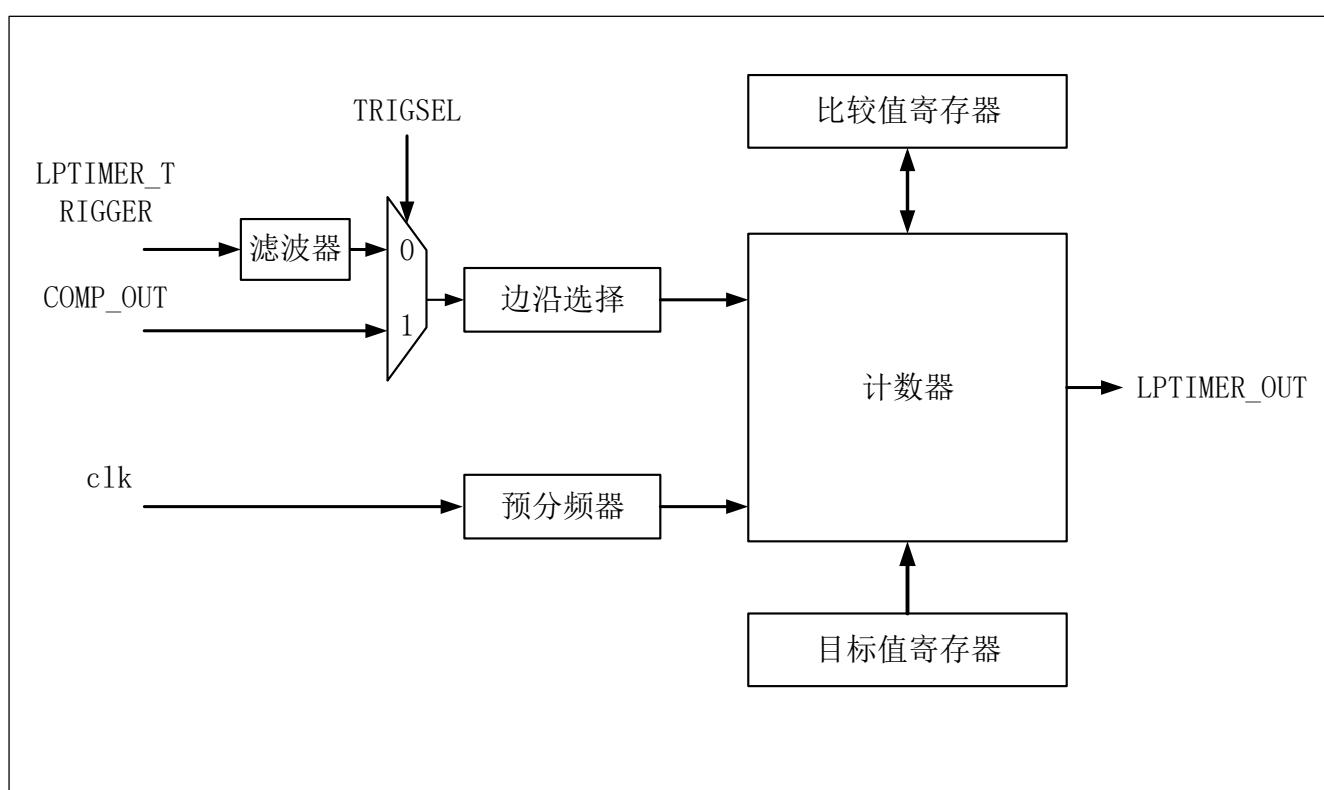
图 11-1 功能框图
