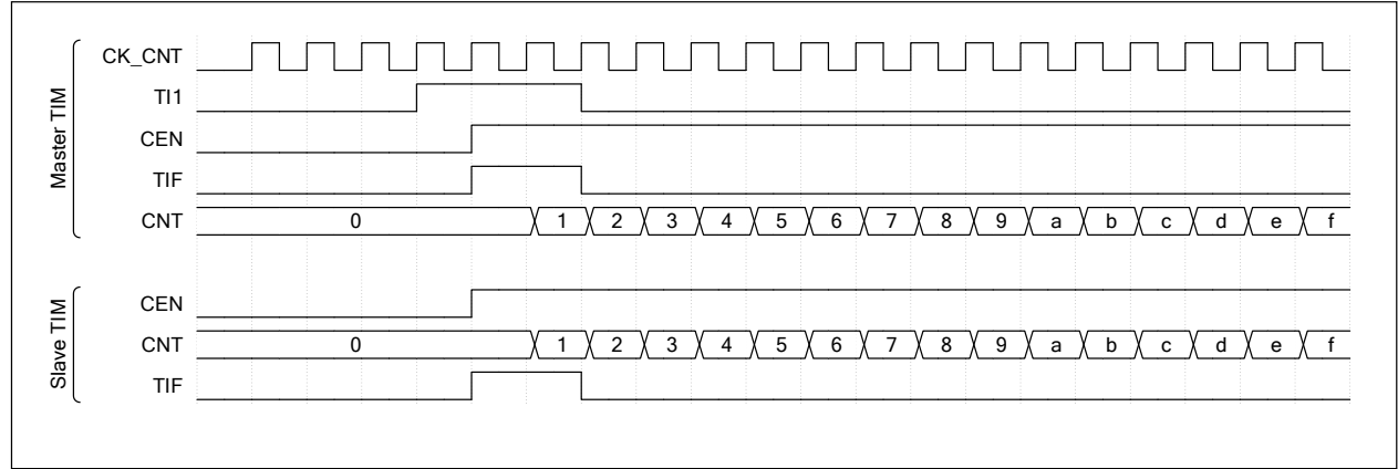
图 9-31 主定时器的 TI1 同步启动主定时器和从定时器
