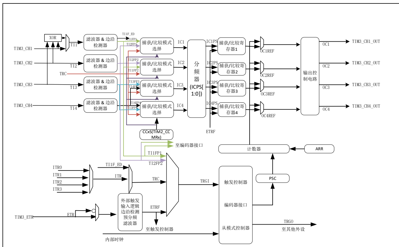
图 9-1 TIMx 结构图
