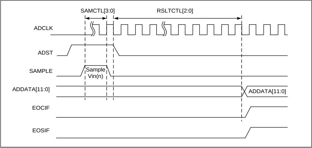
图 18-3 单次转换模式时序图
