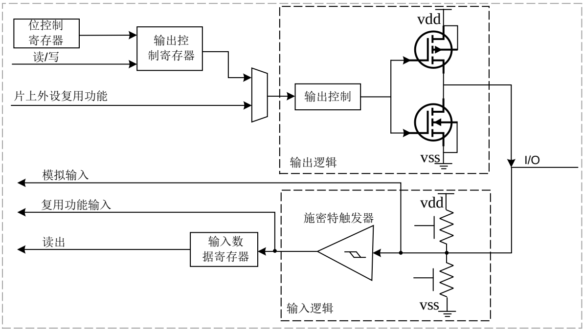
图 8-1 标准 I/O 端口
