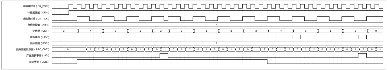
图 10-4 递增计数模式（UDIS=1 禁止产生更新事件）
