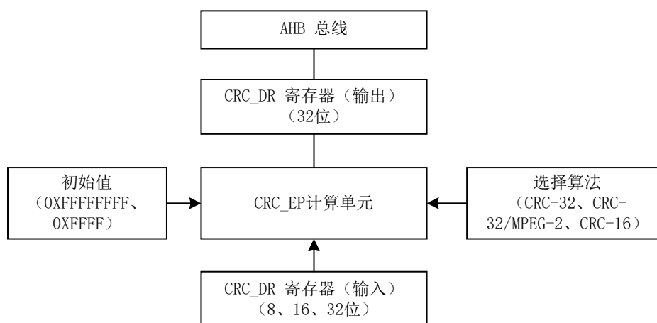
图 7-1 CRC_EP 功能框图
