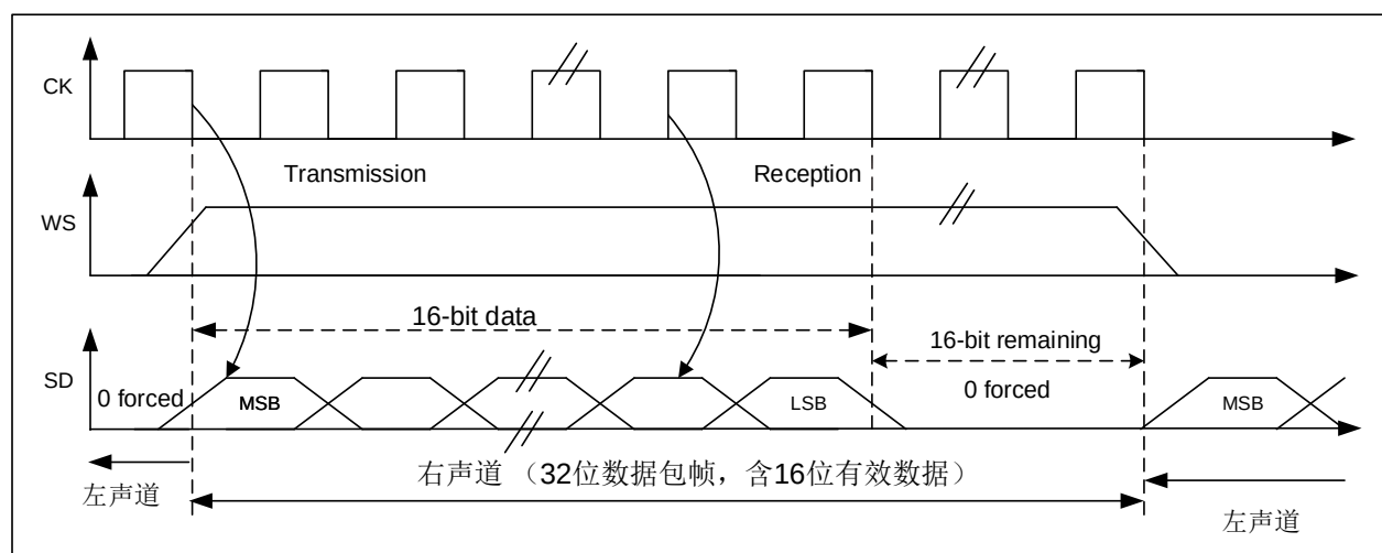
图 14-5 MSB 对齐标准示意图
