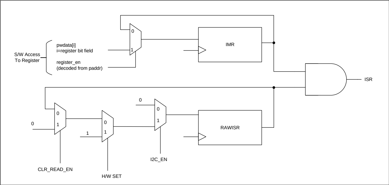
图 17-20 I2C 中断机制
