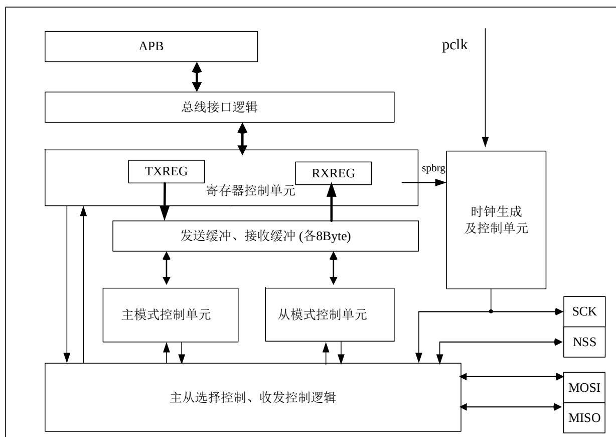
图 14-1 SPI_I2S 功能框图
