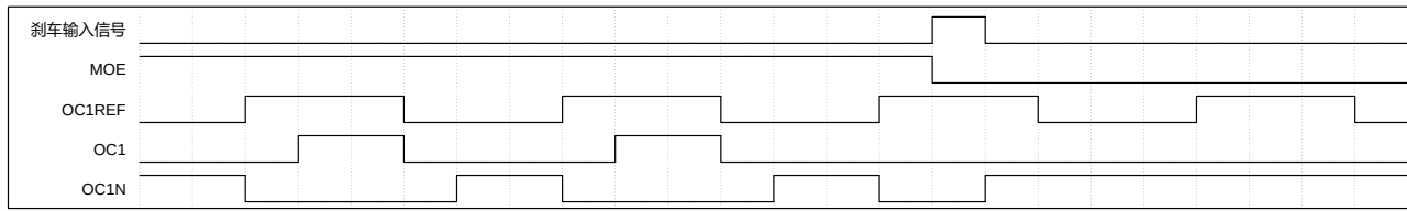
图 10-11 响应刹车的输出（OISx=0，OISxN=1）
