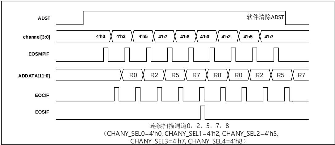
图 18-10 连续扫描模式下通道转换时序图
