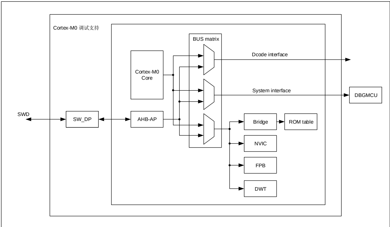
图 21-1 调试功能框图
