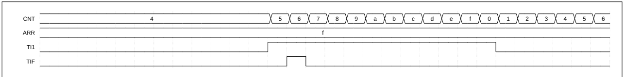
图 9-25 触发器模式下的控制时序图
