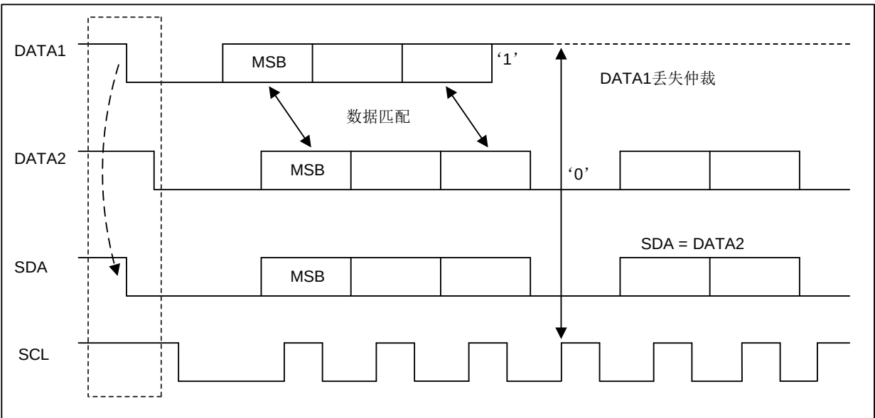
图 17-14 两个主器件仲裁
