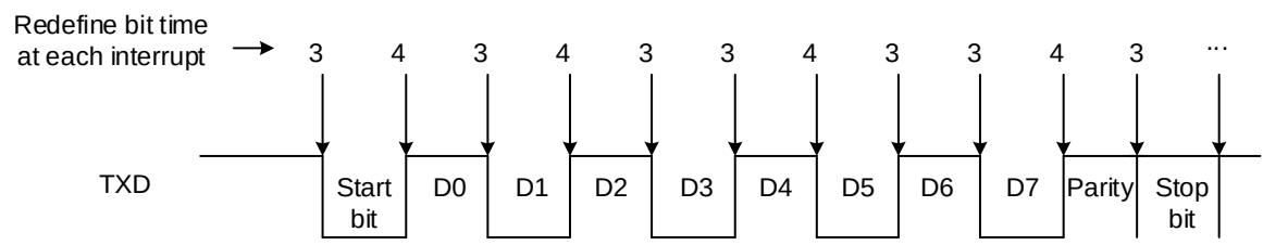
图 16-4 发送时序
