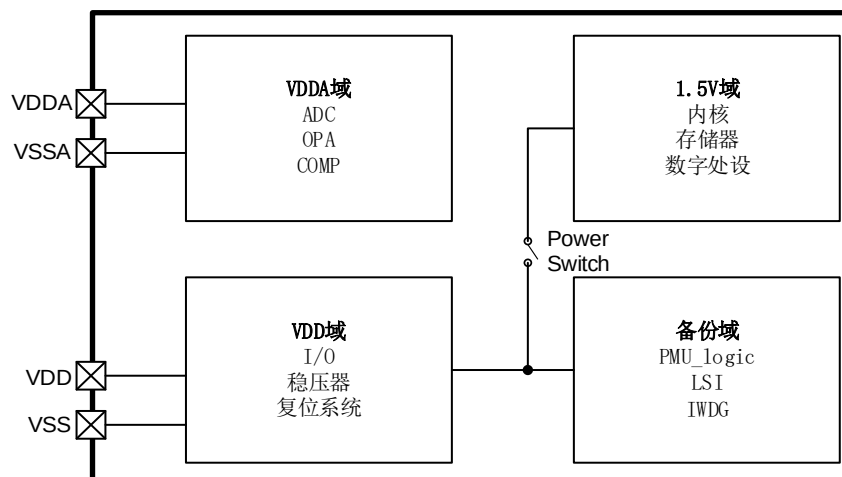
图 3-1 电源控制功能框图
