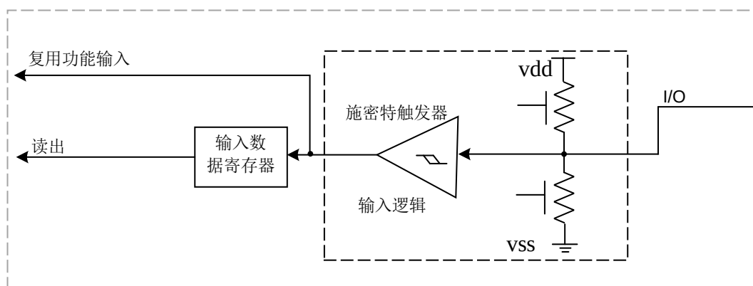
图 8-2 输入浮空/上拉/下拉配置
