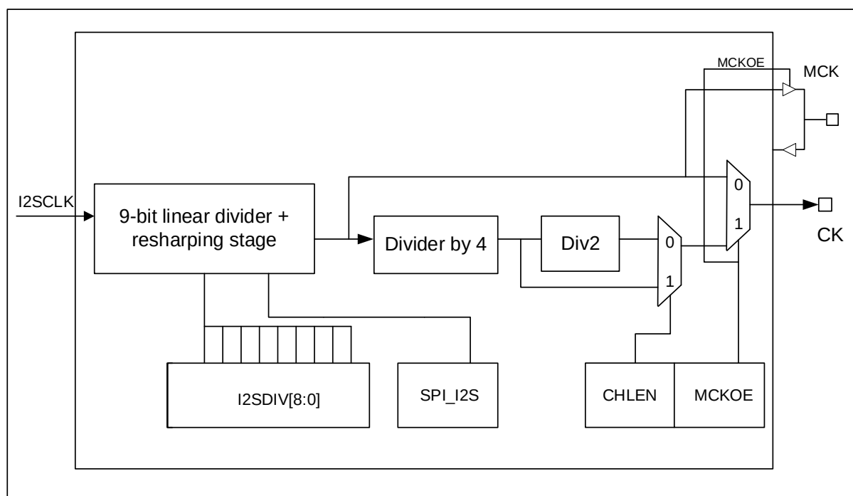
图 14-10 I2S 时钟预分频器示意图
