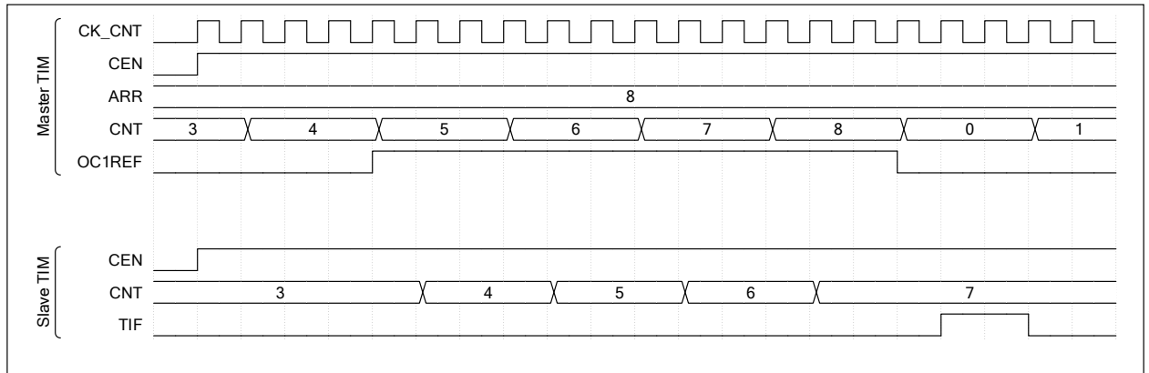
图 9-29 使用主定时器使能从定时器
