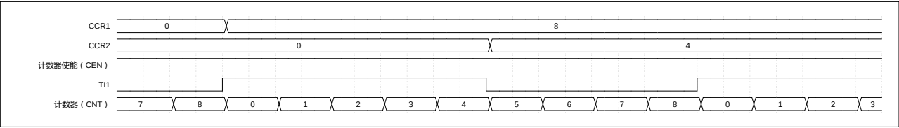
图 9-13 PWM 输入模式时序
