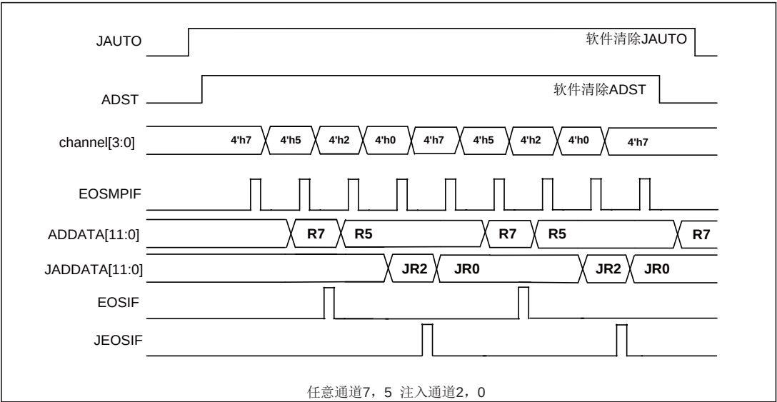
图 18-13 自动注入通道转换连续转换时序图
