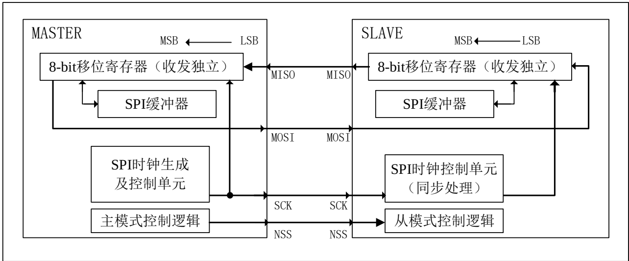
图 14-2 单主和单从应用
