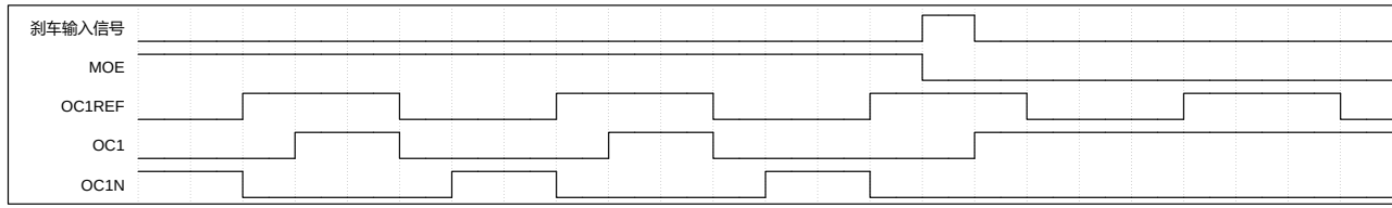
图 10-12 响应刹车的输出（OISx=1，OISxN=0）
