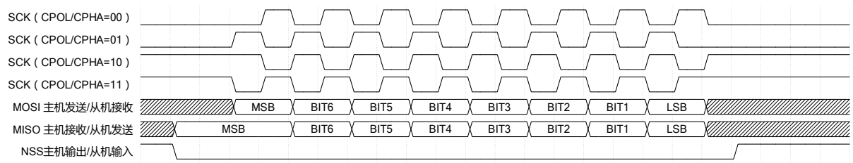
图 14-3 数据时钟时序图
