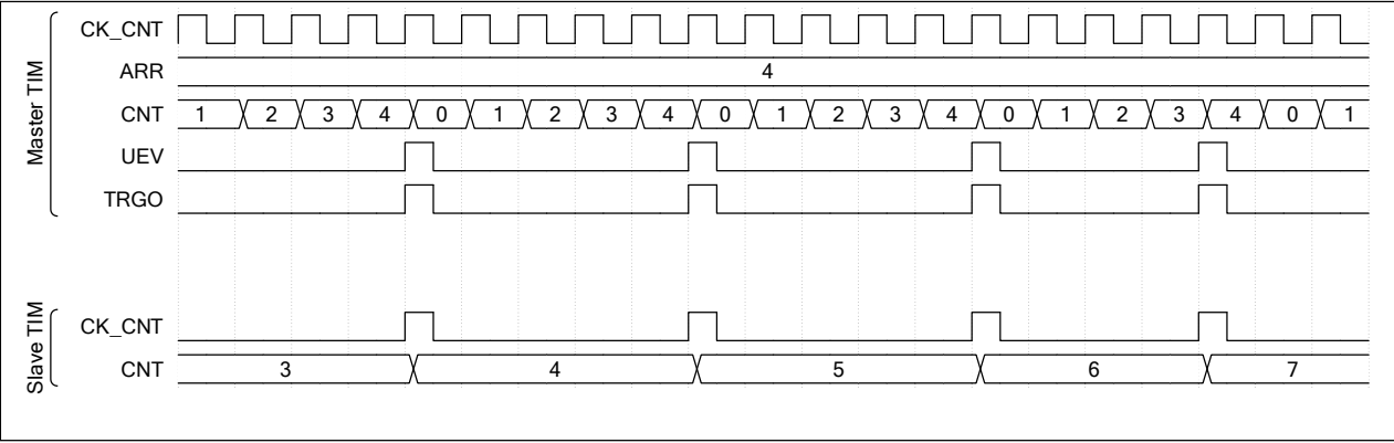
图 9-28 使用主定时器作为从定时器的预分频器
