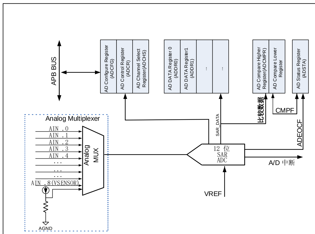
图 18-1 ADC 系统框图
