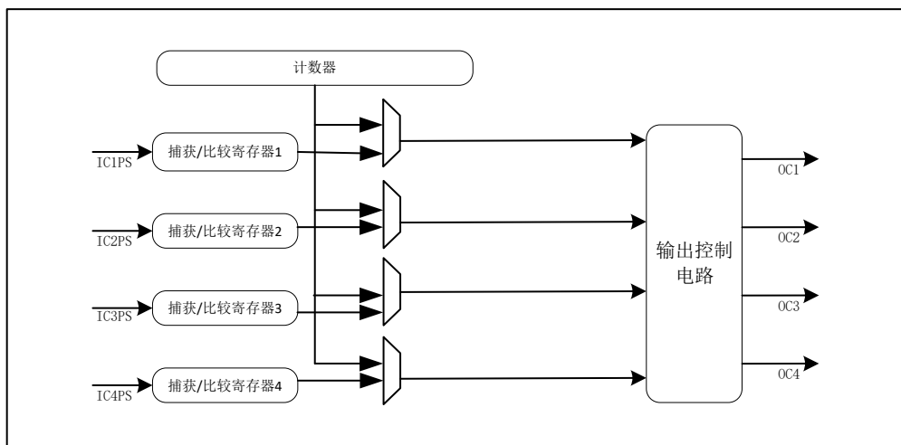
图 9-14 比较输出部分结构图
