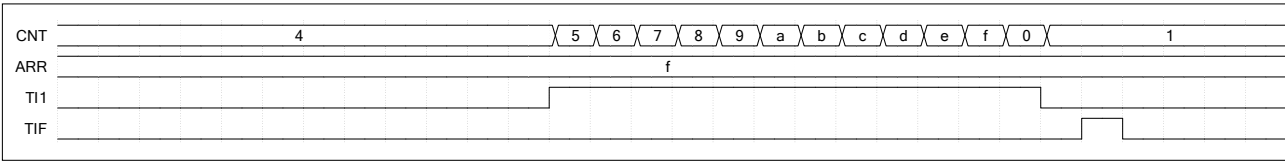
图 9-24 门控模式下的控制时序图
