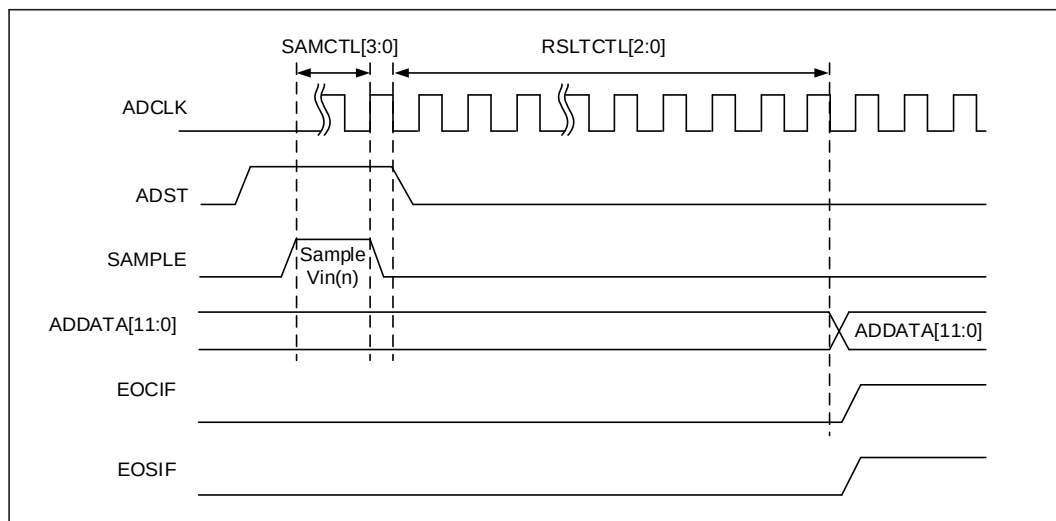
图 18-8 单次转换模式下通道转换时序图
