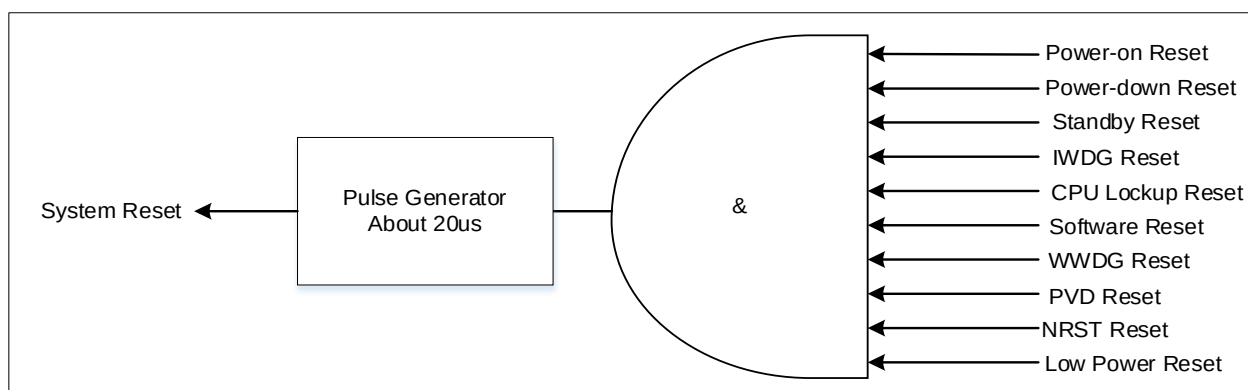
图 4-1 复位功能框图
