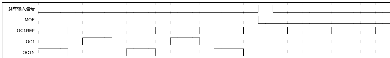
图 10-10 响应刹车的输出（OISx=0，OISxN=0）
