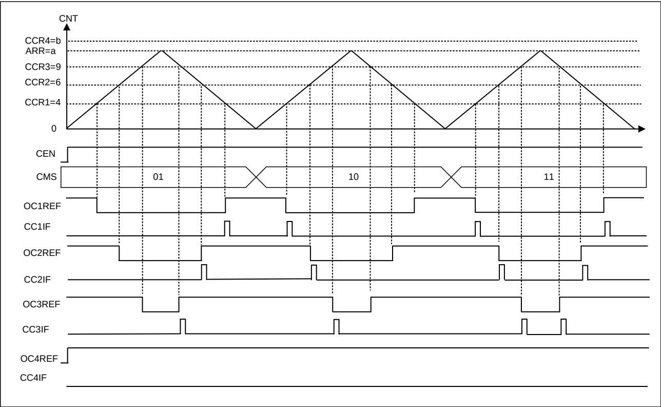
图 9-18 中央对齐 PWM 模式 1 的波形
