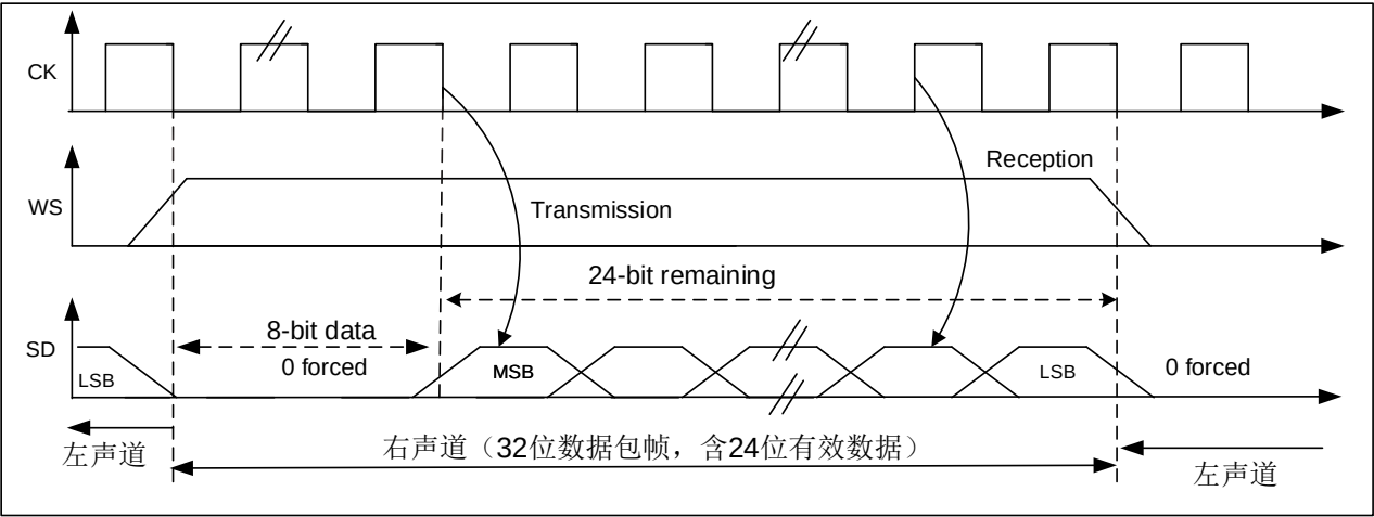
图 14-6 LSB 对齐标准示意图
