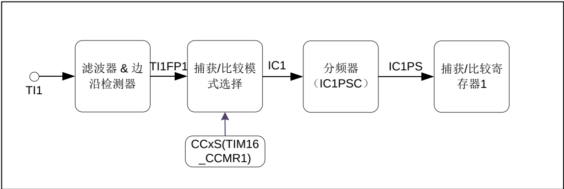
图 10-5 TIMx 输入捕获结构图
