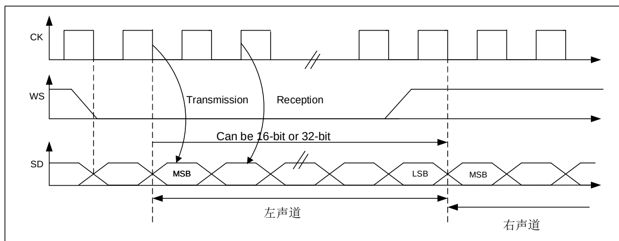
图 14-4 飞利浦标准示意图
