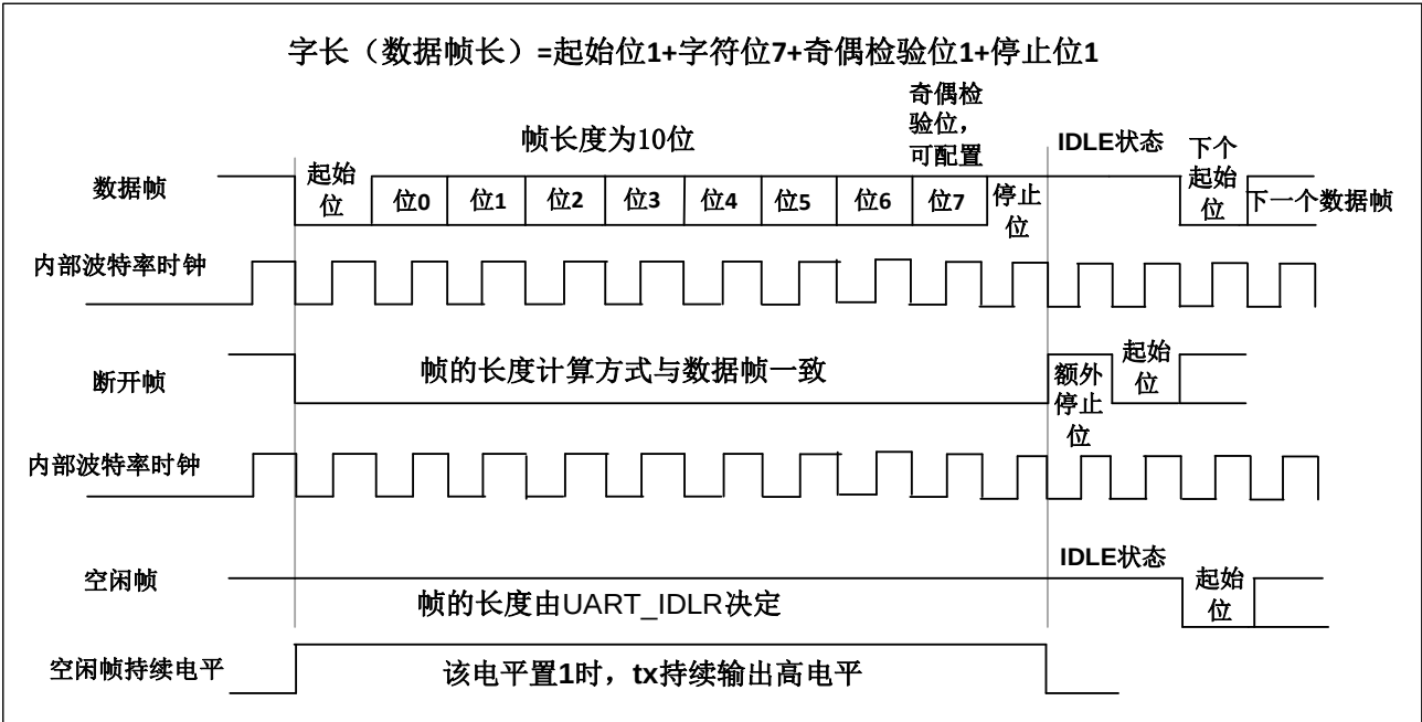
图 15-2 UART 时序
