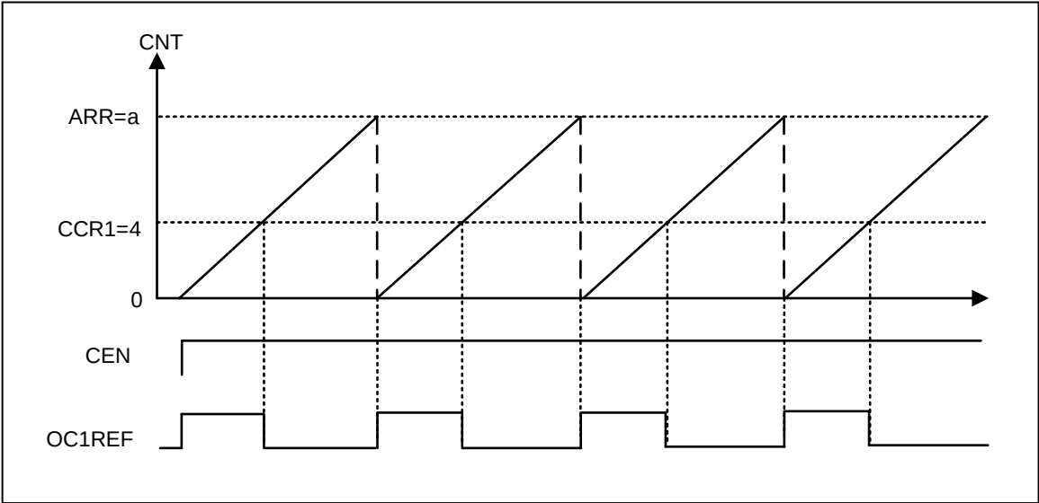
图 10-8 边沿对齐递增计数时 PWM 模式 1 的波形
