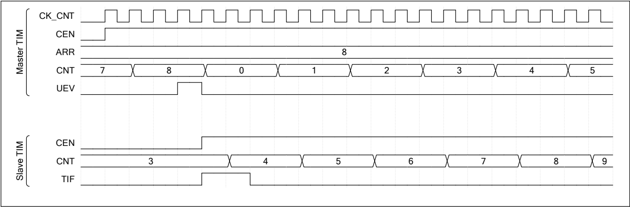
图 9-30 使用主定时器的更新事件启动从定时器
