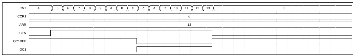
图 10-14 单脉冲模式
