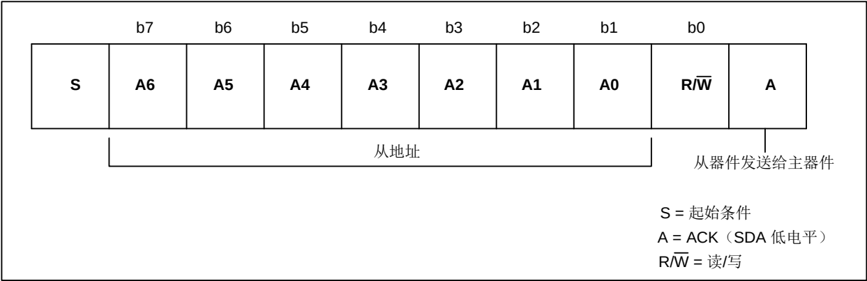
图 17-3 7 位地址格式
