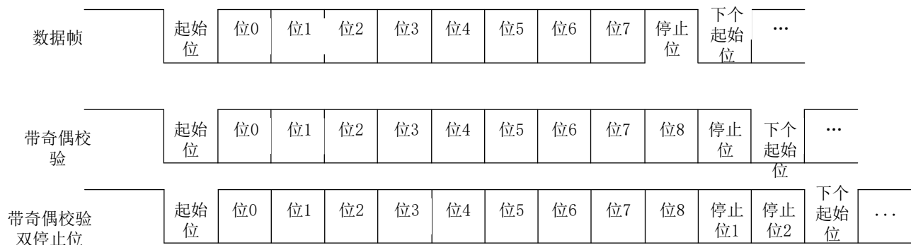
图 16-2 帧时序
