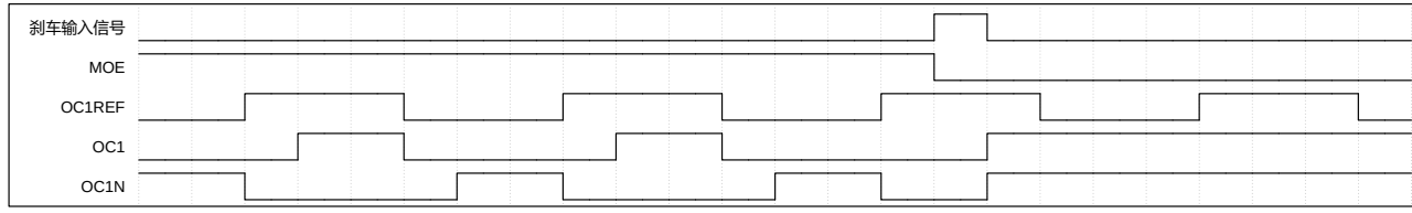
图 10-13 响应刹车的输出（OISx=1，OISxN=1）
