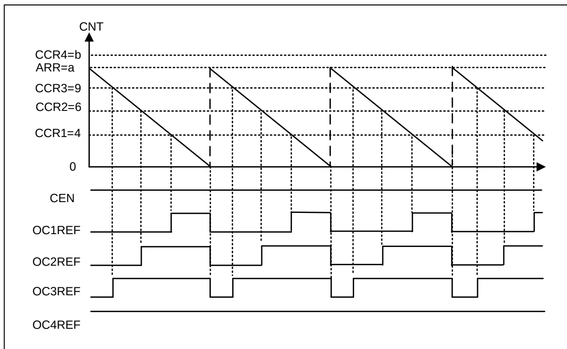
图 9-17 边沿对齐递减计数时 PWM 模式 1 的波形
