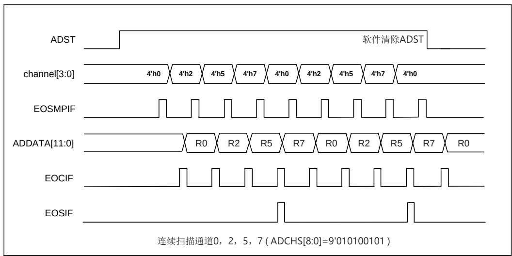
图 18-6 连续扫描模式使能通道转换时序图（通道方向由低到高）
