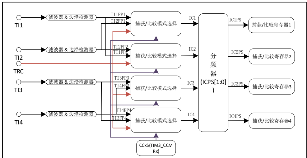
图 9-12 TIMx 输入捕获结构图
