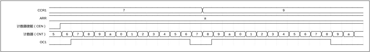
图 10-7 比较输出模式，OC1 信号在匹配时翻转
