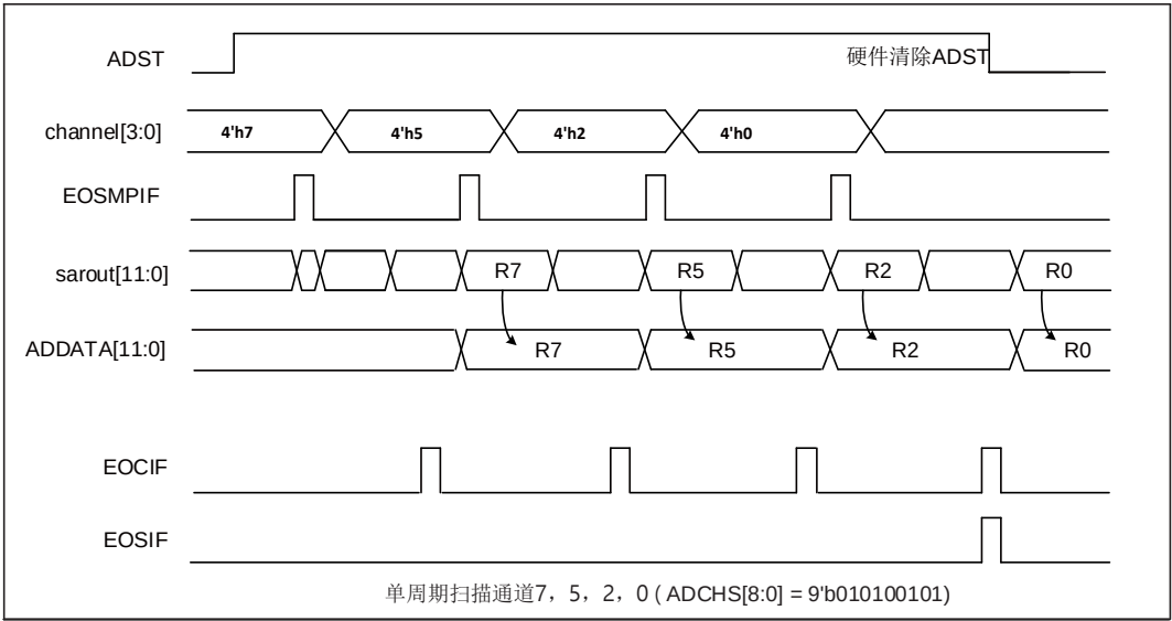
图 18-4 单周期扫描下使能通道转换时序图（通道方向从高到低）
