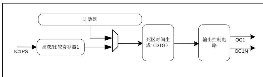
图 10-6 比较输出部分结构图
