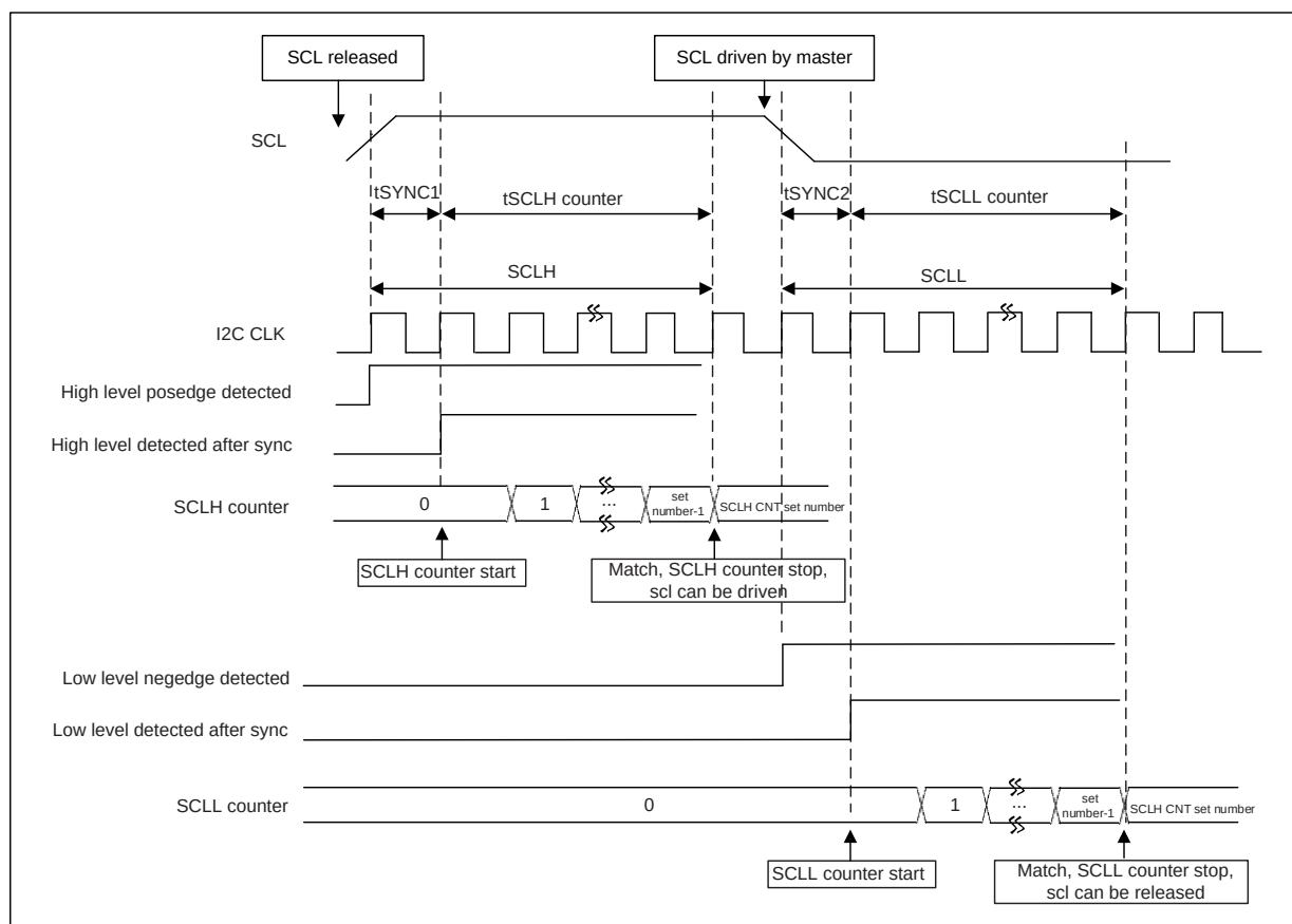
图 17-17 SCL 生成时序
