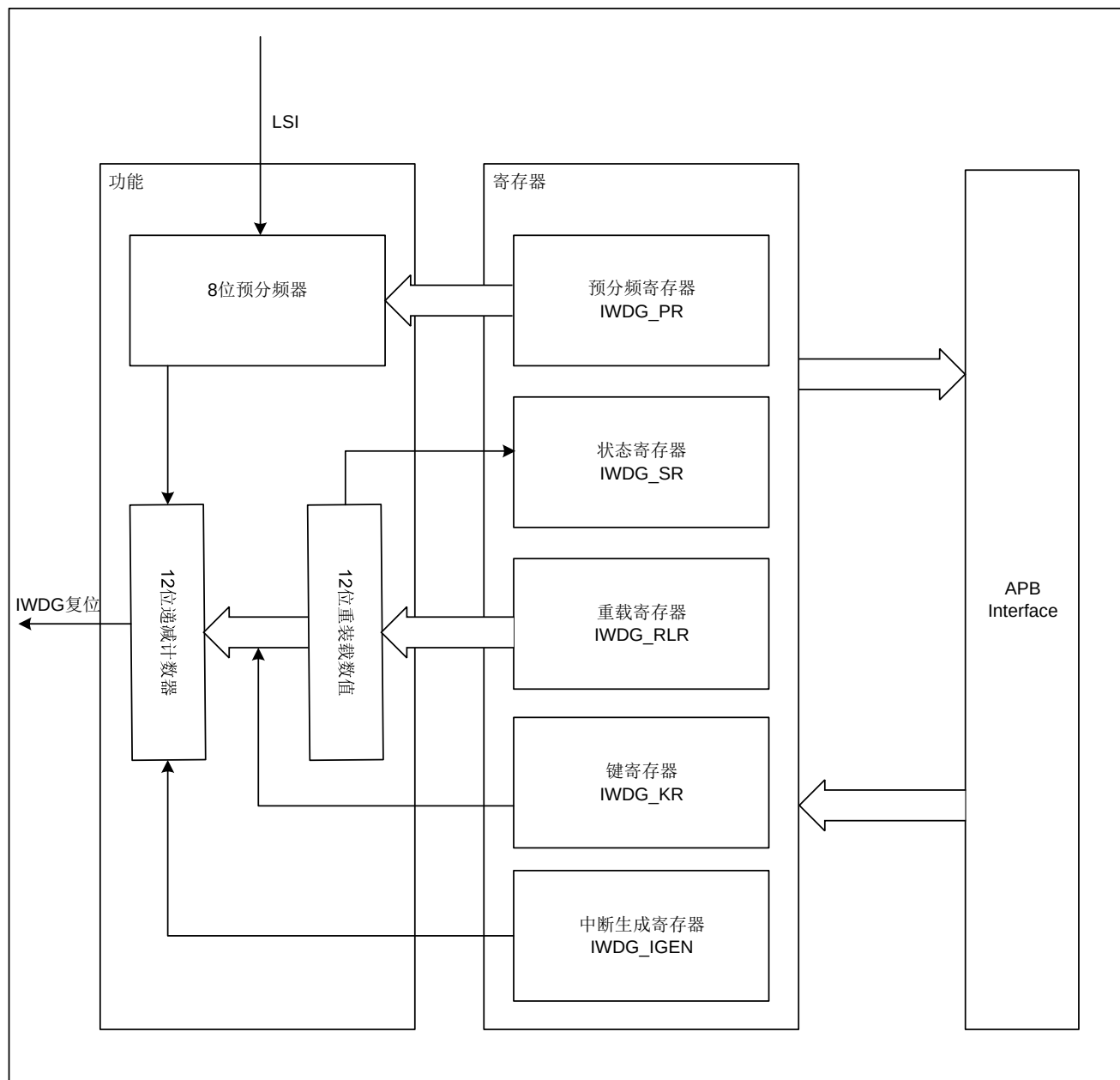
图 12-1 功能框图
