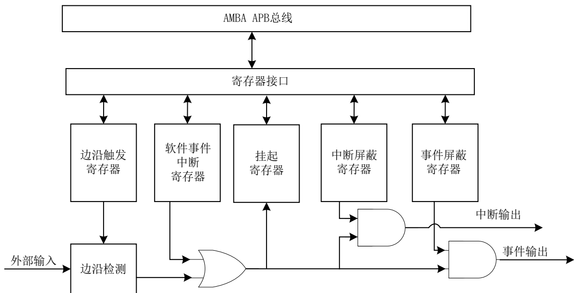
图 6-1 EXTI 结构框图
