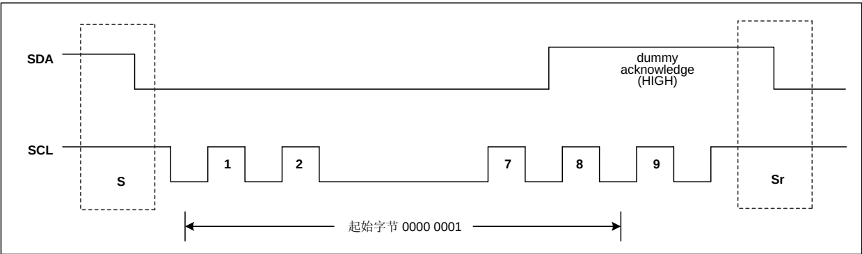
图 17-8 起始字节传输
