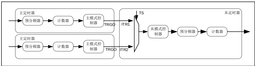
图 9-27 定时器间互联
