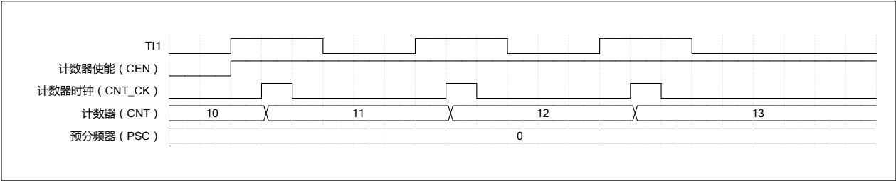
图 9-3 外部时钟模式 1 下的控制电路
