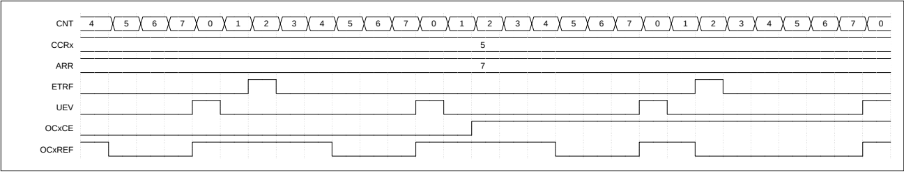
图 9-19 外部事件清除 OCxREF
