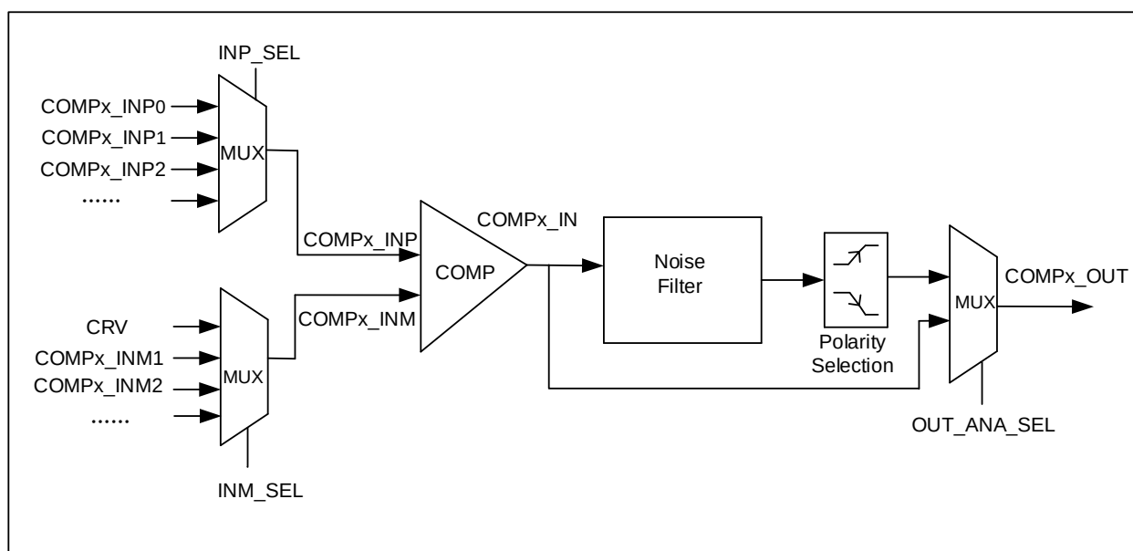
图 19-1 比较器框图
