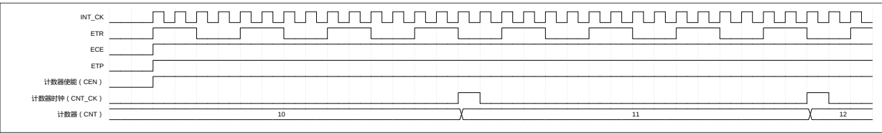
图 9-4 外部时钟模式 2 下的控制电路
