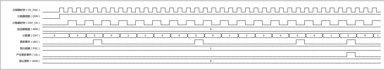
图 10-3 递增计数模式（UDIS=0）
