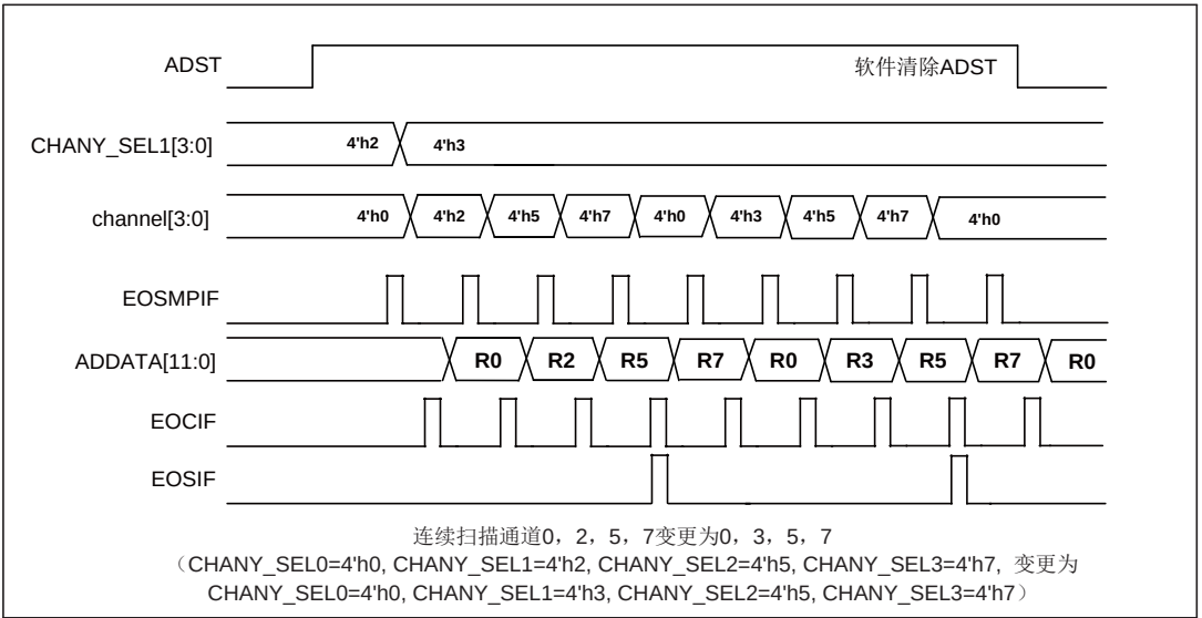
图 18-11 连续扫描模式下动态更新配置时序图
