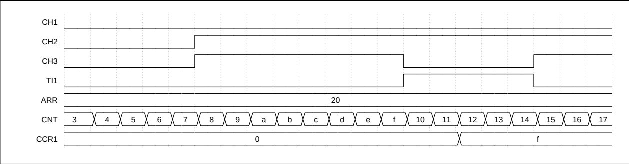
图 9-32 （TI1 异或输入）输入捕获波形图
