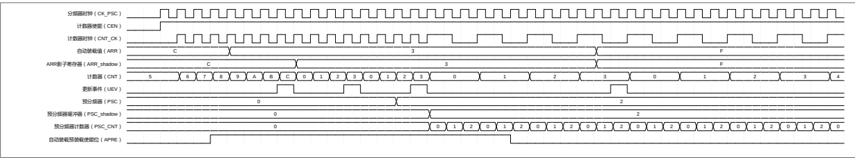
图 10-2 自动预装载
