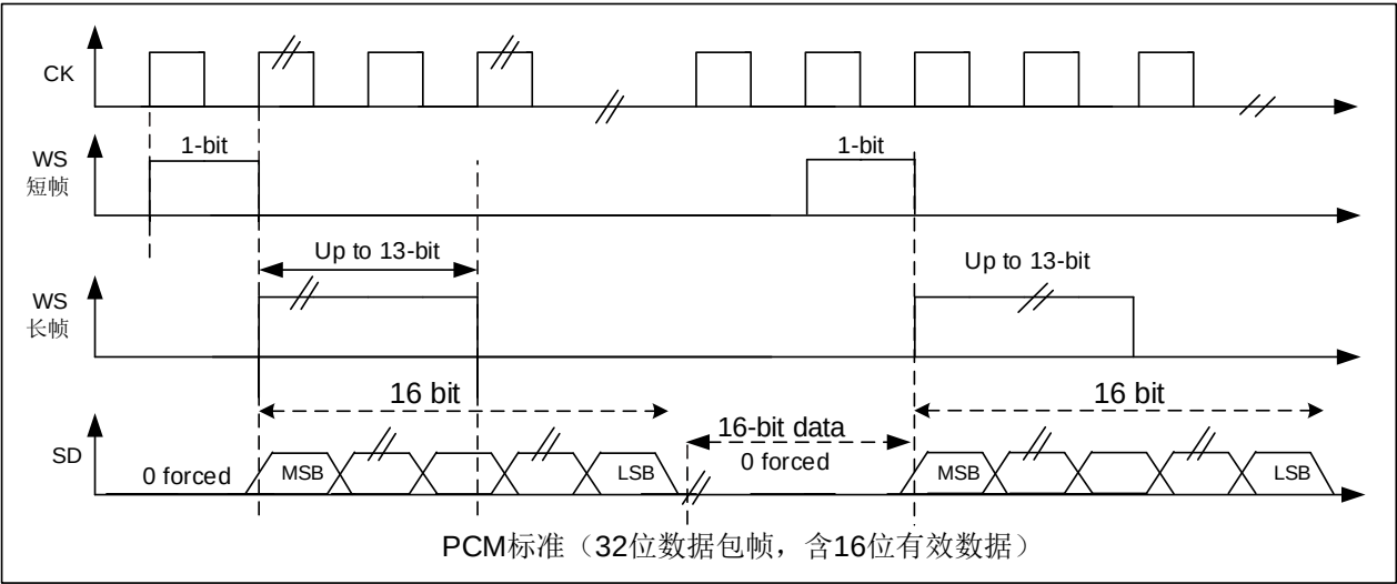
图 14-7 PCM 标准示意图
