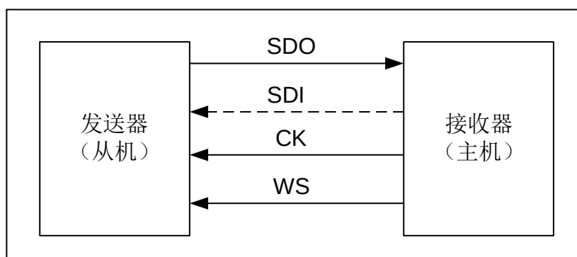
图 14-8 I2S 从模式（SD 配置成 SDO 为发送器，配置成 SDI 为接收器）
