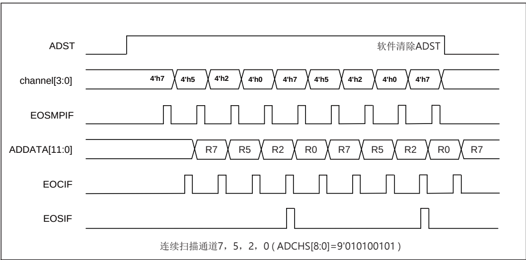
图 18-7 连续扫描模式使能通道转换时序图（通道方向由高到低）
