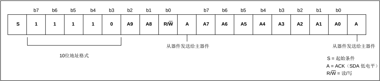
图 17-4 10 位地址格式
