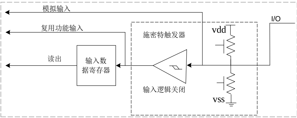
图 8-5 模拟输入
