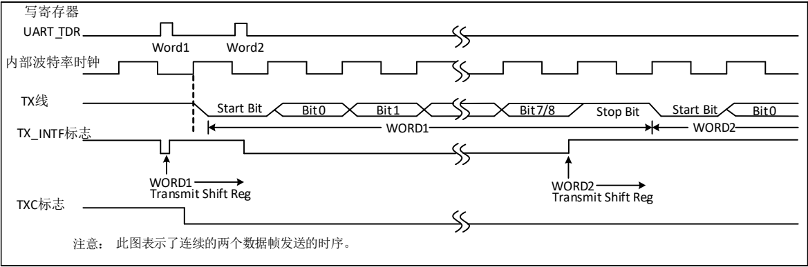
图 15-4 发送时状态位变化
