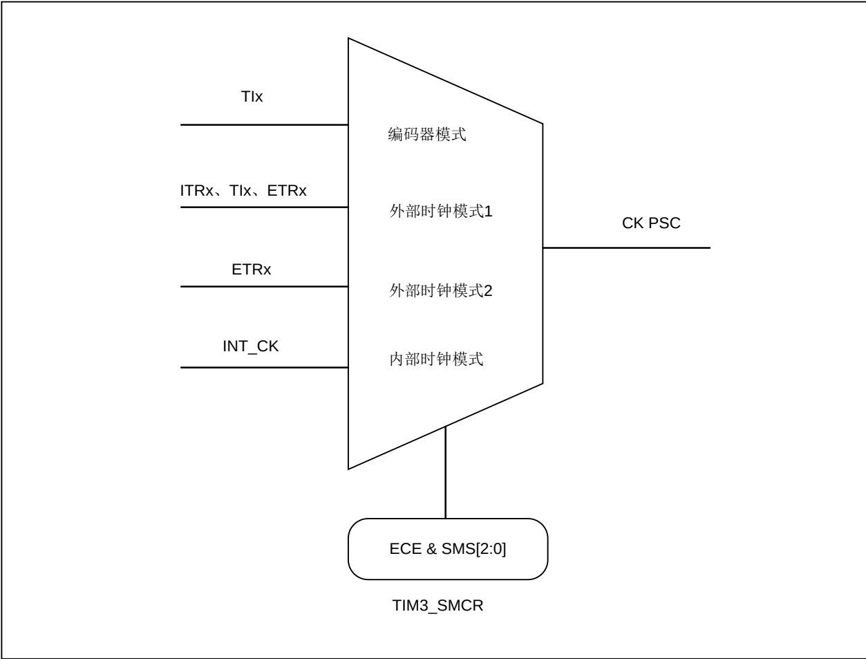
图 9-2 时钟选择
