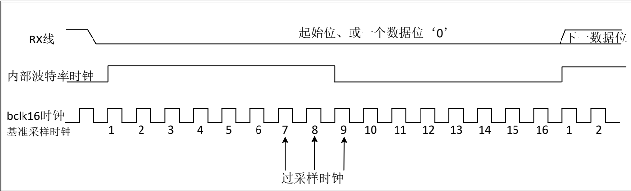
图 15-3 RX 引脚采样方法
