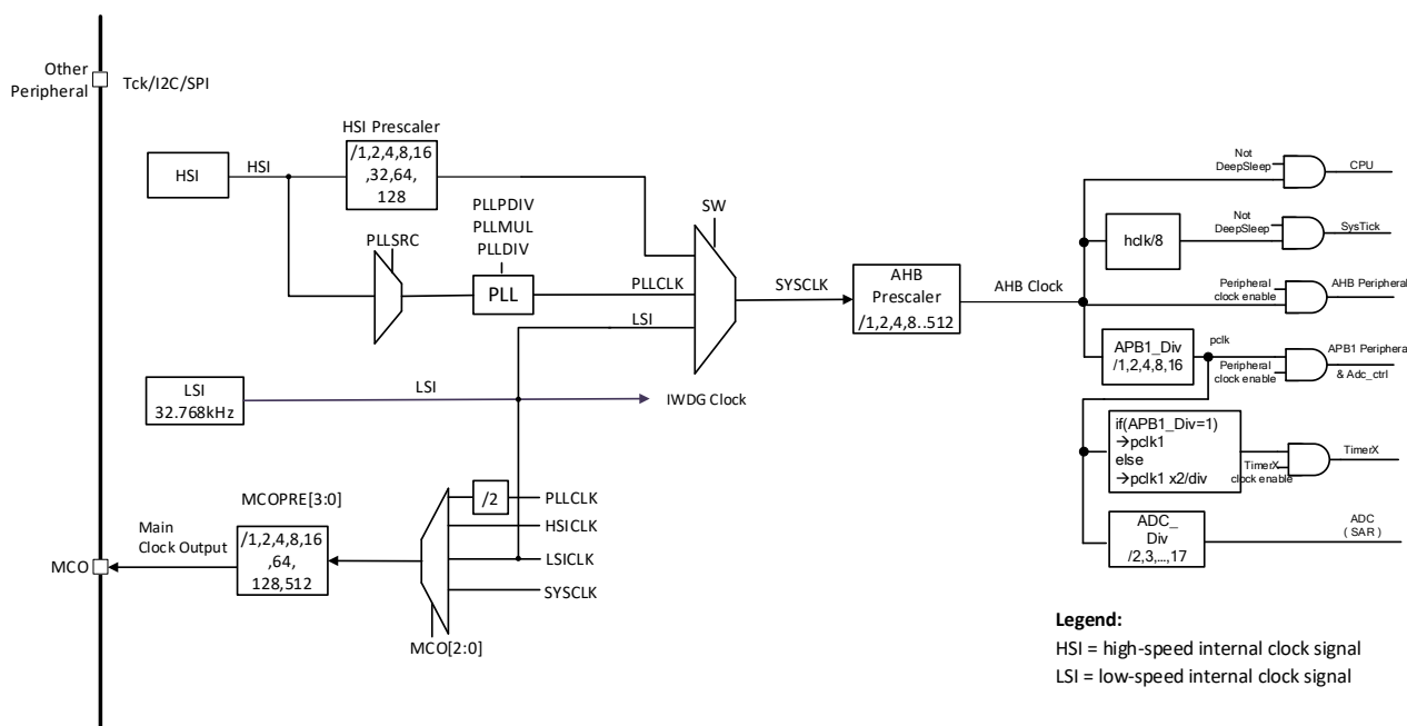
图 4-2 时钟树
