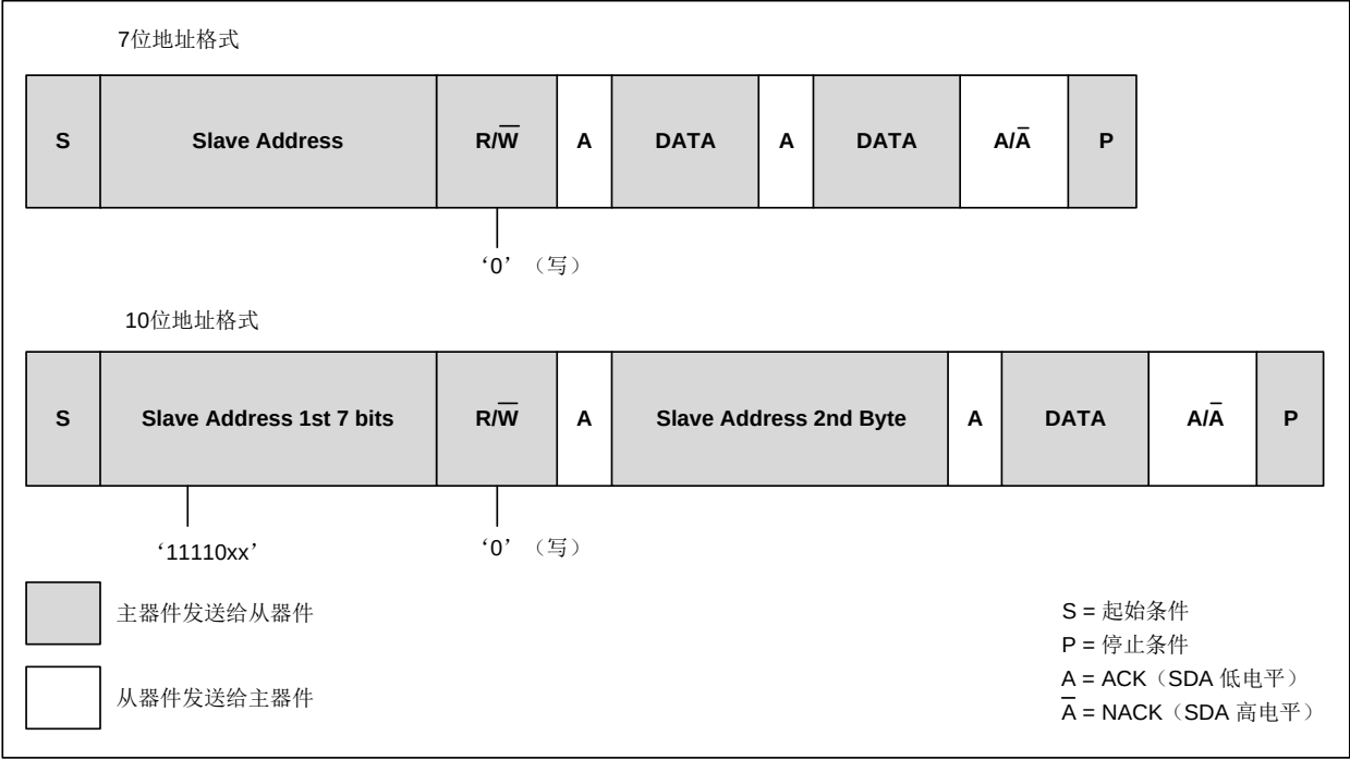
图 17-5 主发送协议
