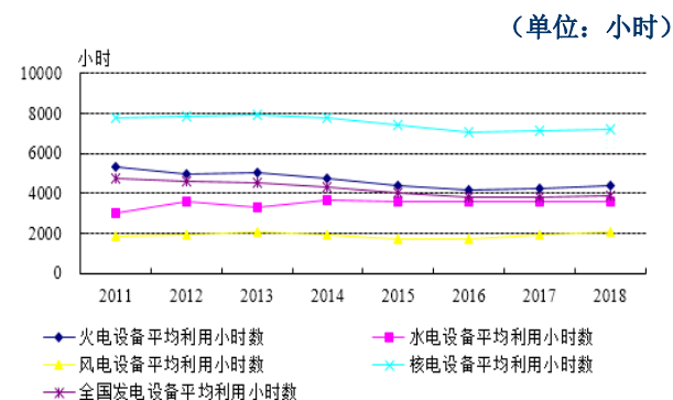
图3：2011年以来全国电力设备利用小时数情况
