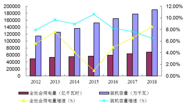
图2：2012年以来我国电力消费与发电装机增长情况
