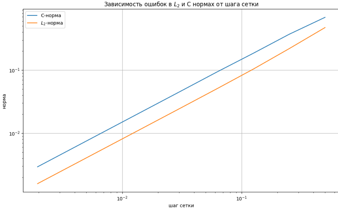
Рис. 1: Зависимость С-нормы и дискретной L2-нормы ошибки решения от шага сетки h = \frac{1}{N}
