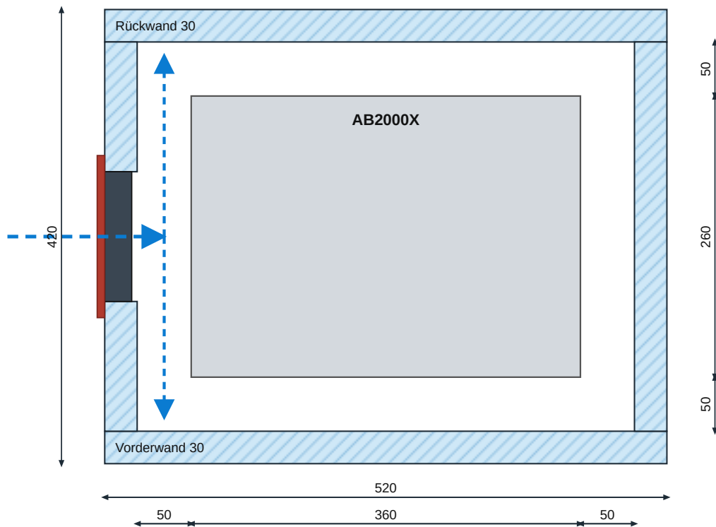
SCHNITT C-C auf Höhe z = 110 mm (unterste AB2000X, Zuluft-Lüfter)
