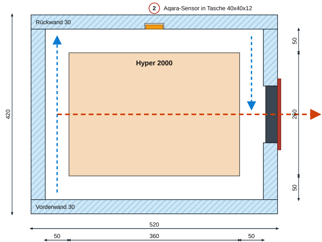
SCHNITT B-B auf Höhe z = 780 mm (Hyper, Abluft-Lüfter, Sensor)
