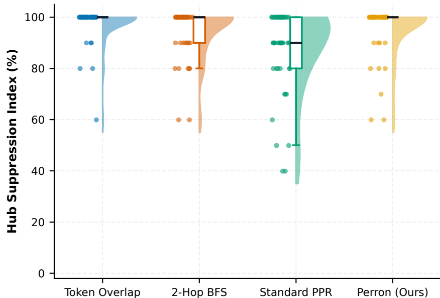
(a) Hub Suppression Distribution (Raincloud)
