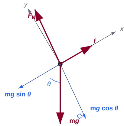
자유물체도 (FBD)
