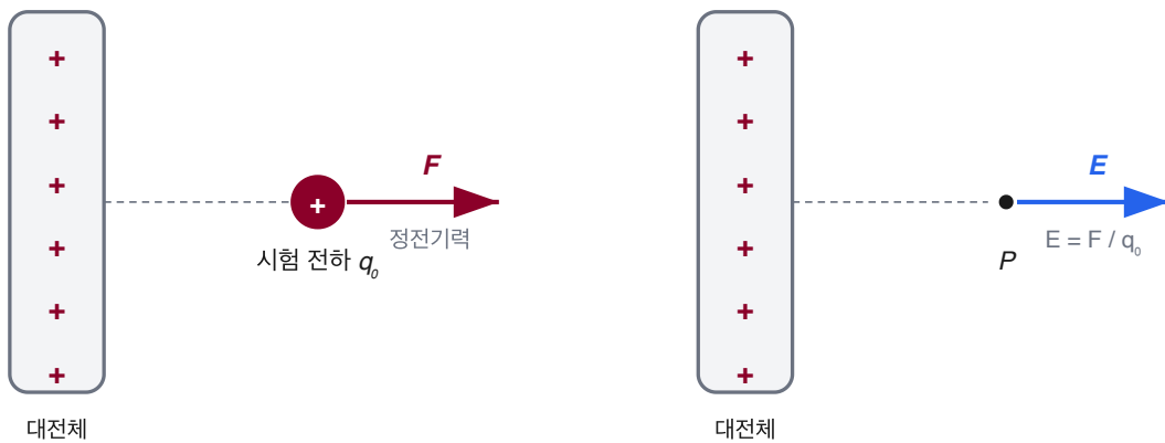
(a) 시험 전하 q_0 가 받는 힘
