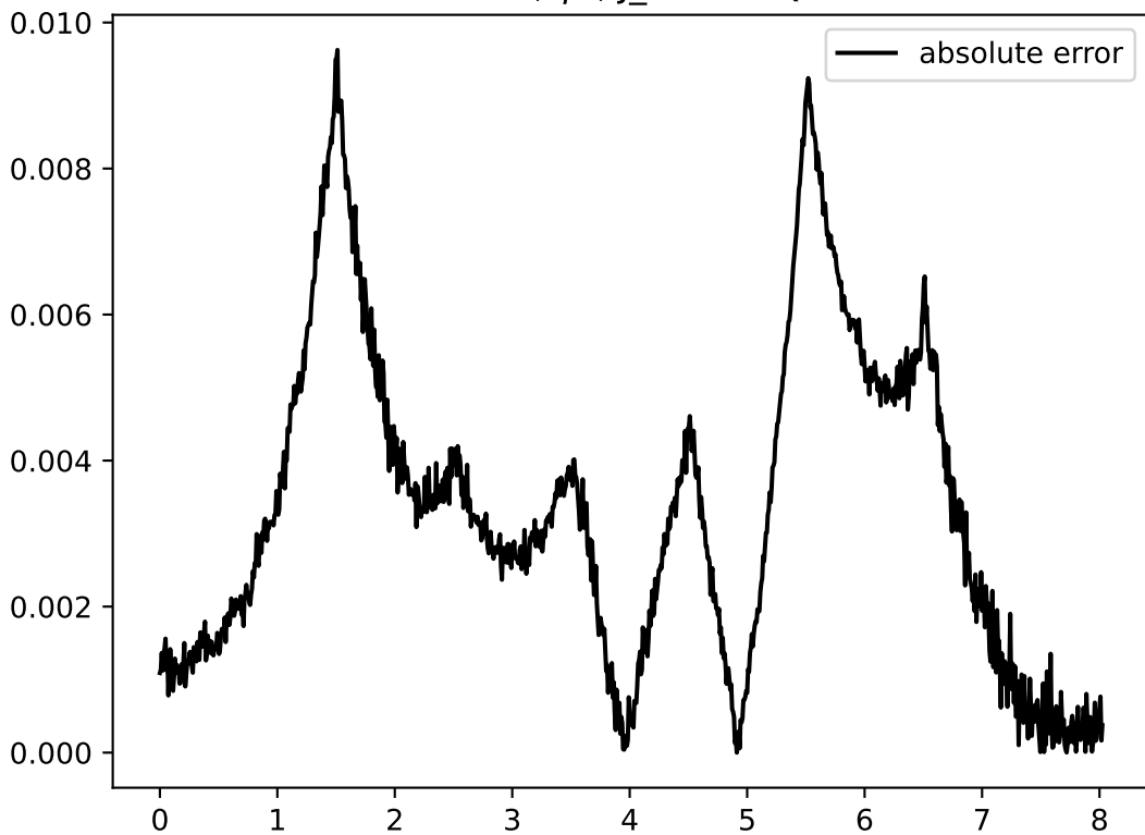
RFM error, \psi^2 , J_n=200 Q=200
