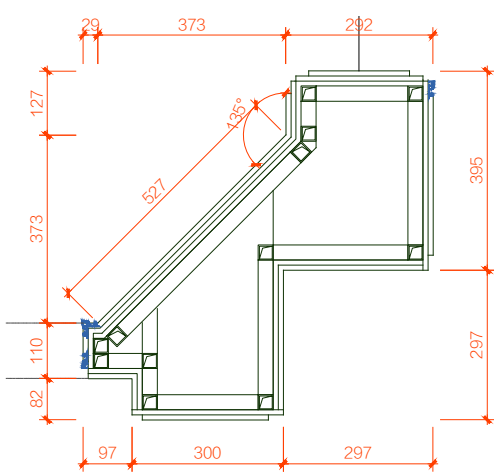
02 — 大样图 SCALE 1: 15
