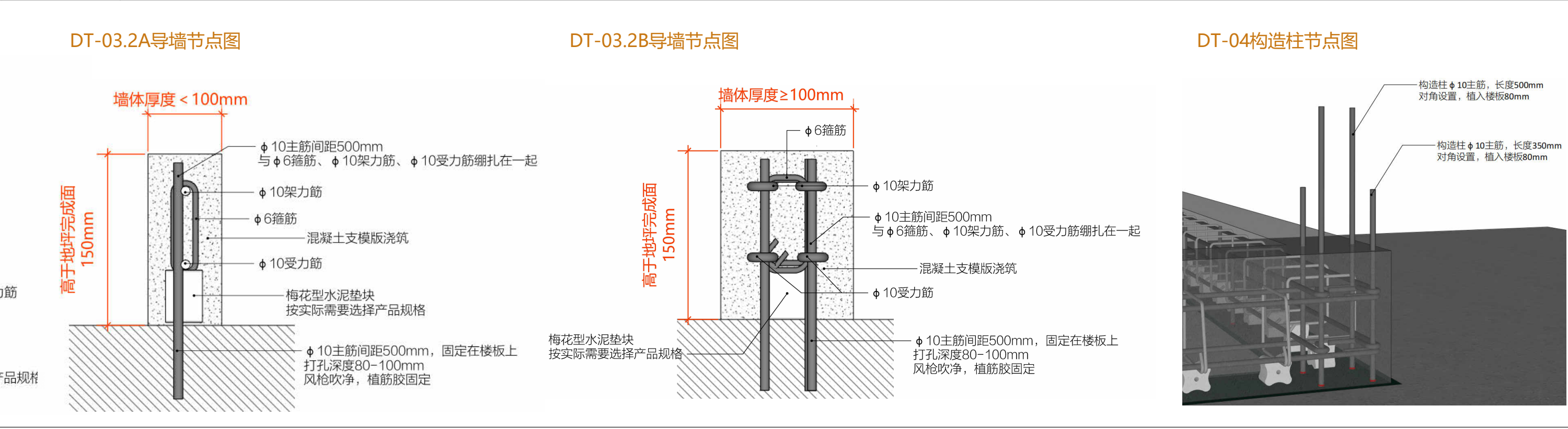
2 客厅-02 1F客厅混凝土导墙、构造柱钢筋立面图2 Scale比例 1:20@A2
