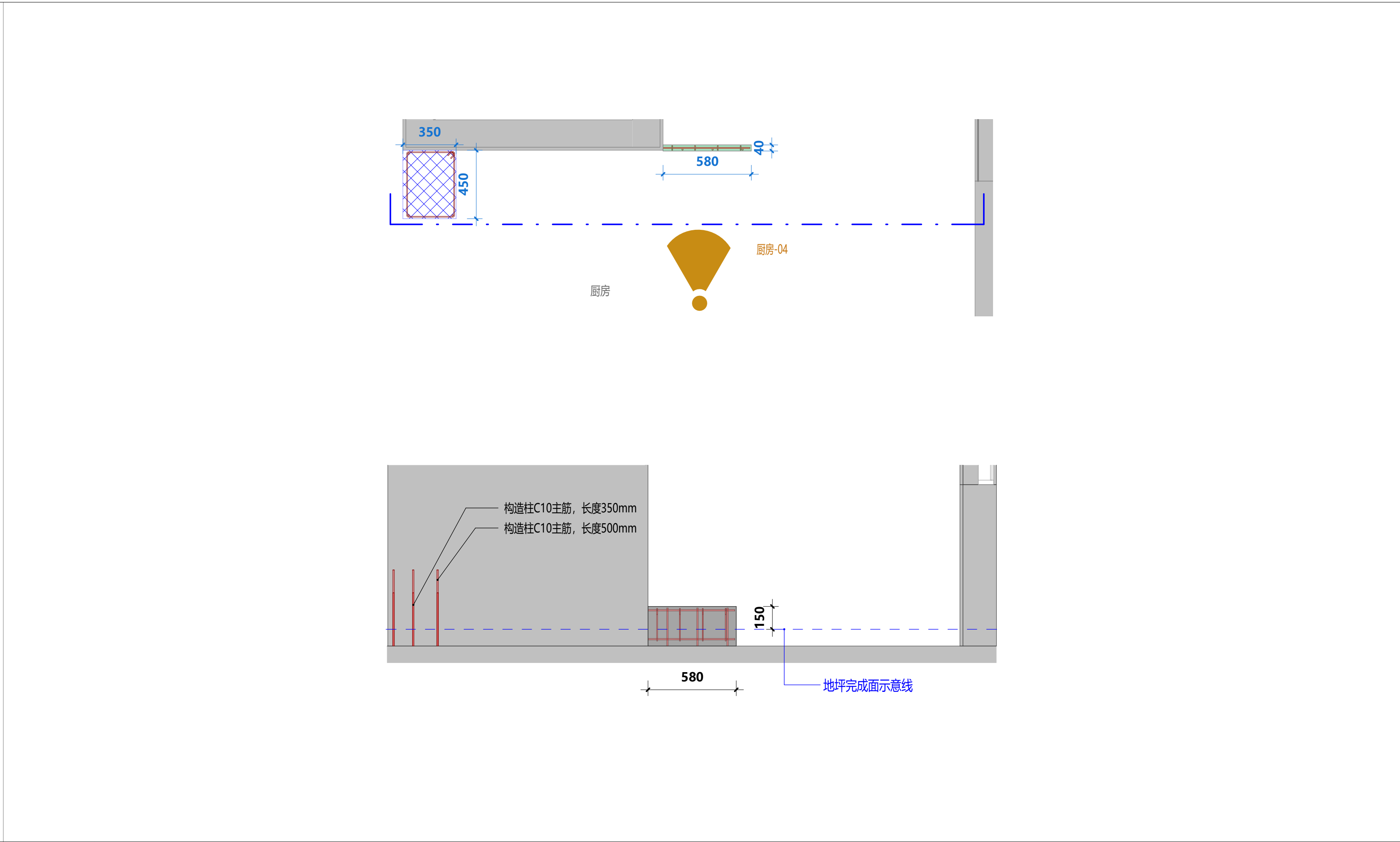
2 1F厨房混凝土导墙、构造柱钢筋立面图4 厨房-04 Scale比例 1:20@A2
