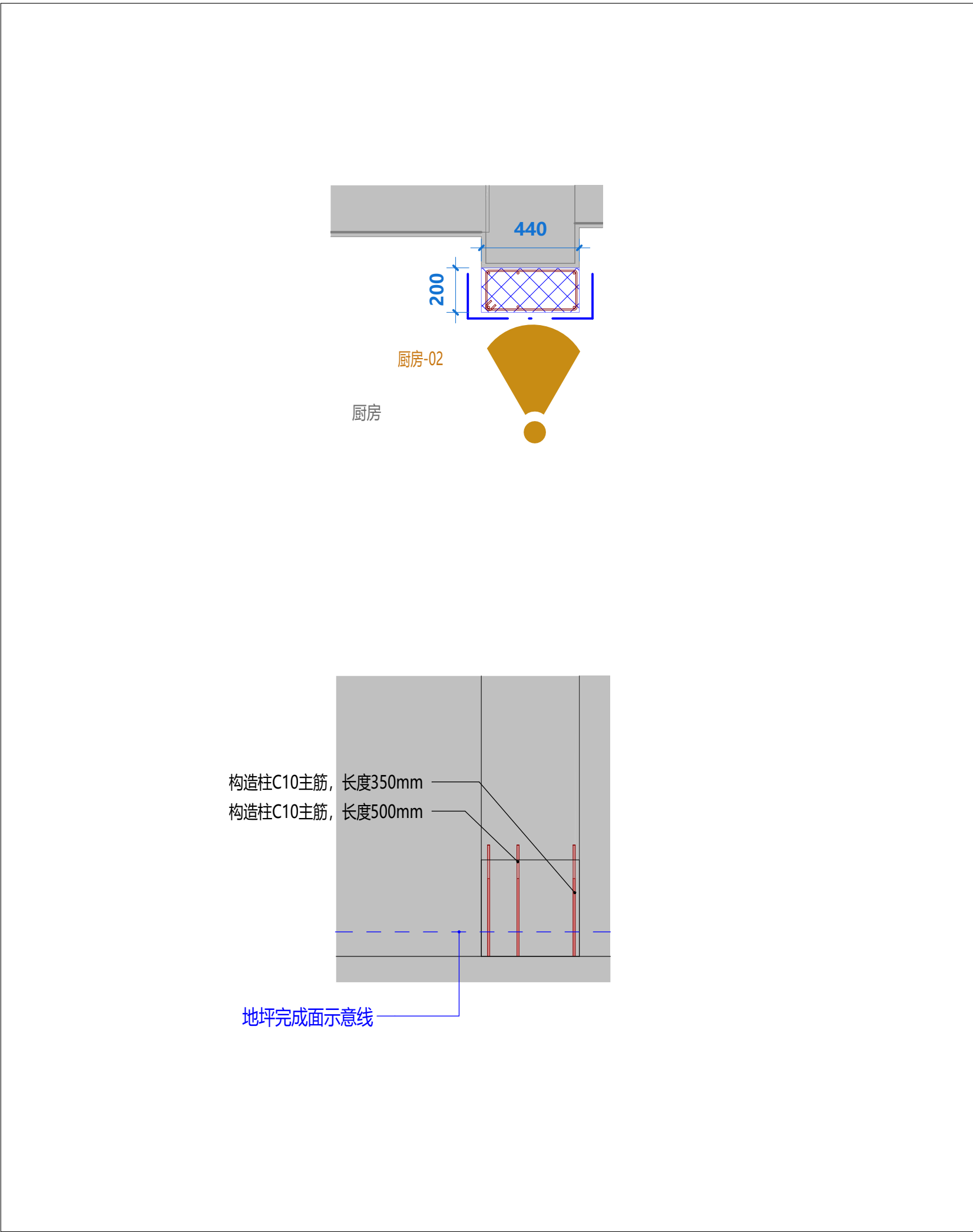
1 1F厨房混凝土导墙、构造柱钢筋立面图2 厨房-02 Scale比例 1:20@A2
