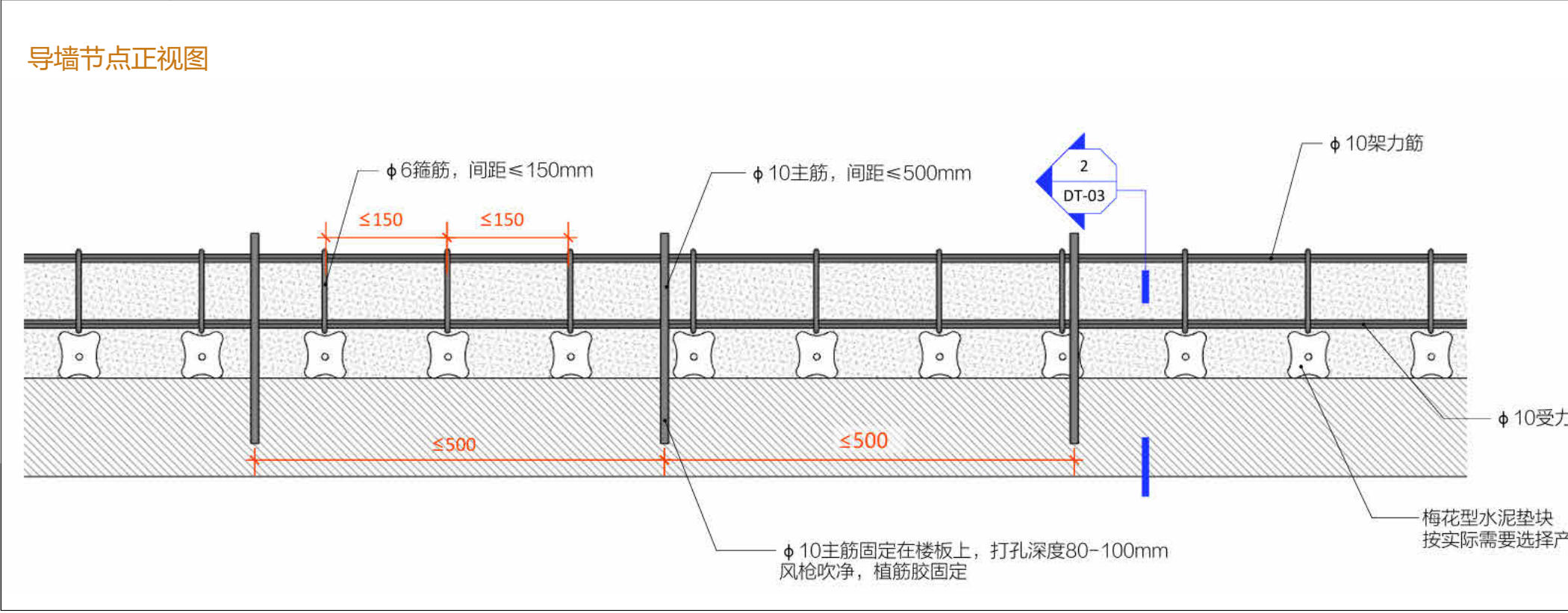
1 客厅-01 1F客厅混凝土导墙、构造柱钢筋立面图1 Scale比例 1:20@A2
