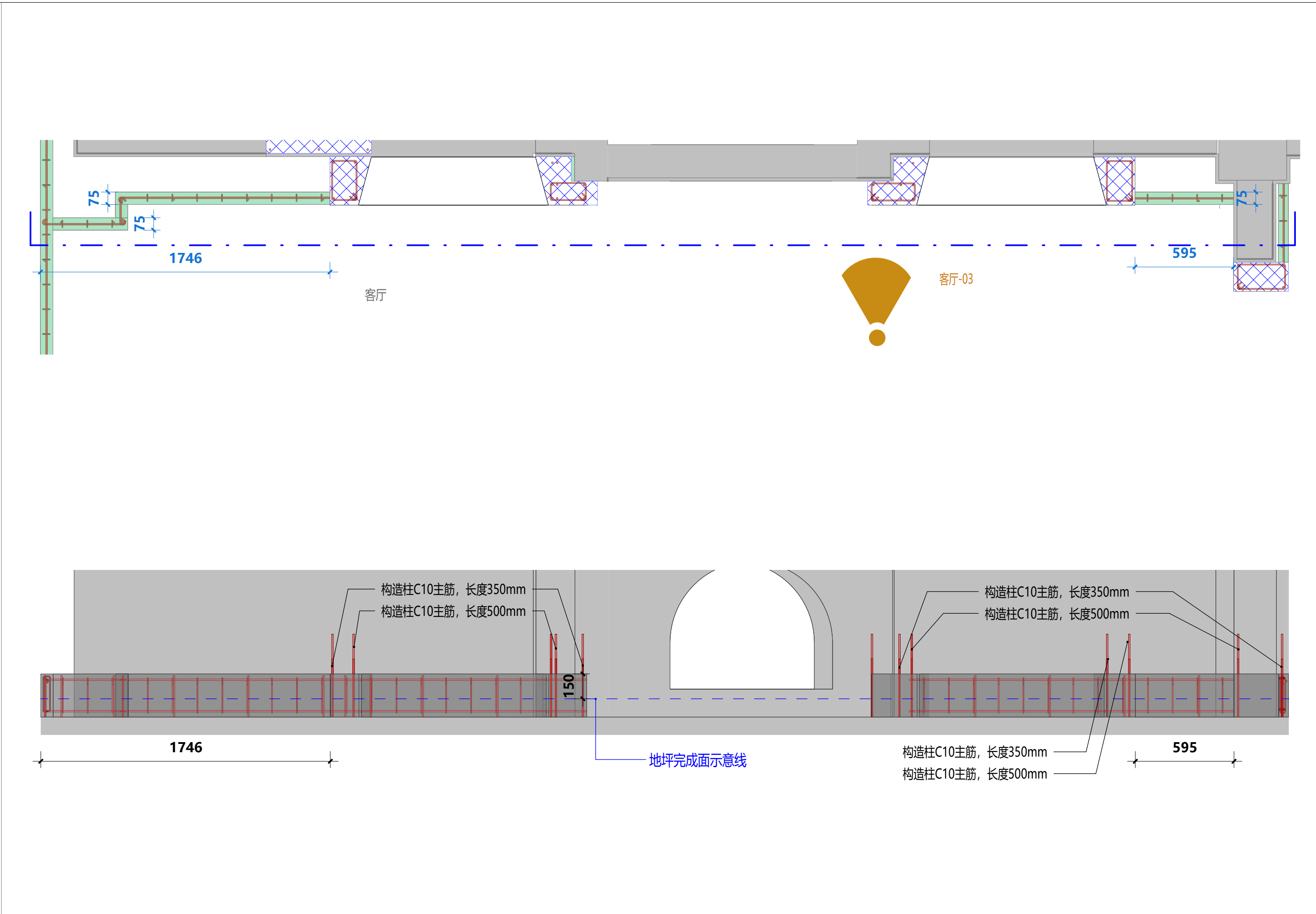
2 客厅-02 1F客厅混凝土导墙、构造柱钢筋立面图2 Scale比例 1:20@A2
