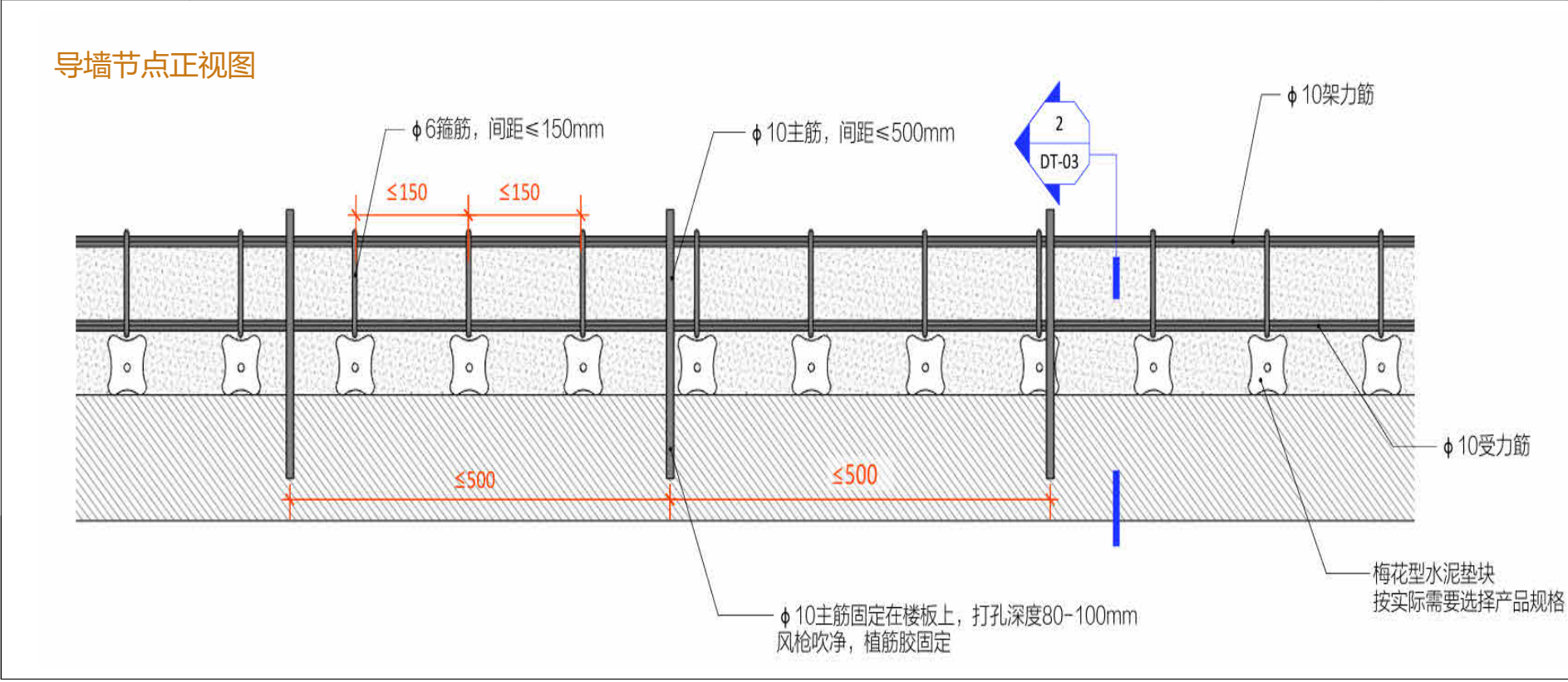
1 1F厨房混凝土导墙、构造柱钢筋立面图2 厨房-02 Scale比例 1:20@A2
