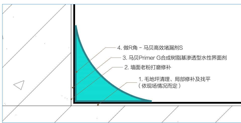
B 墙根防水节点图 Scale比例 1:2 @A2
