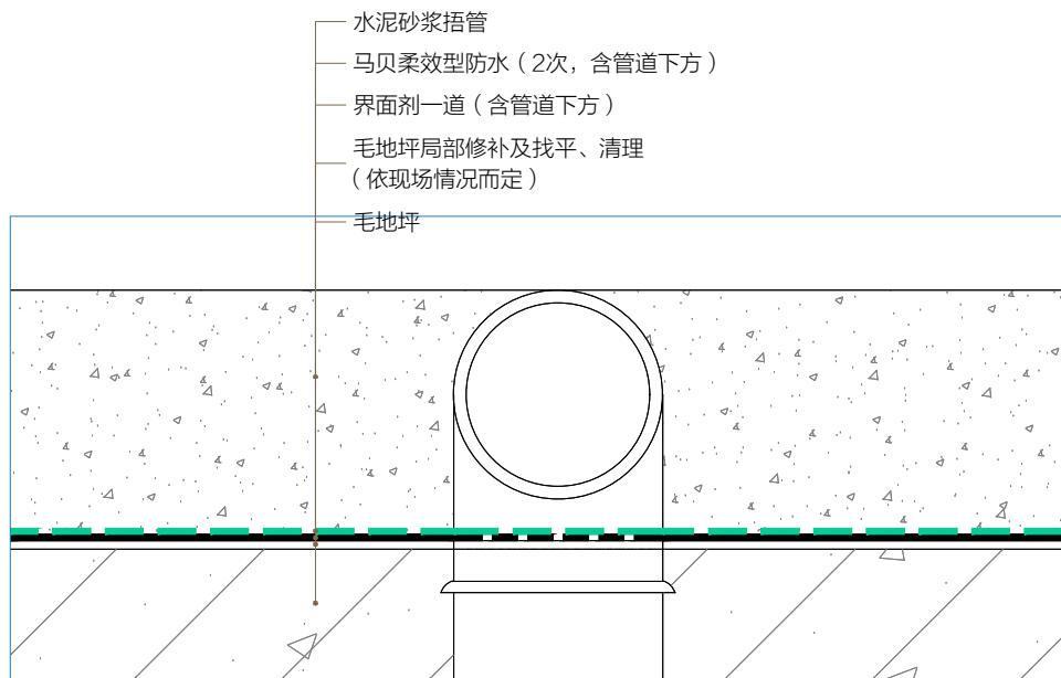
C 地面管道 插管防水节点图 Scale比例 1:2 @A2
