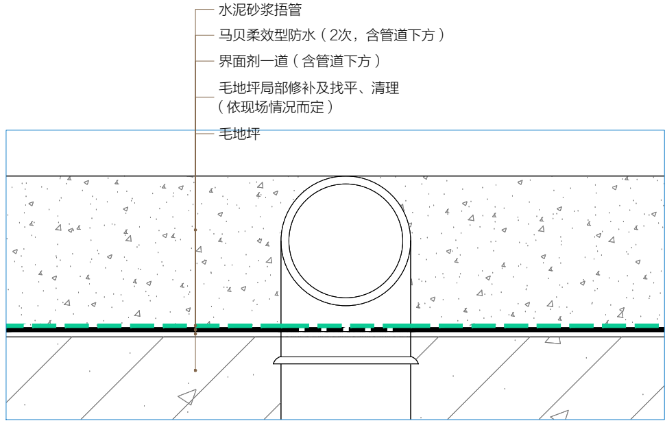
C 地面管道 捂管防水节点图 Scale比例 1:2 @A2
