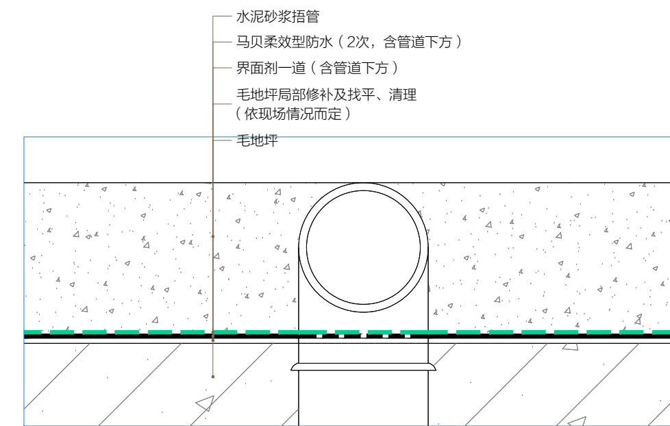
C 地面管道 堵管防水节点图 Scale比例 1:2 @A2
