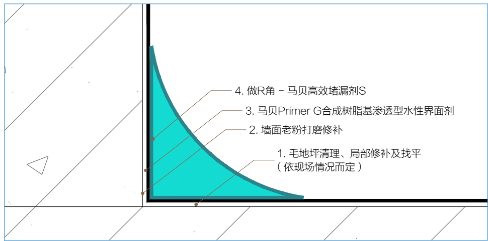
B 墙根防水节点图 Scale比例 1:2 @A2
