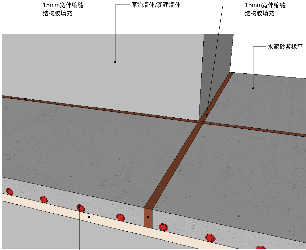
阳角伸缩缝剖面3D示意图
