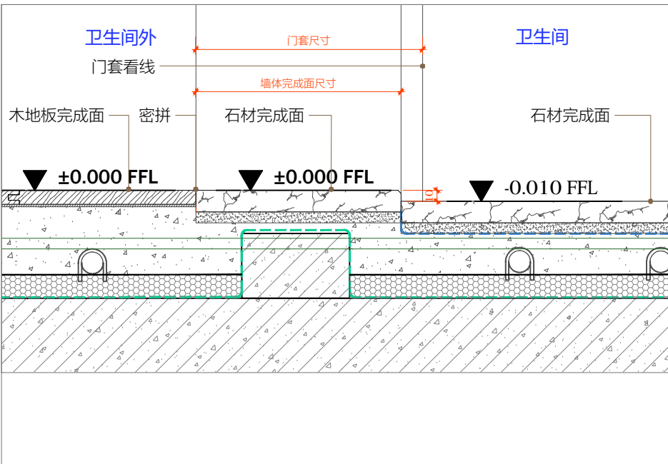
D 卫生间门槛大样 Scale比例 1:5 @A2
