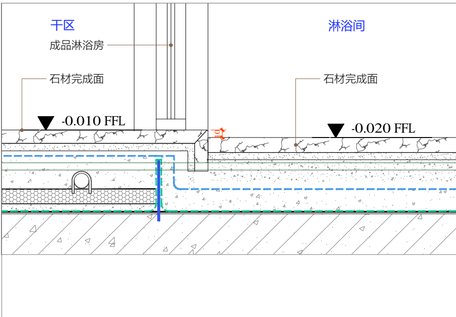
E 淋浴间大样 Scale比例 1:5 @A2
