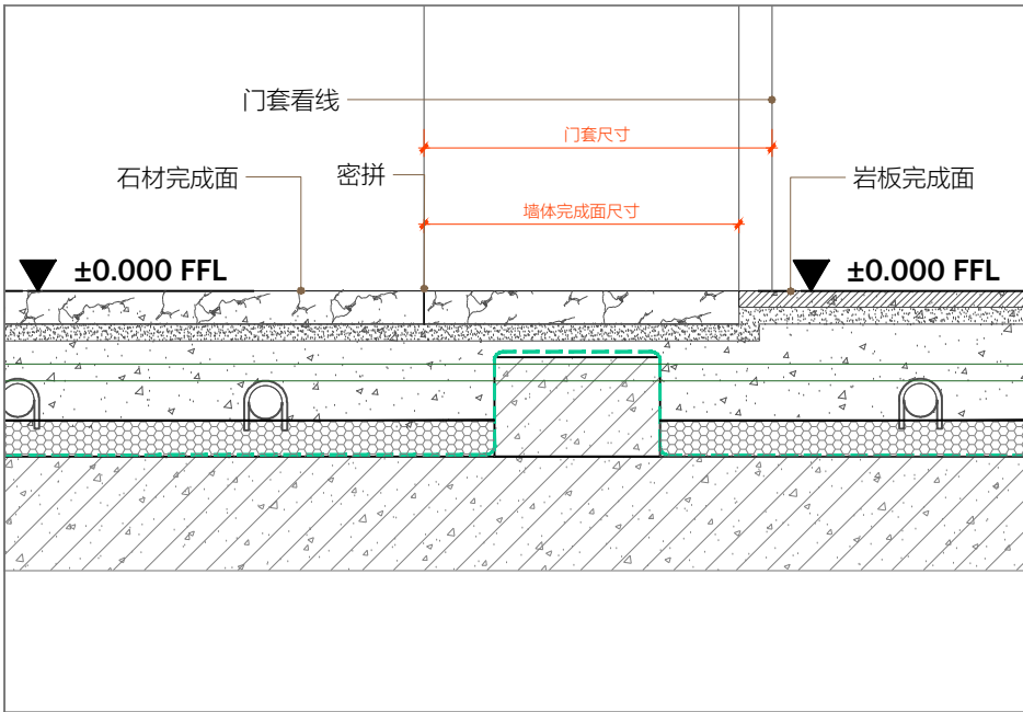
B 石材和岩板收口大样 Scale比例 1:5 @A2
