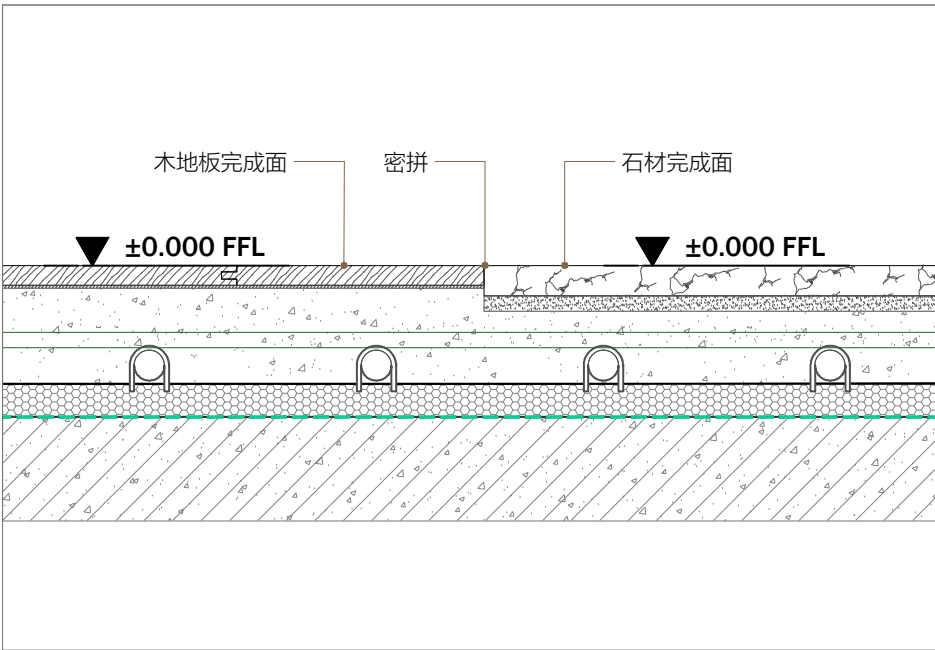
A 石材和木地板收口大样 Scale比例 1:5 @A2
