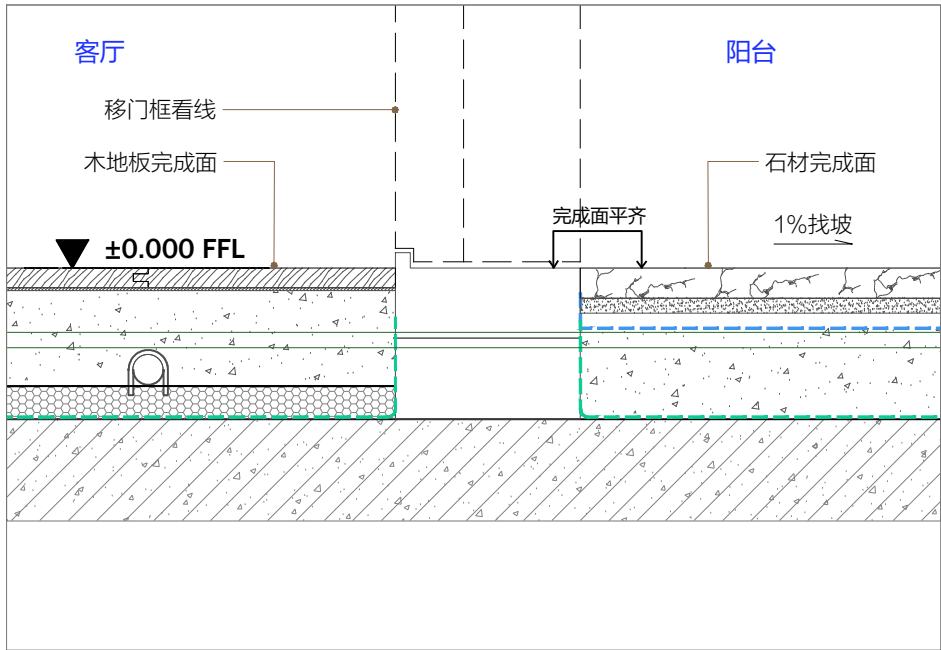
C 阳台门槛大样 Scale比例 1:5 @A2
