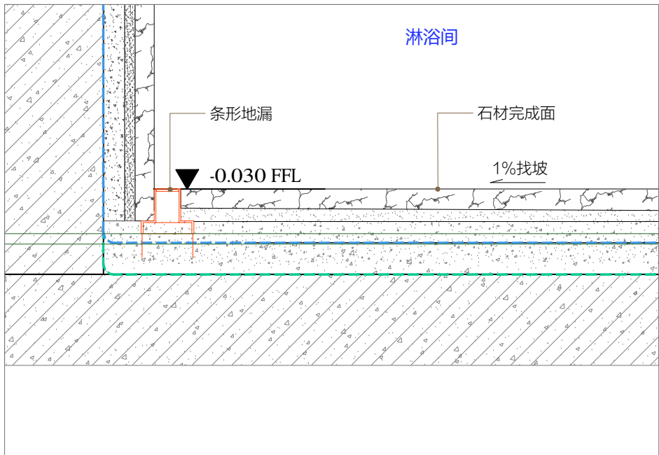
F 淋浴间地漏大样 Scale比例 1:5 @A2
