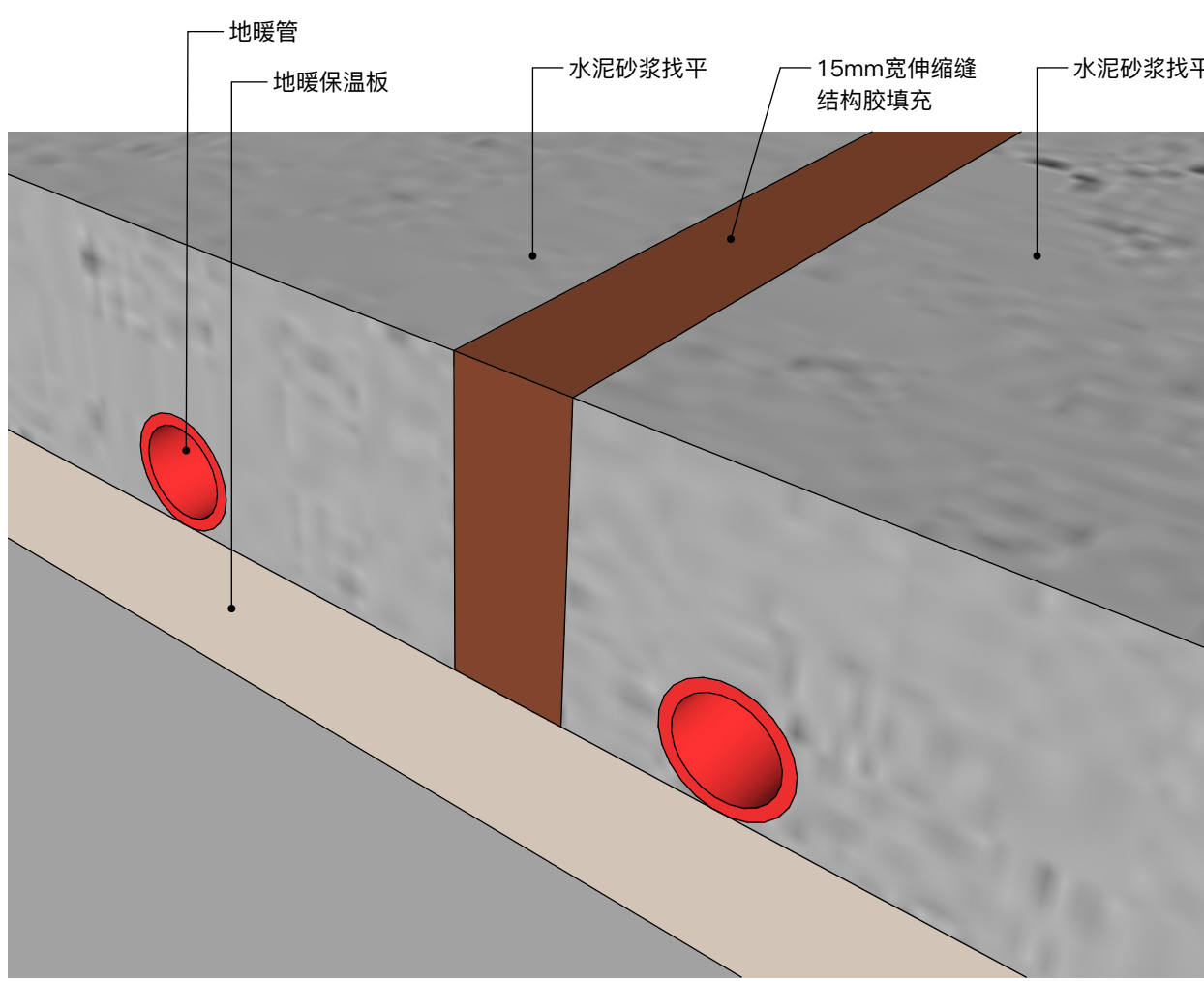
伸缩缝剖面3D示意图
