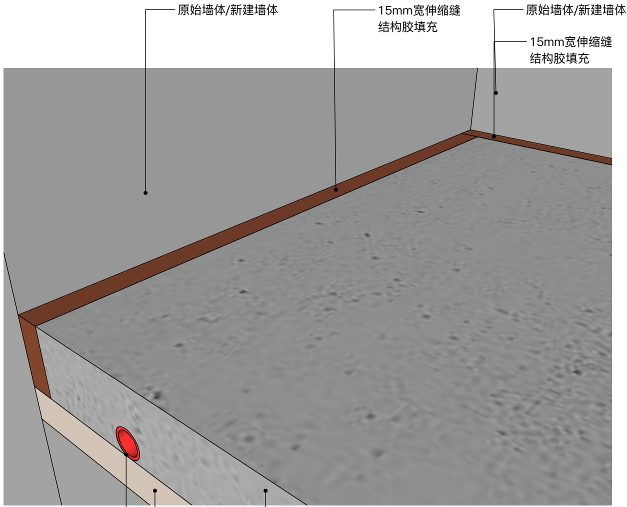
阴角伸缩缝剖面3D示意图
