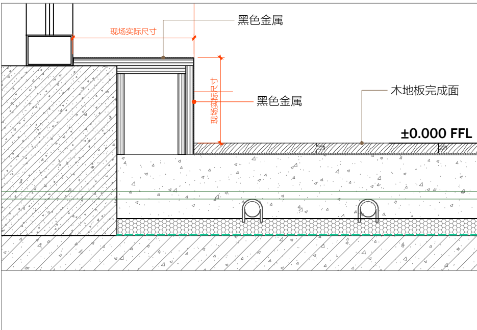
G 落地窗台大样 Scale比例 1:5 @A2
