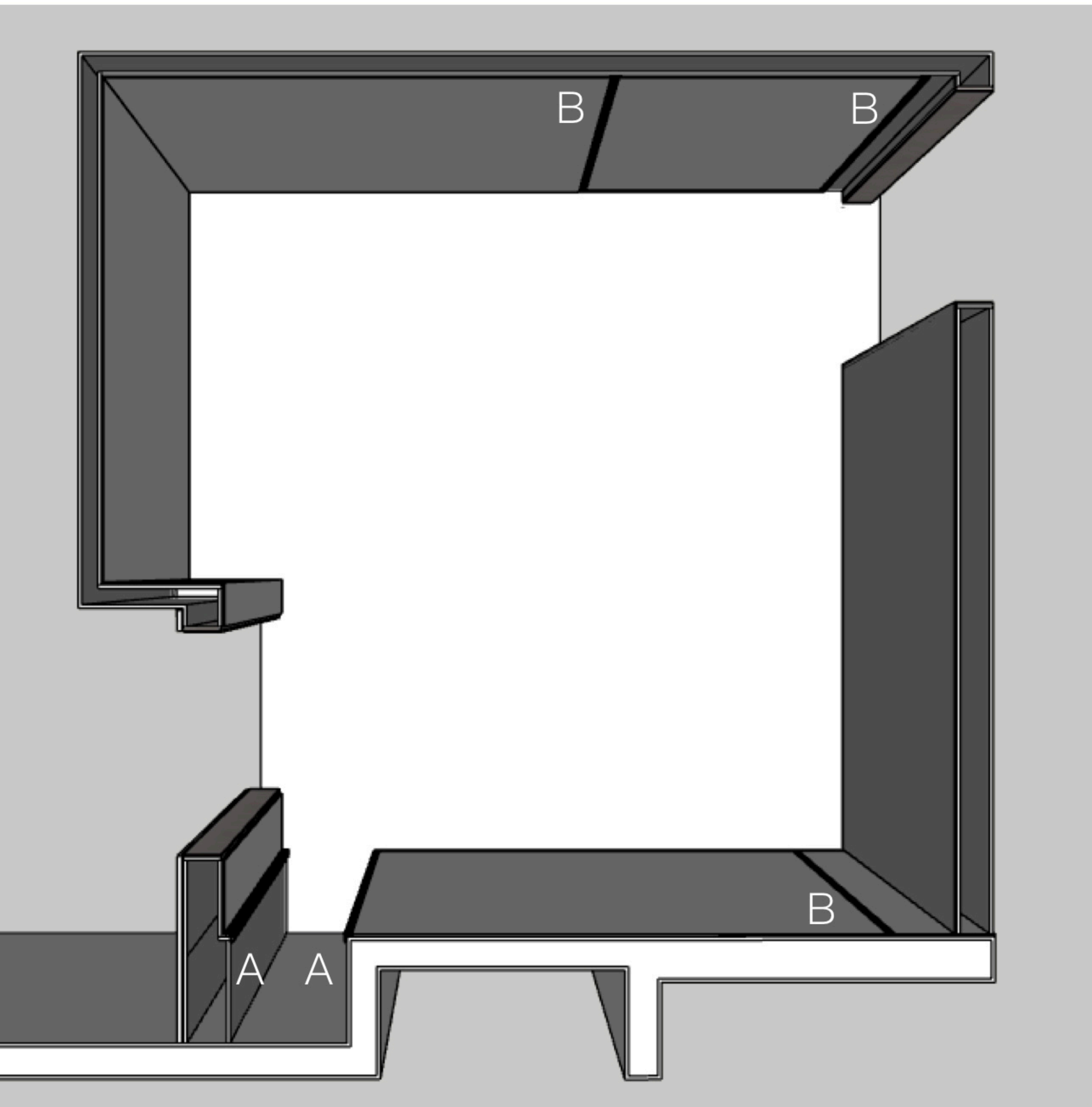
A处细节 15mm石膏板+面层 9mm硅酸钙板
