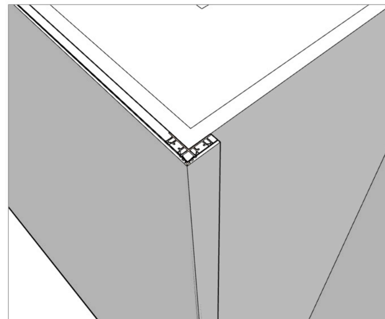
A处细节 15mm石膏板+面层 9mm硅酸钙板
