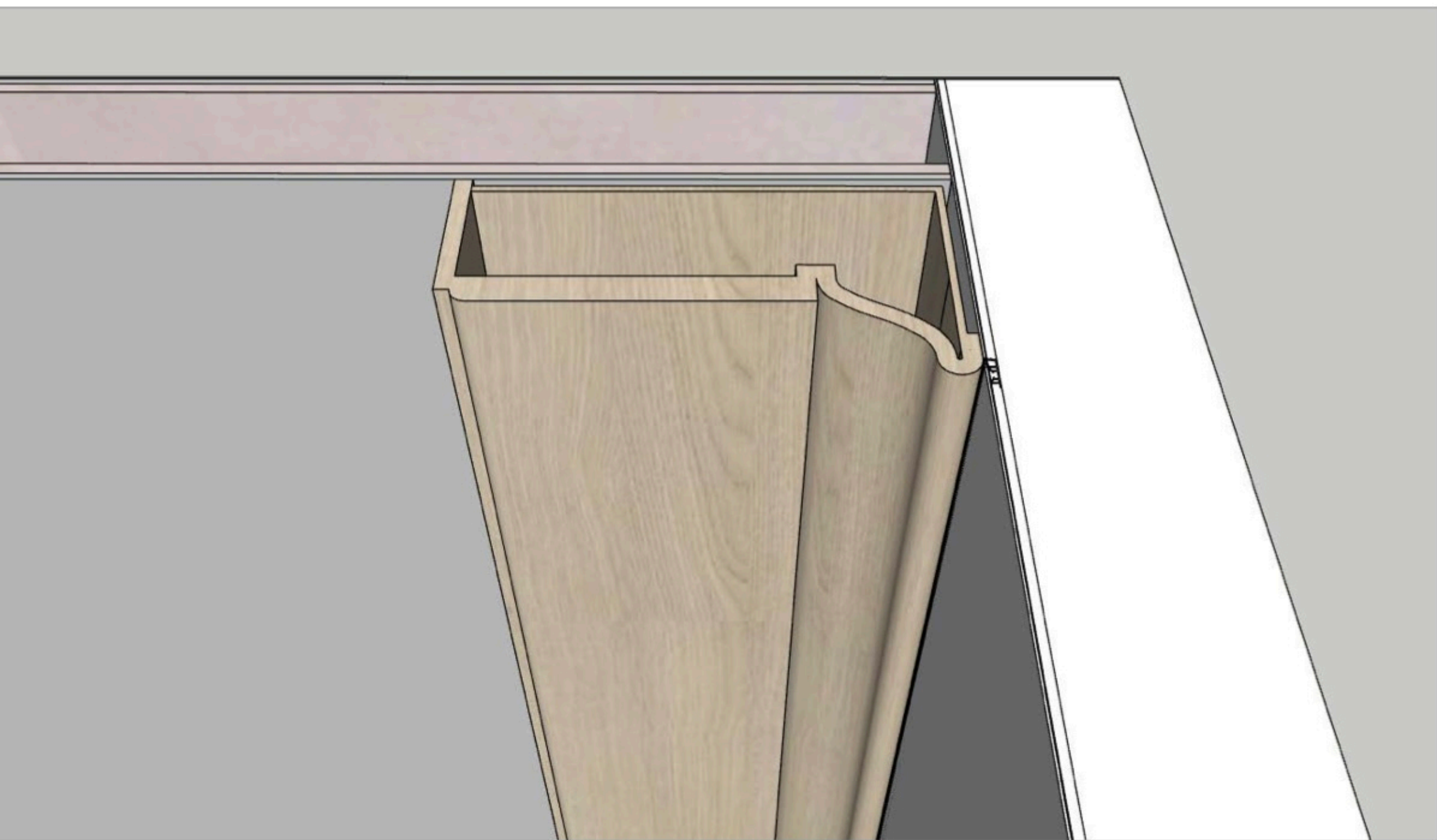
12 安装造型墙板
