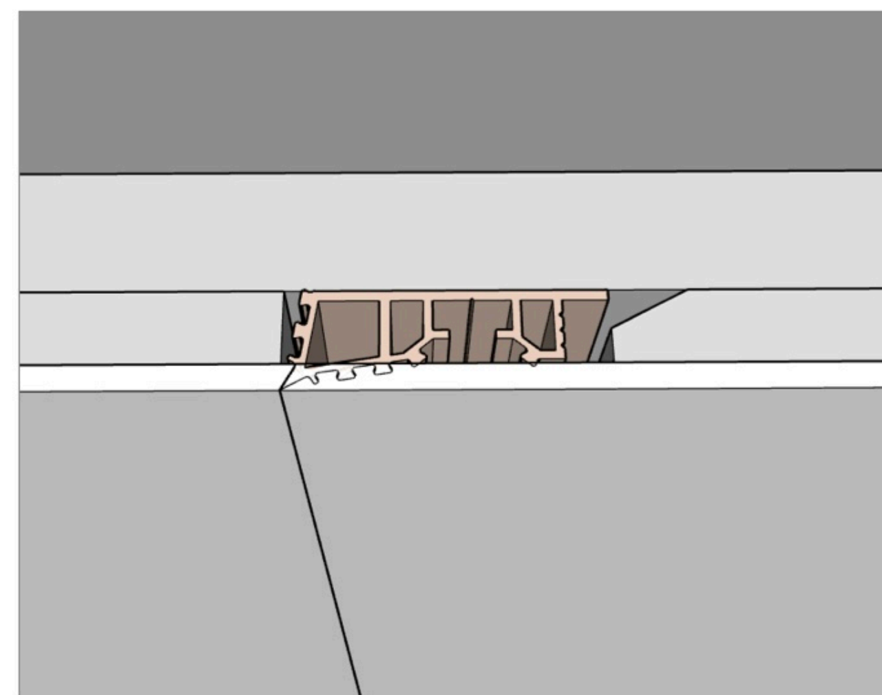
B处细节 15mm石膏板+面层 9mm硅酸钙板
