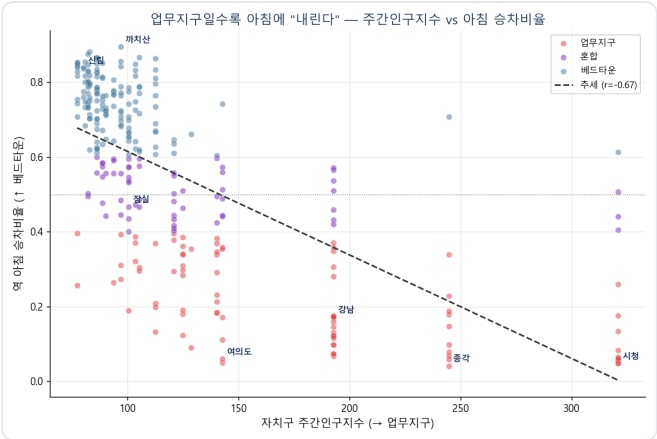
자치구 주간인구지수 vs 역 아침 승차비율
