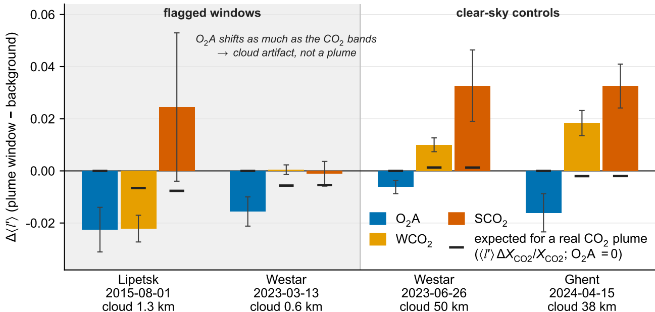
(d) band-resolved \langle I' \rangle fingerprint
