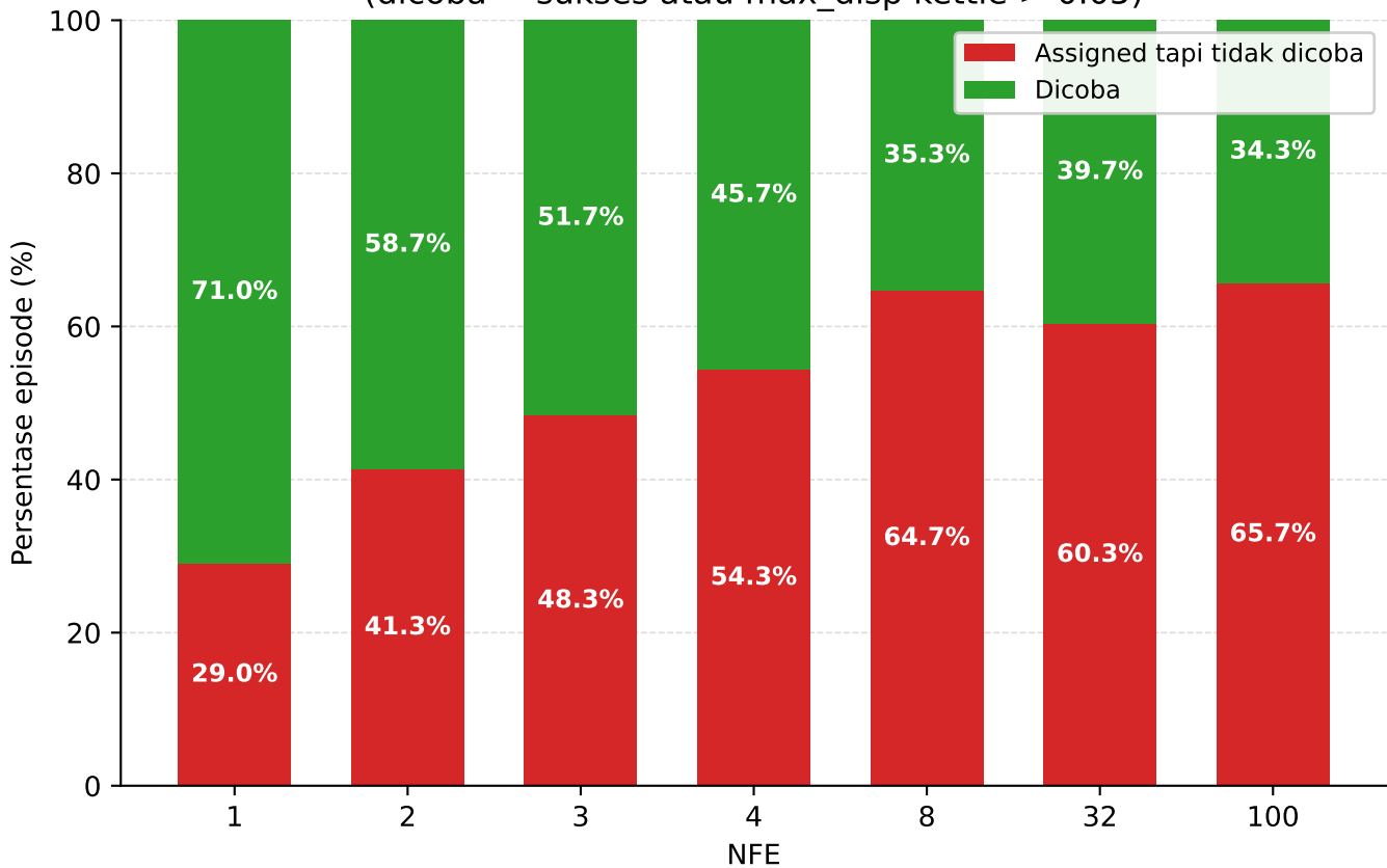
FlowPolicy: proporsi episode yang mencoba kettle vs NFE (dicoba = sukses atau max_disp kettle > 0.05)
