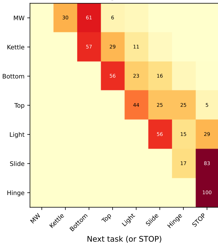
FP@NFE=10
