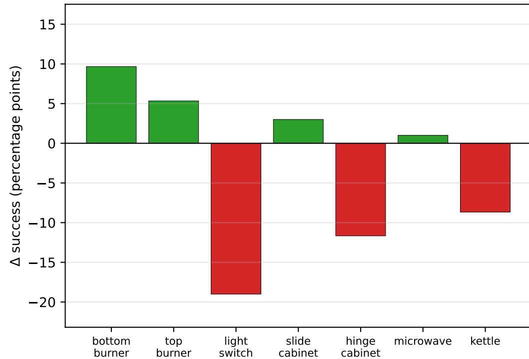
FP – CNN (pp) (all @NFE=100)
