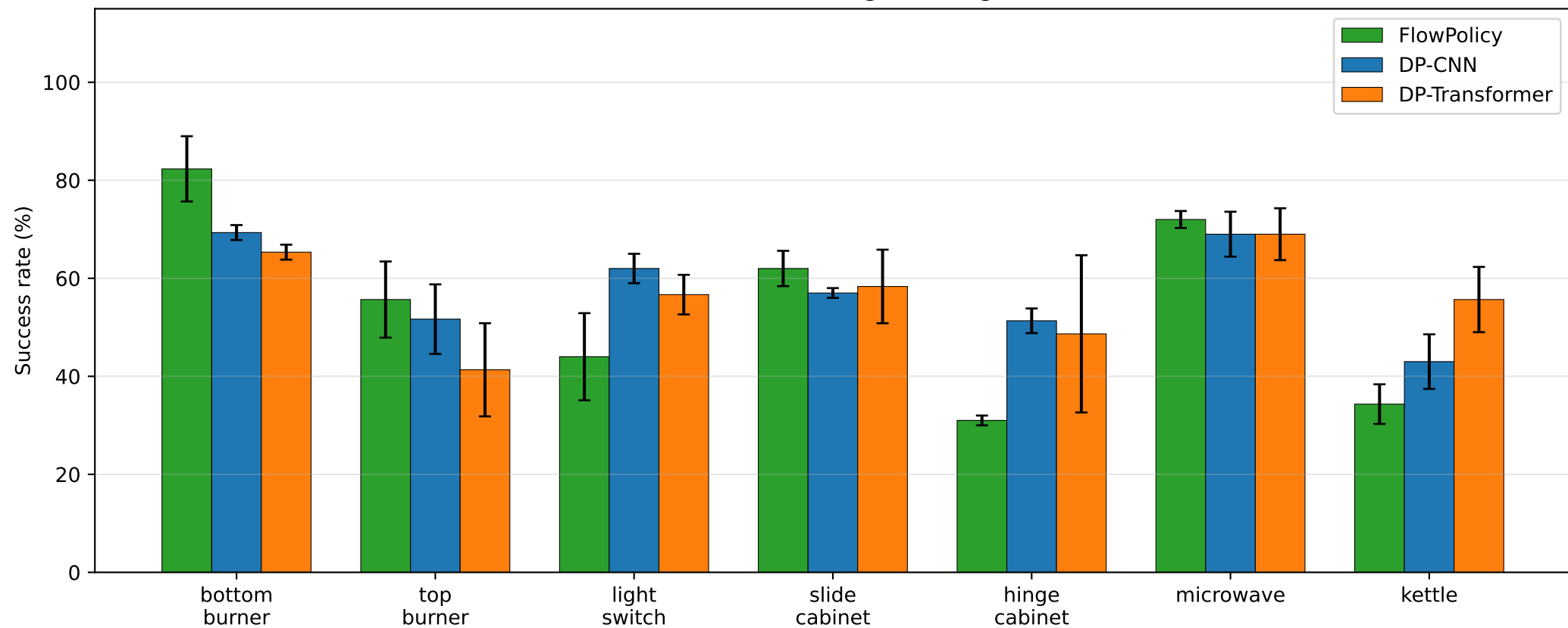
Per-task success (FP@8 vs DP@100)
