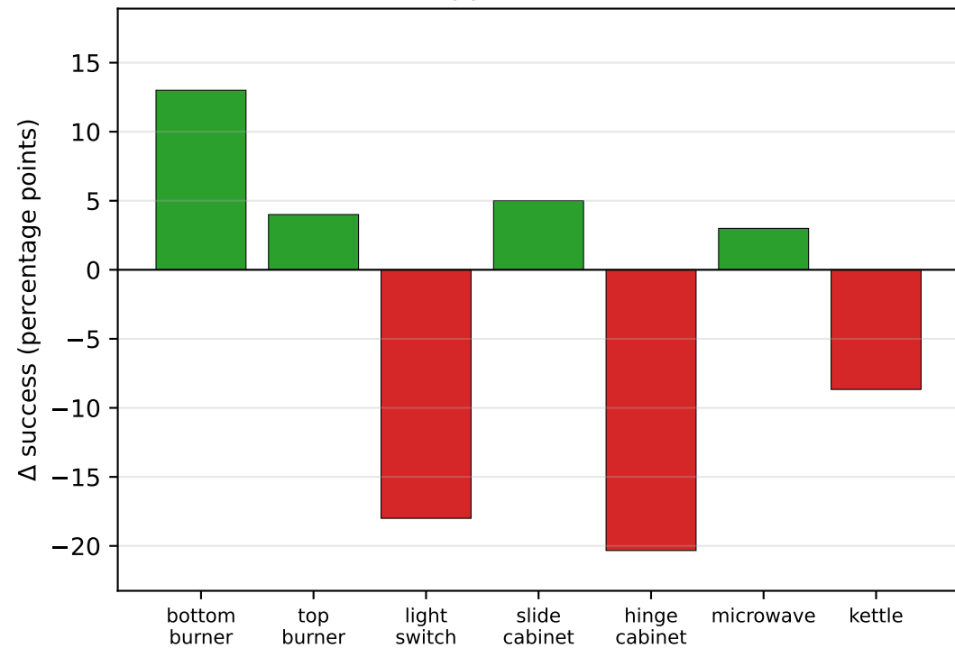
FP – CNN (pp) (FP@8 vs DP@100)
