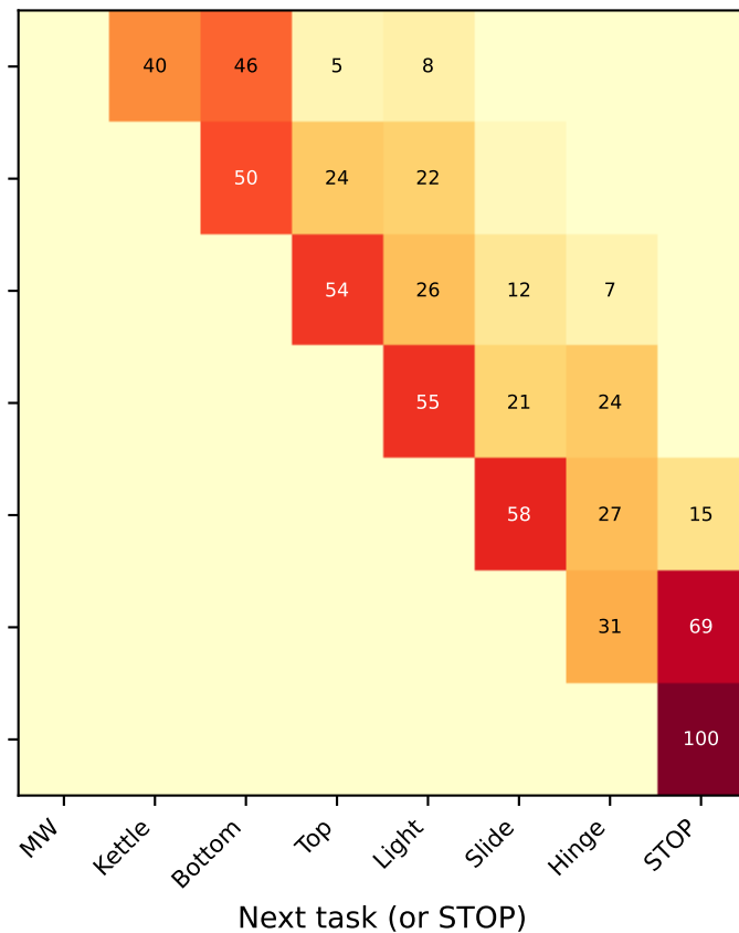
DP-CNN
