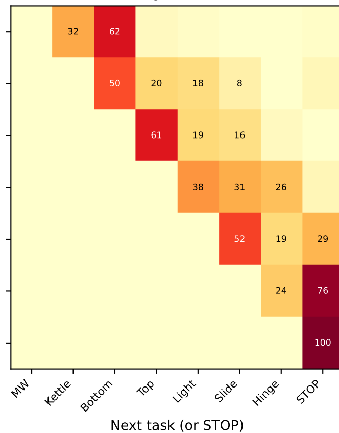
FP@NFE=32
