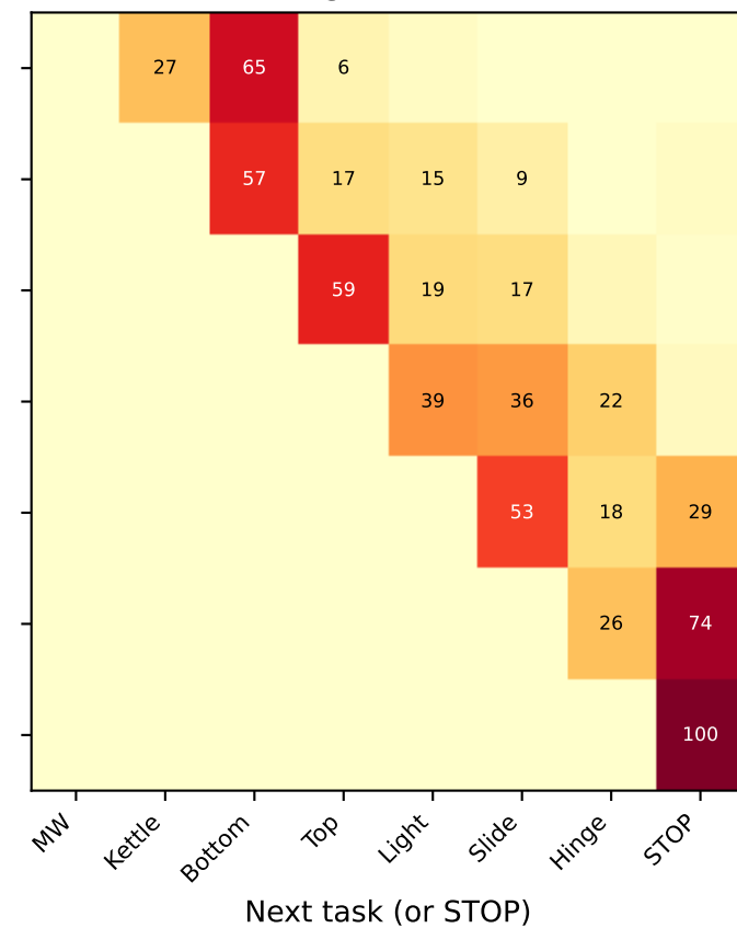
FP@NFE=100
