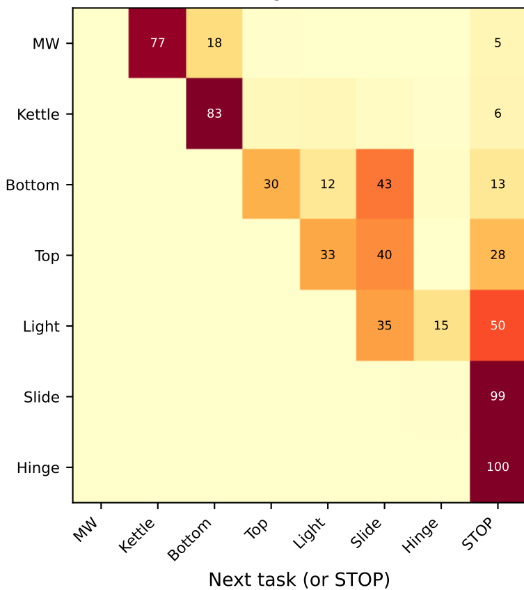
FP@NFE=1
