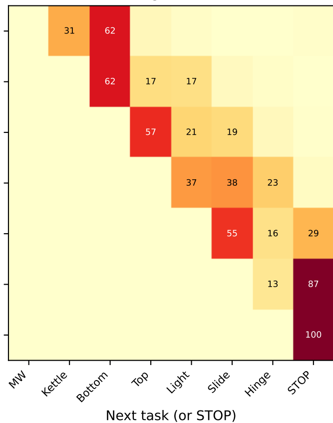
FP@NFE=8
