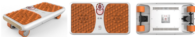
图5 第六代固柢太极车外观形状（立体图、俯视图、仰视图）
