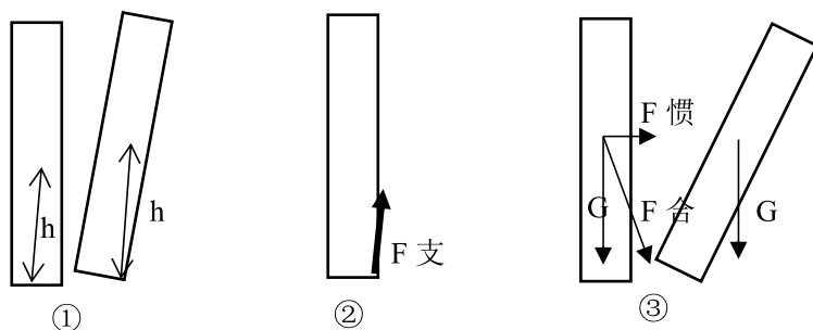
图 13 固抵力学分析示意图
