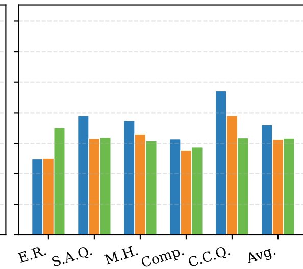
Qwen3-vl-8B
