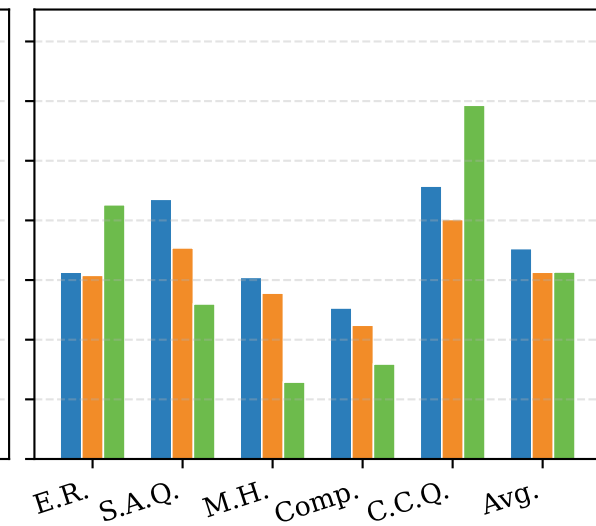
Qwen3-vl-32B
