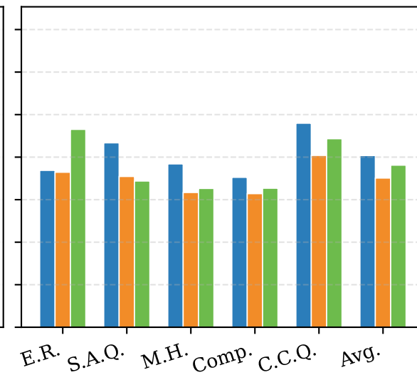
Qwen3-vl-4B
