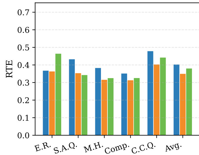
Qwen3-vl-4B
