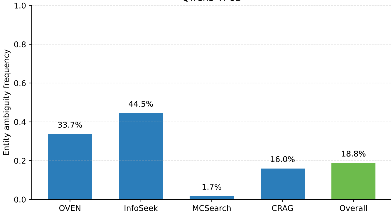
Qwen3-vl-8B
