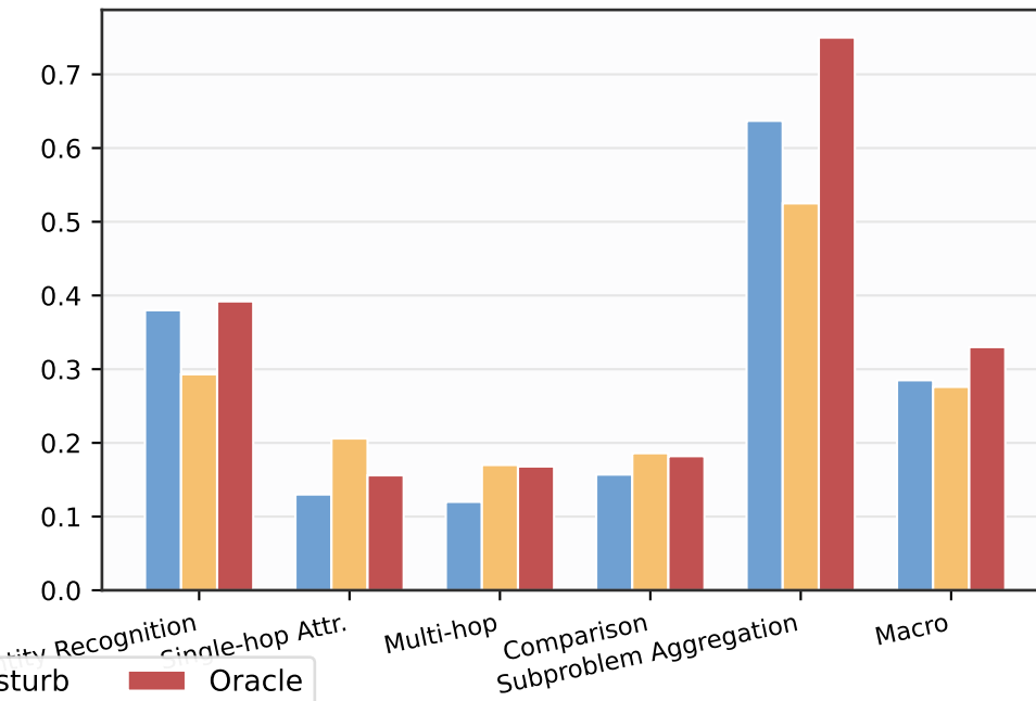
LJ score
