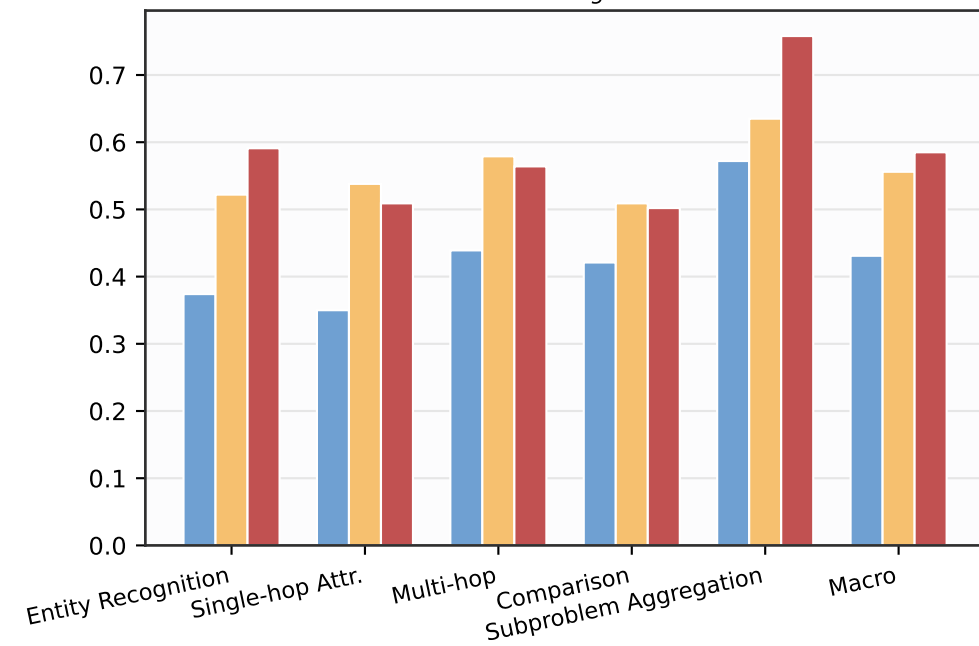
LJ score
