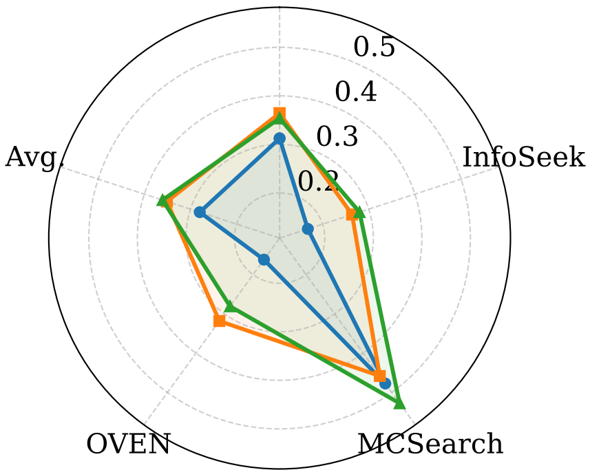
RTE CRAG-MM
