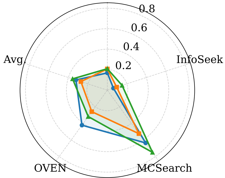
LJ score CRAG-MM
